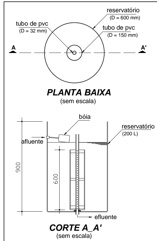
Figura 4.10 – Reservatório de 200L utilizado para instalação da coluna de 0,60m de altura (medidas em milímetros).
