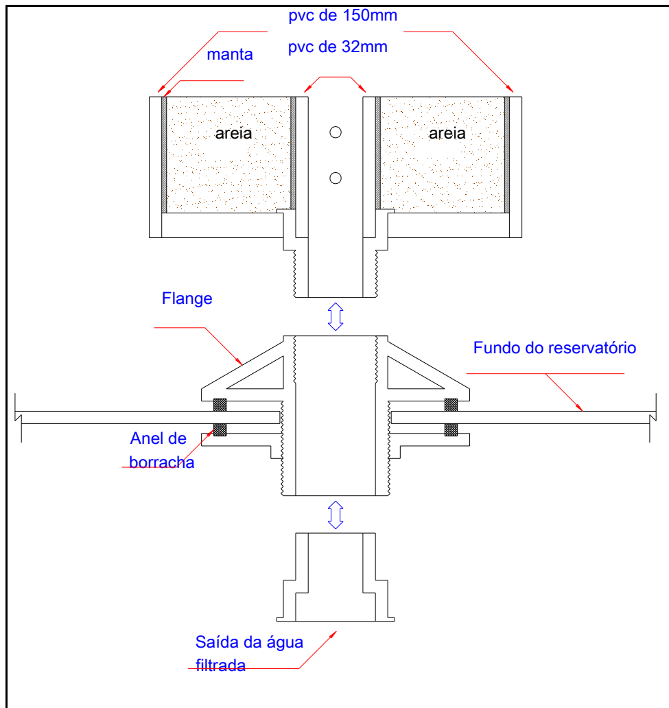
Figura 4.11 – Detalhamento do engate roscável das colunas verticais de filtração.
