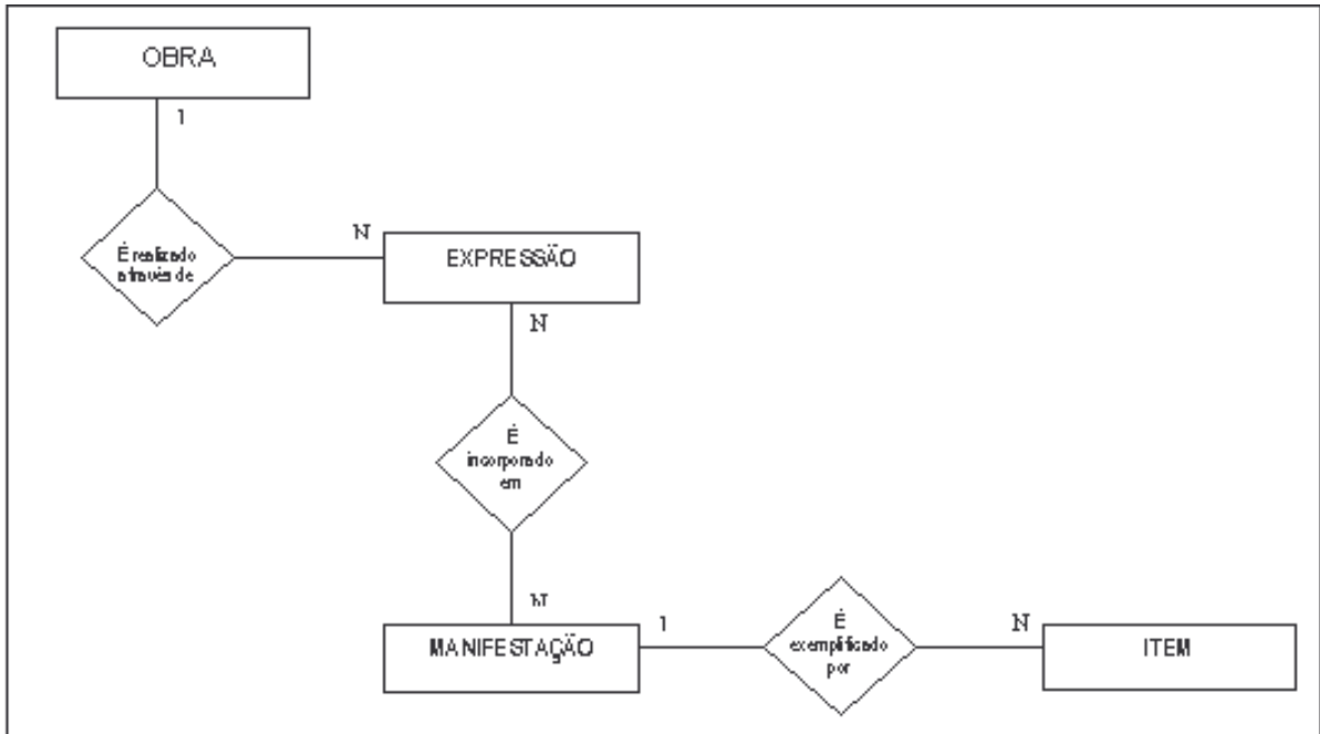
FIGURA 9 – Diagramação original do MER - Exemplo
