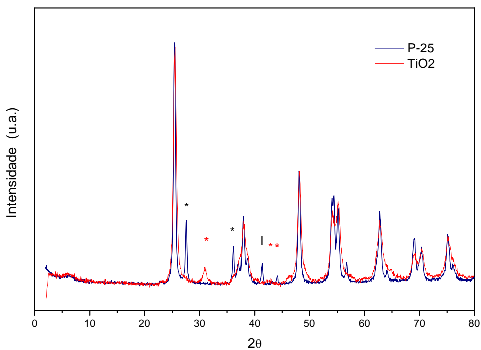
Figura 4.1. Difractogramas de Raios-X dos fotocatalisadores a) 10% ZnO/TiO 2 , TiO 2 e ZnO b) TiO 2 e P25-Degussa.
