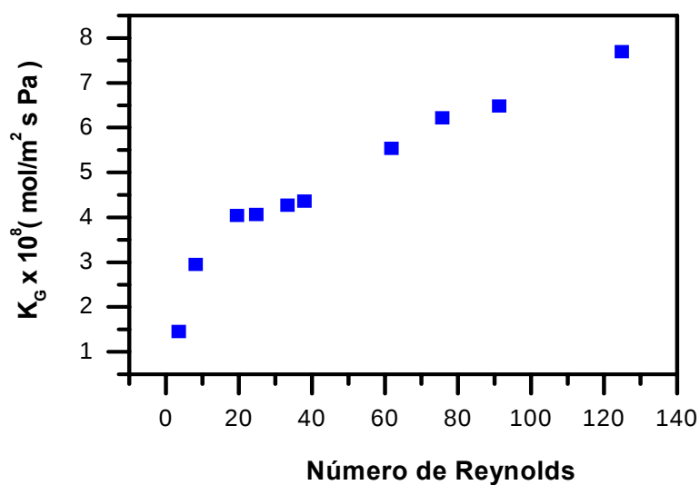
Figura 4.3 - Variação do coeficiente global de transferência de massa em função do número de Reynolds, com alimentação do módulo sendo feita pelo casco, com composição média de 10,5 %.
