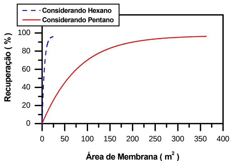
Figura 4.31 - Simulação da variação da recuperação de hexano e de pentano com o aumento da área de permeação para a membrana com espessura de 400 \mu\text{m} . Condições de operação: Vazão= 40 \text{m}^3/\text{h} , Concentração= 20% molar, \text{Re}= 200 (Hexano), 107 (Pentano), Pressões: alimentação (manométrica) = 0,5 atm,(Hexano), 0,8 atm (Pentano), permeado= 1 cmHg
