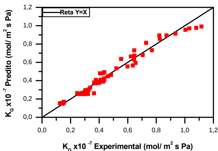
Figura 4.19 Comparação entre os dados experimentais de K_G e aqueles estimados pelo modelo de resistência em série modificado (Equação 4.1).
