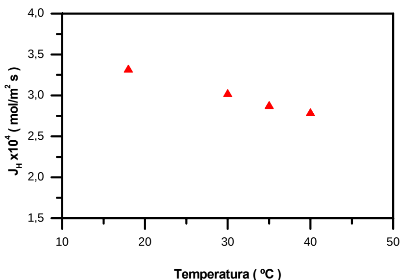
Figura 4.13 - Variação do fluxo de permeado com a temperatura de operação.
