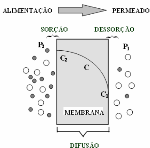
Figura 2.3 - Mecanismo sorção e difusão (HABERT et al , 2006).
