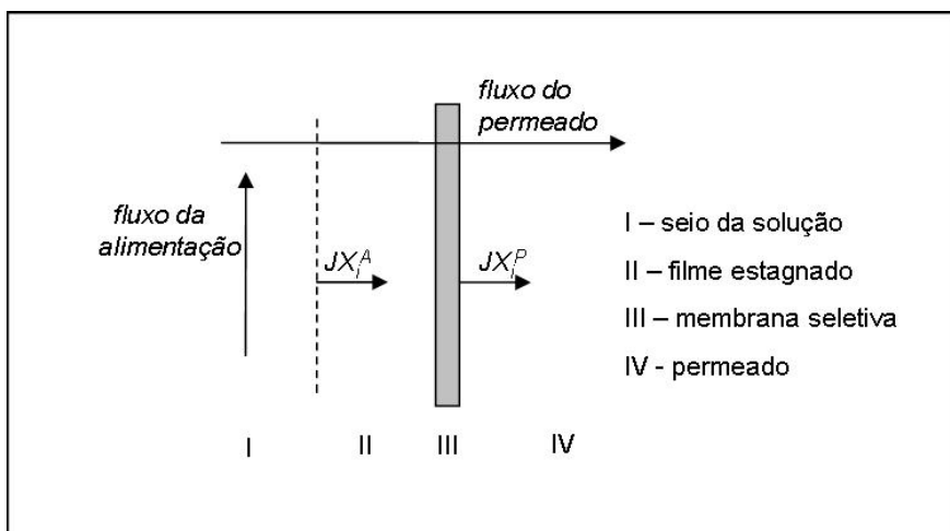
Figura 2.5 - Representação esquemática do filme estagnado adjacente à superfície da membrana (WIJMANS et al , 1996 ).
