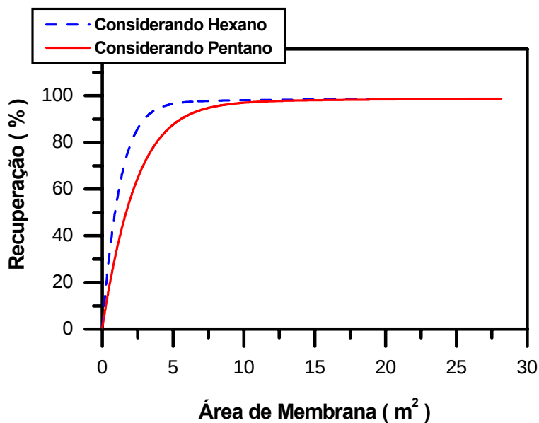
Figura: 4.22 Simulação da variação da recuperação de hexano e de pentano com o aumento da área de permeação para a membrana com espessura de 10 \mu\text{m} . Condições de operação: Vazão= 40 \text{m}^3/\text{h} , Concentração= 20% molar, \text{Re}= 200 (Hexano), 200 (Pentano), Pressões: alimentação (manométrica) = 0,5 atm,(Hexano), 0,5 atm (Pentano), permeado= 1 cmHg
