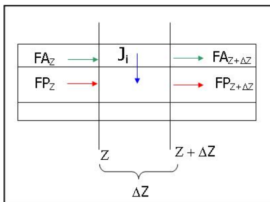
Figura 2.9 - Balanço de massa diferencial no módulo de fibra oca em configuração co-corrente.
