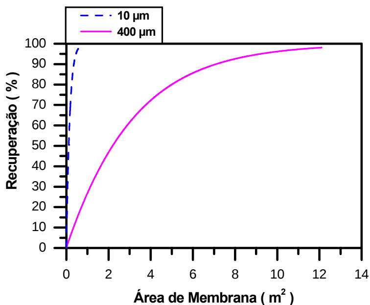
Figura 4.27 - Simulação da variação da recuperação de hexano com o aumento da área de permeação, utilizado membranas com diferentes espessuras (400 e 10 \mu\text{m} ). Condições de operação: Vazão= 10 m³/h, Concentração= 15% molar, Re= 200, Pressões: alimentação= 1 atm permeado= 0 cmHg
