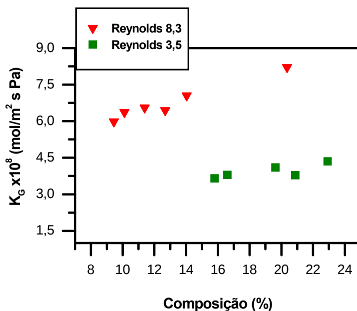
Figura 4.8 - Variação do coeficiente global de transferência de massa em função da composição de hexano na alimentação do módulo, feita por dentro das fibras.
