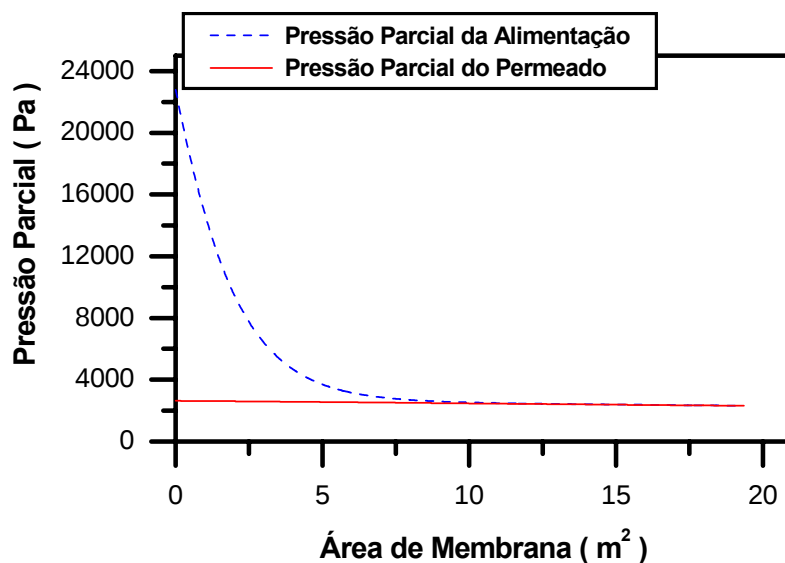
Figura 4.25 - Simulação da variação na pressão parcial de hexano na alimentação e no permeado com o aumento da área de membrana. Condições de operação: Vazão= 5m 3 /h, Concentração= 15% molar, Re= 100, Pressões: alimentação= 0,5 atm permeado= 2 cmHg.
