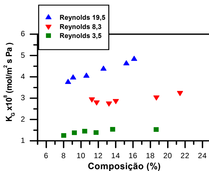
Figura 4.7 - Variação do coeficiente global de transferência de massa em função da composição de hexano na alimentação do módulo, feita pelo casco.
