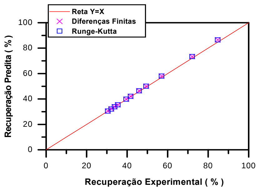
Figura 4.17 - Comparação dos dados experimentais e calculados para a recuperação de hexano com a alimentação ocorrendo por dentro das fibras.
