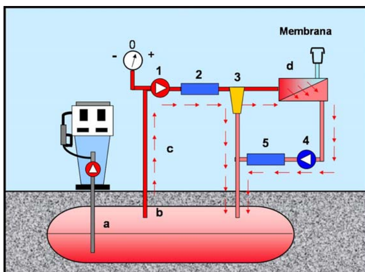
Figura 4.30 - URV para postos de serviços: 1 compressor, 2 trocador de calor, 3 separador líquido-gás, 4 bomba de vácuo, 5 condensador.
