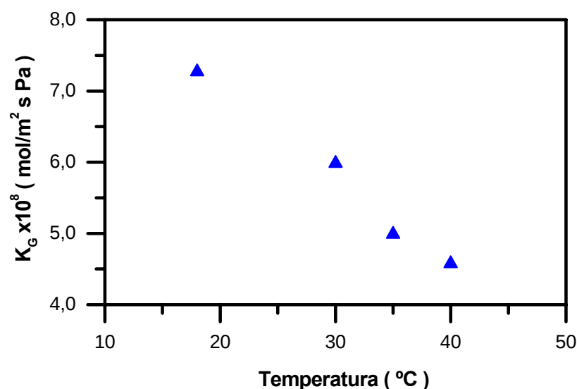
Figura 4.14 - Variação do coeficiente global de transferência de massa com a temperatura de operação.
