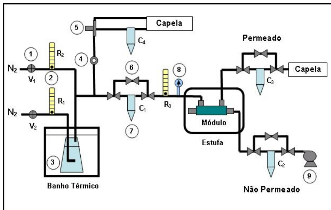
Figura 3.2 - Esquema simplificado do sistema de permeação de vapor: 1 Válvula controladora de pressão, 2 Rotômetro, 3 Frasco lavador de gás, 4 Válvula agulha, 5 Válvula de três vias, 6 Válvula esfera, 7 Cristalizador, 8 Manômetro, 9 Bomba de vácuo.
