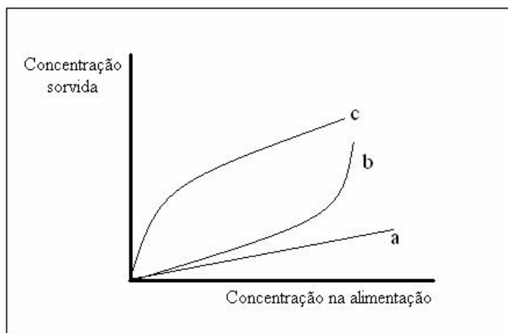
Figura 2.4 - Tipos de isothermas de sorção em membranas poliméricas: (a) ideal; (b) com inchamento; (c) modelo dupla sorção.
