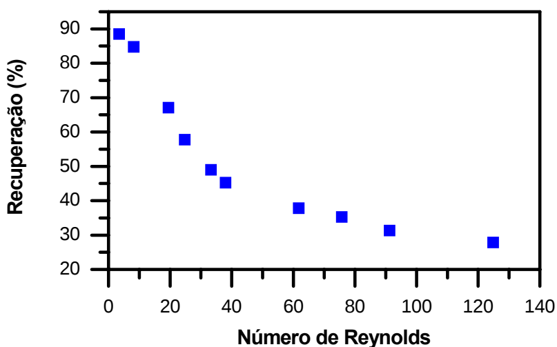
Figura 4.1 - Variação da recuperação de hexano em função do número de Reynolds, com alimentação do módulo sendo feita pela carcaça, com composição média de 10,5 %.
