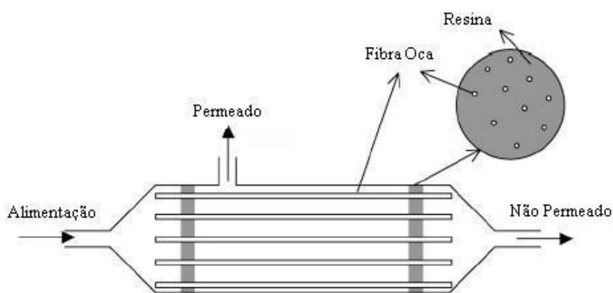
Figura 3.1 - Esquema de confeccção dos módulos de permeação.
