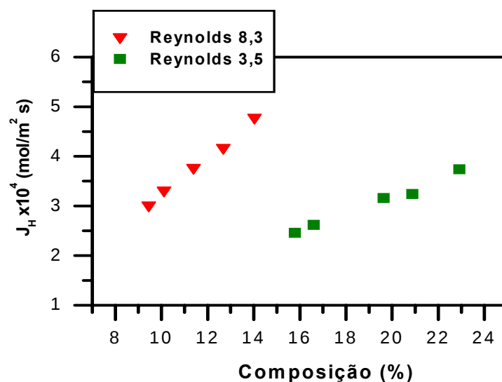
Figura 4.6 - Variação do fluxo de permeado com a composição de hexano na alimentação do módulo feita por dentro das fibras.
