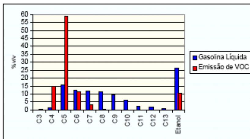
Figura 4.16 Perfil de composição da emissão de VOC e da gasolina líquida (SOUZA, 2004).
