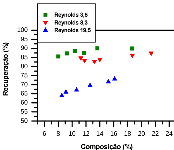
Figura 4.9 - Variação da recuperação de hexano em função da composição de alimentação do módulo, sendo feita pela carcaça.
