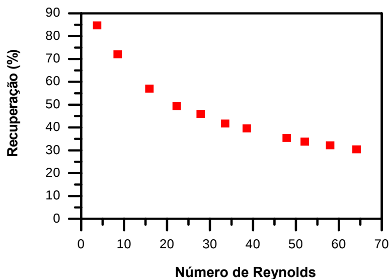
Figura 4.2 - Variação da recuperação de hexano em função do número de Reynolds, com alimentação do módulo sendo feita por dentro das fibras, com composição média de 8,0 %.
