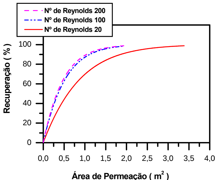
Figura 4.20 - Simulação da recuperação de hexano com o aumento da área de permeação, em diferentes números de Reynolds. Alimentação por dentro das fibras nas seguintes condições: Vazão = 2 m³/h, Concentração = 15% molar, Pressão = 1 atm.
