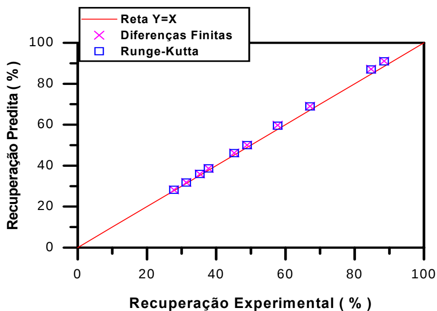
Figura 4.18 - Comparação dos dados experimentais e calculados para a recuperação de hexano com a alimentação ocorrendo pelo casco.
