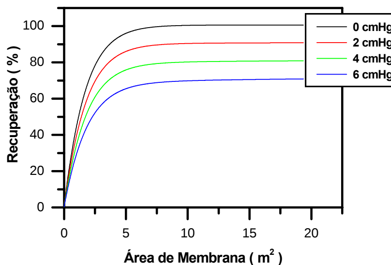
Figura 4.24 - Simulação da recuperação de hexano com o aumento da área de membrana, utilizando diferentes pressões no lado permeado. Alimentação: Vazão = 5m³/h, Concentração = 15% molar, Pressão da alimentação = 0,5 atm, Re = 100
