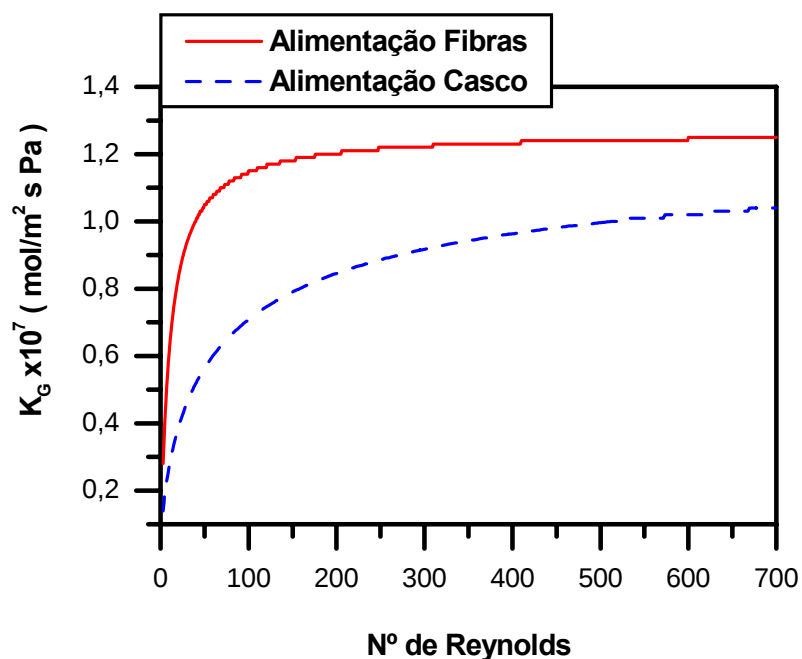
Figura 4.21 - Simulação da coeficiente global de transferência de massa para o hexano com o aumento do números de Reynolds, para alimentação por dentro das fibras e pelo casco.
