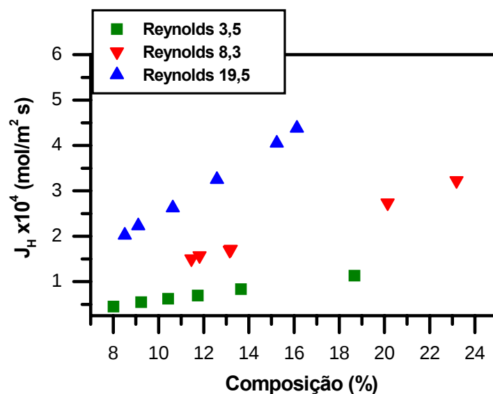
Figura 4.5 - Variação do fluxo de permeado com a composição de hexano na alimentação do módulo feita pelo casco.
