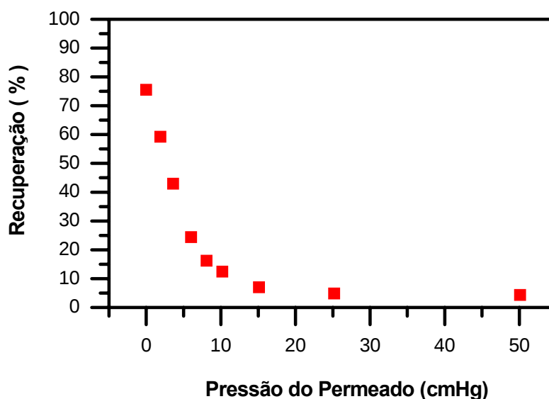
Figura 4.12 - Variação da recuperação de hexano em função da pressão do permeado.
