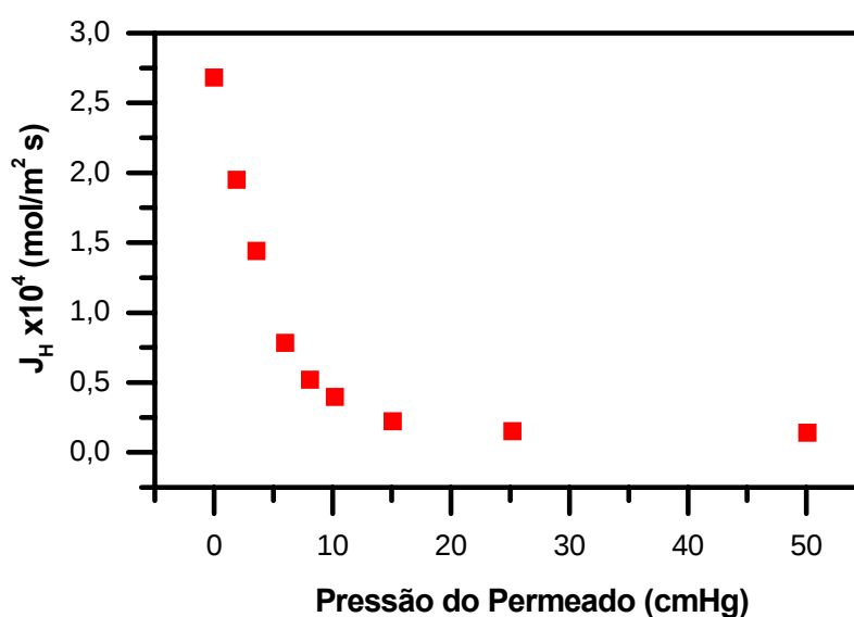
Figura 4.11 - Variação do fluxo permeado em função da pressão do permeado.
