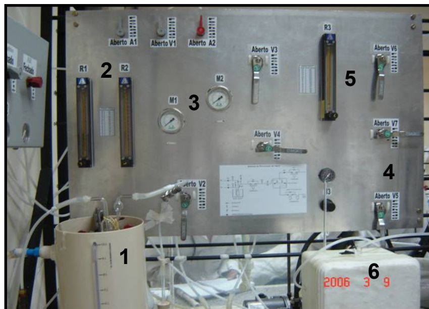
Figura 3.3 - Fotografia do sistema de permeação de vapor: 1 Banho térmico, 2 Rotômetros de admissão de nitrogênio, 3 Manômetros, 4 Válvulas esfera, 5 Rotâmetro de controle de vazão de alimentação, 6 Estufa com o módulo de membranas.
