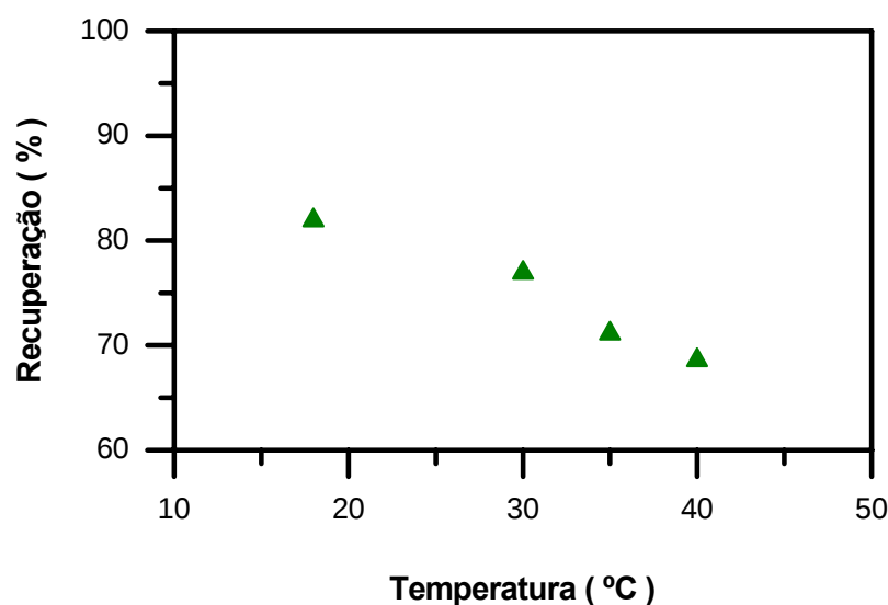
Figura 4.15 - Variação da recuperação de hexano em função da temperatura de operação.
