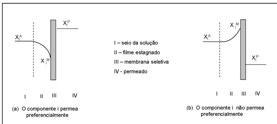
Figura 2.6 - Representação esquemática do fenômeno de polarização de concentração no filme estagnado adjacente à membrana (WIJMANS et al , 1996).
