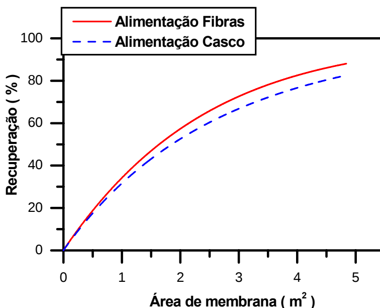
Figura 4.22 - Simulação da recuperação de hexano com o aumento do comprimento do módulo, utilizando diferentes modos de alimentação. Alimentação nas seguintes condições: Vazão = 10 \text{ m}^3/\text{h} , Concentração = 15% molar, Pressões: Alimentação = 1 atm Permeado=0 cmHg
