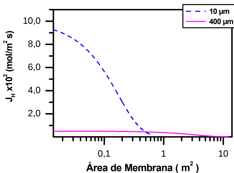
Figura 4.26 - 16 Simulação da variação do fluxo permeado de hexano com o aumento da área de permeação, utilizando membranas com diferentes espessuras (400 e 10 \mu\text{m} ). Condições de operação: Vazão= 5 \text{m}^3/\text{h} , Concentração= 15% molar, Re= 100 , Pressões: alimentação= 1 atm permeado= 0 cmHg.
