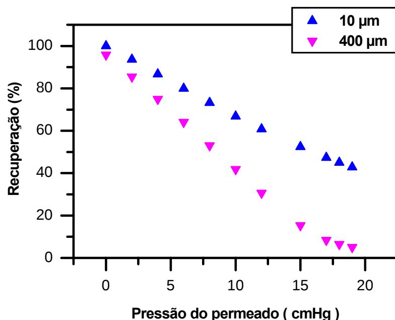
Figura 4.28 - Simulação da variação da recuperação de hexano com o aumento da pressão de permeado, utilizado membranas com diferentes espessuras (400 e 10 µm). Condições de operação: Vazão= 10 m 3 /h, Concentração= 15% molar, Re= 200, Pressões: alimentação= 0,5 atm, Ap=3,87 m 2
