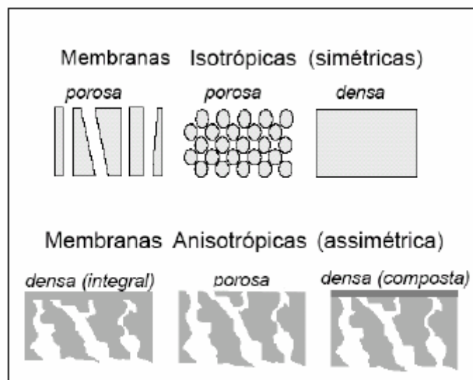
Figura 2.2 - Representação esquemática da seção transversal dos diferentes tipos de morfologia de membranas sintética (HABERT et al 2006).
