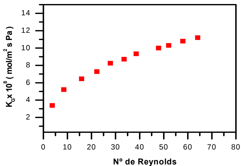
Figura 4.4 - Variação do coeficiente global de transferência de massa em função do número de Reynolds, com alimentação do módulo sendo feita por dentro das fibras, com composição média de 8,0 %
