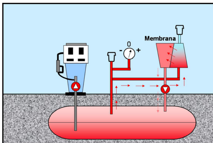
Figura 1.2 - Esquema simplificado de uma unidade de recuperação de COVs por permeação de vapor em postos de combustíveis.
