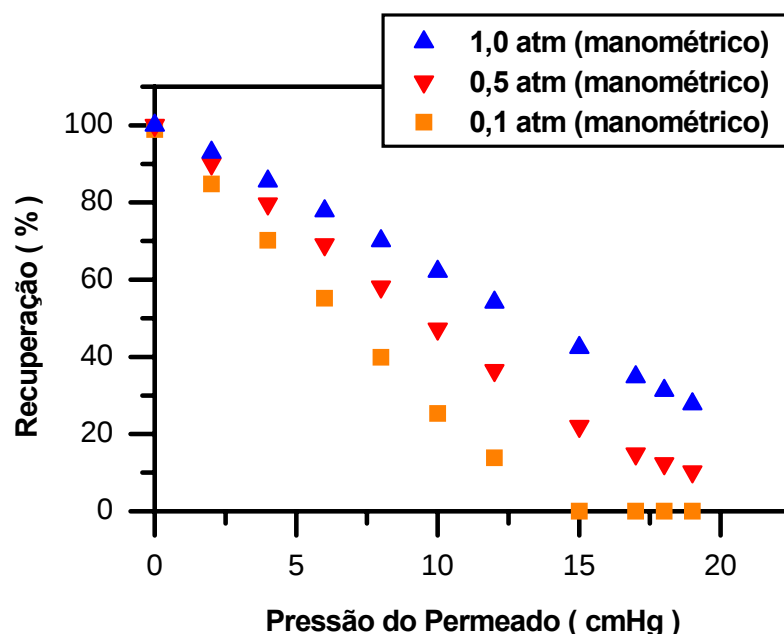
Figura 4.23 - Simulação da recuperação de hexano com o aumento da pressão do permeado, utilizando diferentes pressões para a alimentação. Alimentação nas seguintes condições: Vazão = 5 m 3 /h, Concentração = 15% molar, Re = 100, Ap= 4,35 m 2
