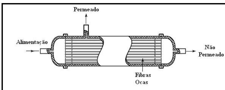
Figura 2.7 – Esquema simplificado do módulo de membranas de fibras ocas (BAKER, 2004.).
