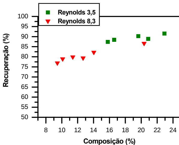
Figura 4.10 - Variação da recuperação de hexano em função da composição de alimentação do módulo, sendo feita por dentro das fibras.
