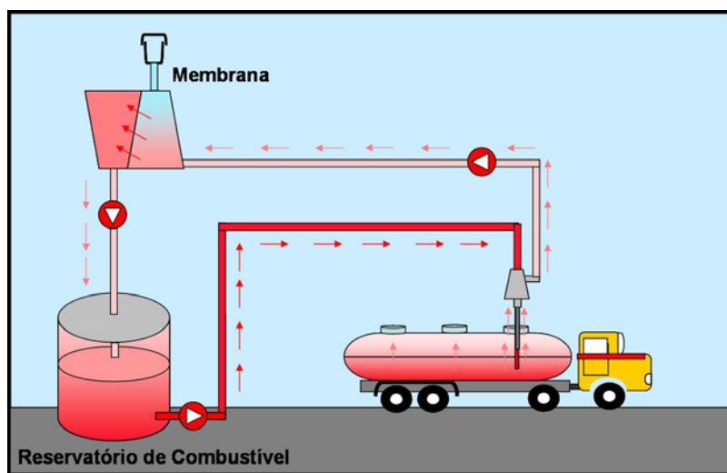
Figura 1.3 - Esquema simplificado do sistema de recuperação de COVs por permeação de vapor, instalados na base de carregamento.
