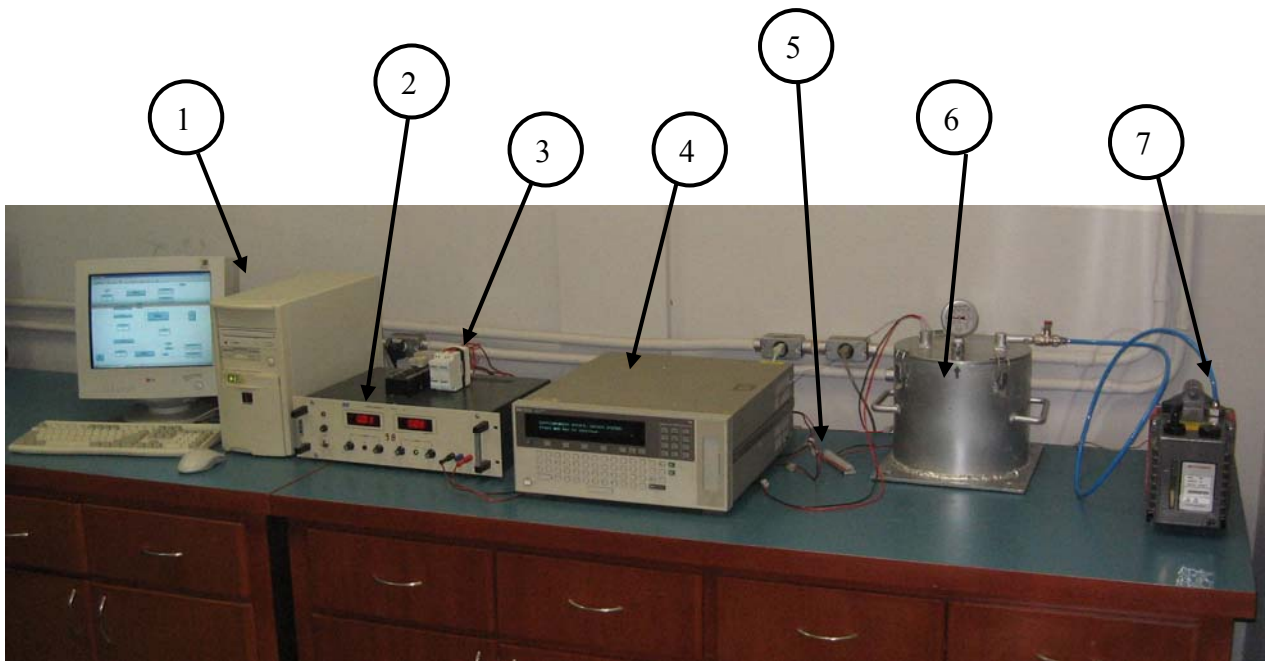
Figura 4.5 – Bancada Experimental
