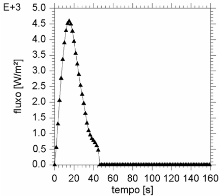
Figura 5.1 - Valores tıpicos de fluxo de calor.
