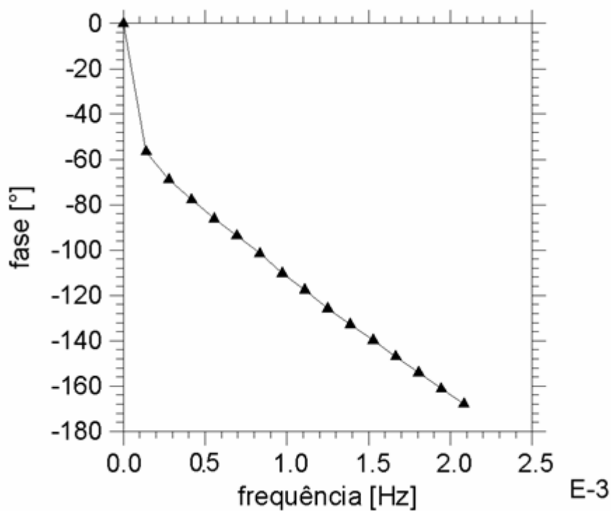
Figura 5.19 – Fase da função resposta em frequência H(f) .
