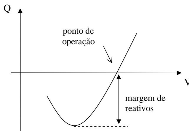
Figura 2.2 – Curva Q-V
