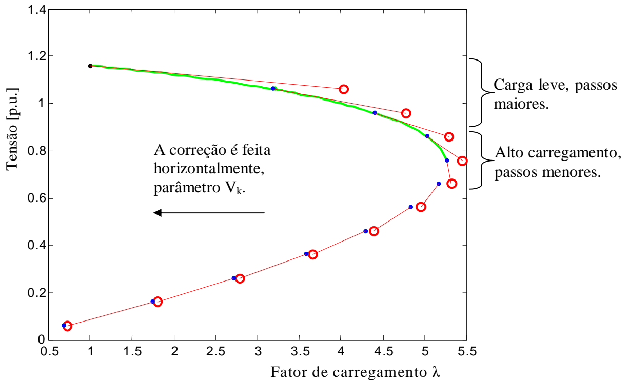
Figura 3.3: Controle automático do passo \sigma .
