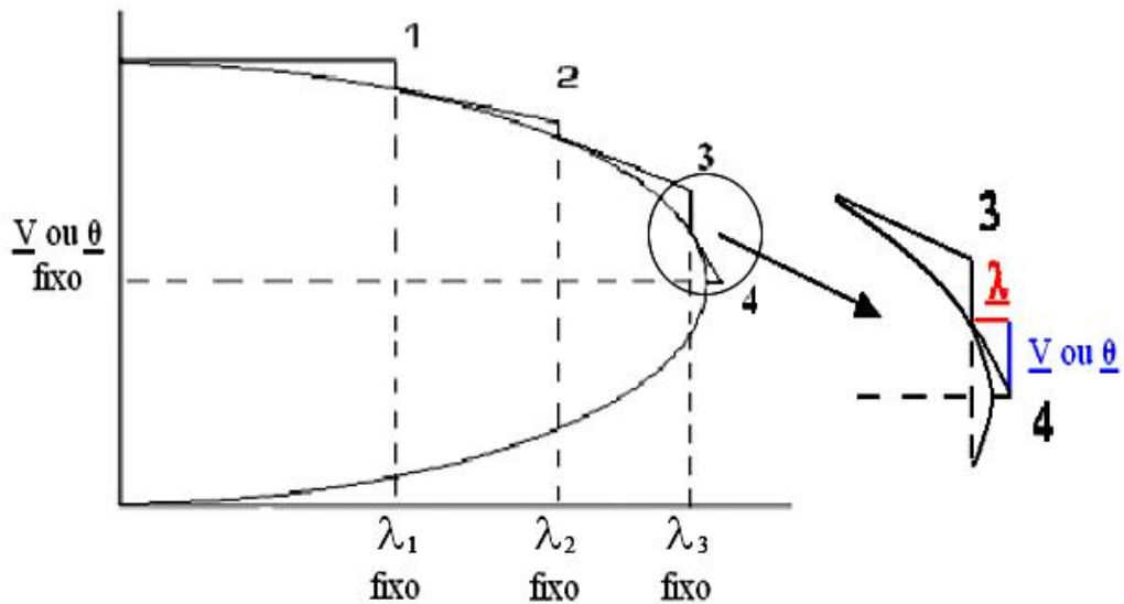
Figura 3.4: Técnica de Parametrização Local
