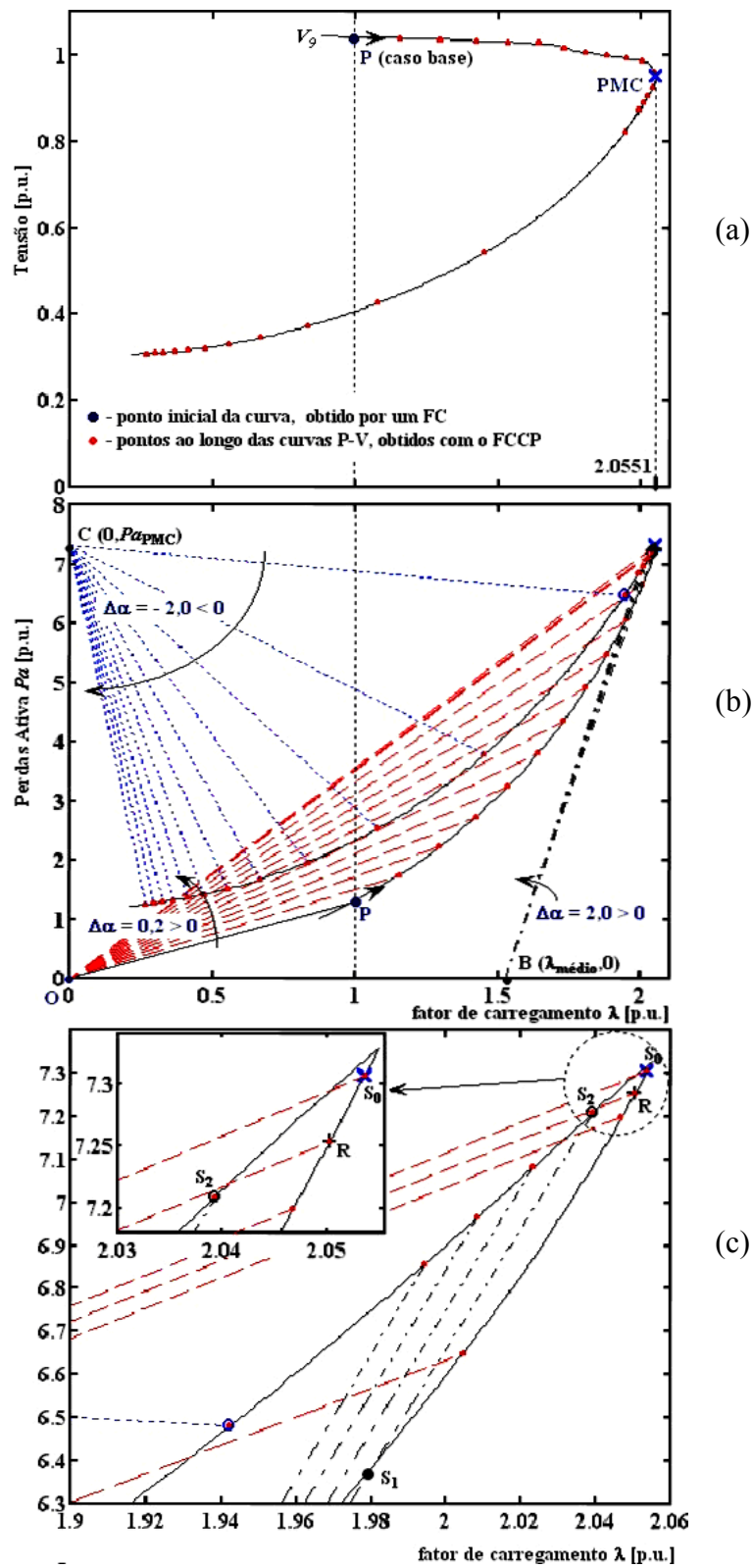
Figura 4.9: Desempenho do método proposto para o IEEE- 118, quadruplicando o passo inicial: (a) magnitude da tensão na barra crítica como função do carregamento, (b) P_a como função de \lambda , (c) detalhes do processo de convergência.
