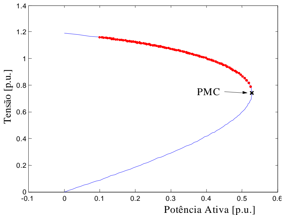
Figura 2.5: Curva P-V obtida através do método de FC (pontilhada), a partir do caso base ( \lambda=1 ).
