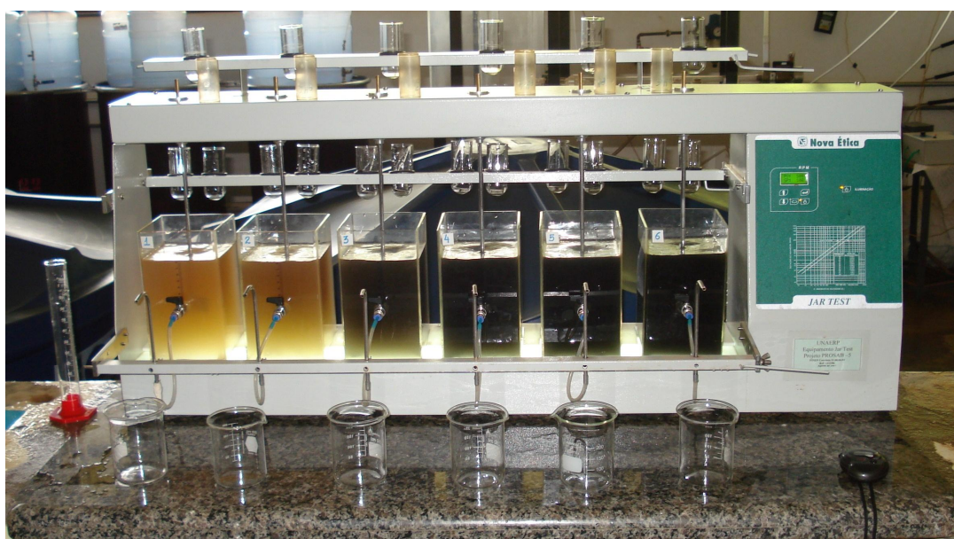
Figura 5.20: Foto de um ensaio de adsorção em CAP.
