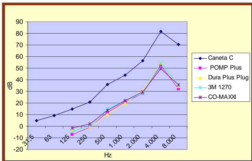
Figura 19 – Valores do ruído produzido pela caneta C de alta rotação expressos em decibels, nas 1/1 de bandas de oitavas
