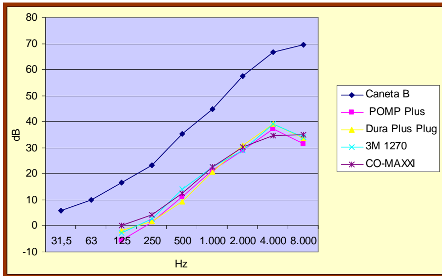
Figura 18 – Valores do ruído produzido pela caneta B de alta rotação expressos em decibels, nas 1/1 de bandas de oitavas (freqüências), expressas Hertz e as atenuações produzidas com as 4 marcas de protetores auditivos. Campinas, HC – Unicamp, 2005.
