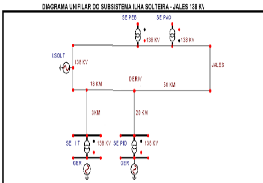
Figura 3.7: Diagrama Unifilar do Subsistema Ilha Solteira - Jales 138 kV.
