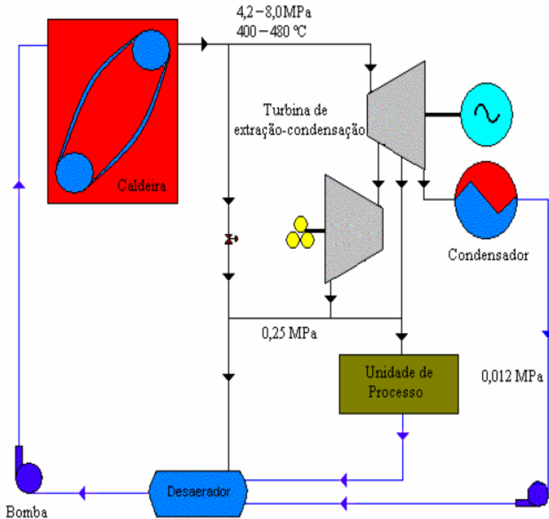
Figura 3.2: Diagrama de um sistema de cogeração a partir do uso de turbinas a vapor de extração-condensação (FIOMARI, 2004).
