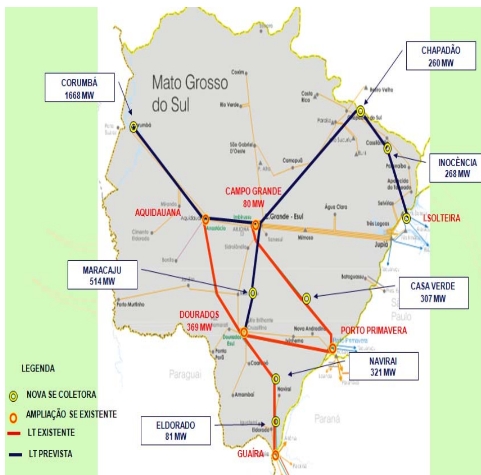
Figura 4.13: Sistema de transmissão do Mato Grosso do Sul, para o ano 2015.
