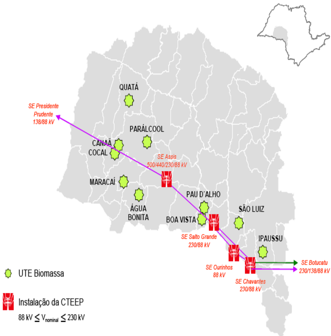
Figura 4.19: Usinas a biomassa e configuração das DIT na área IV (INTEGRAÇÃO, 2008).
