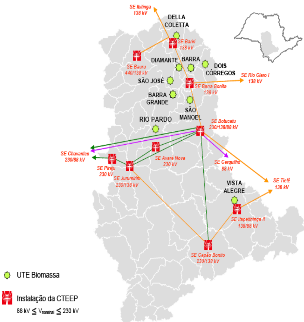
Figura 4.20: Usinas a biomassa e configuração das DIT na área V (INTEGRAÇÃO, 2008).
