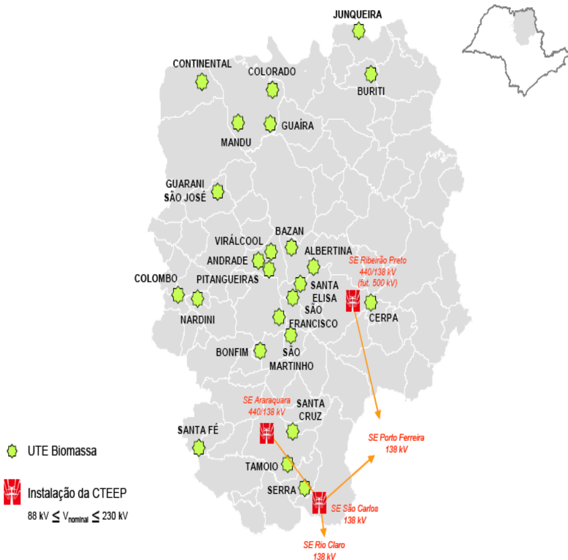
Figura 4.17 – Usinas a biomassa e configuração das DIT na área II (INTEGRAÇÃO, 2008).
