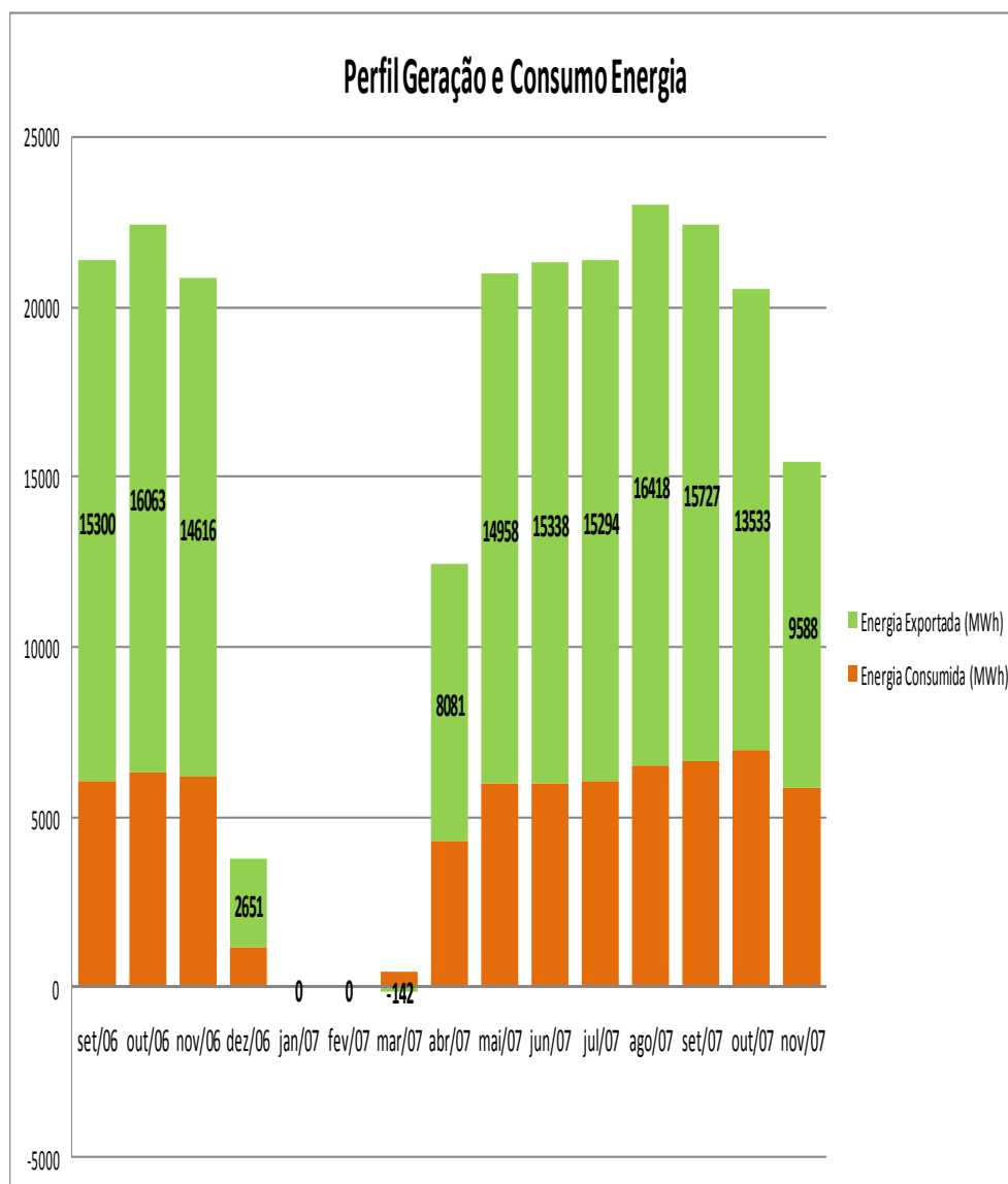
Figura 3.14: Perfil de geração e consumo da UTE.
