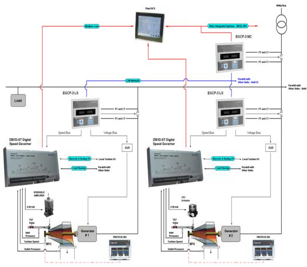
Figura 3.10: Sistema de controle dos turbogeradores da UTE.
