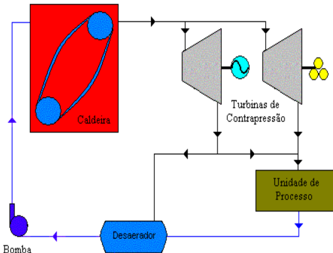
Figura 3.1: Diagrama de um sistema de cogeração a partir do uso de turbinas a vapor de contrapressão (FIOMARI, 2004)
