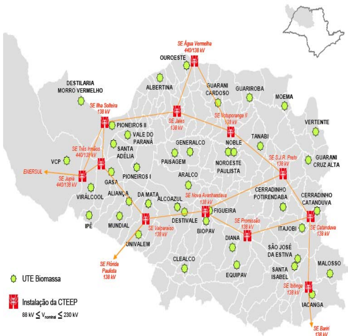
Figura 4.16 – Usinas a biomassa e configuração das DIT na área I (INTEGRAÇÃO, 2008).
