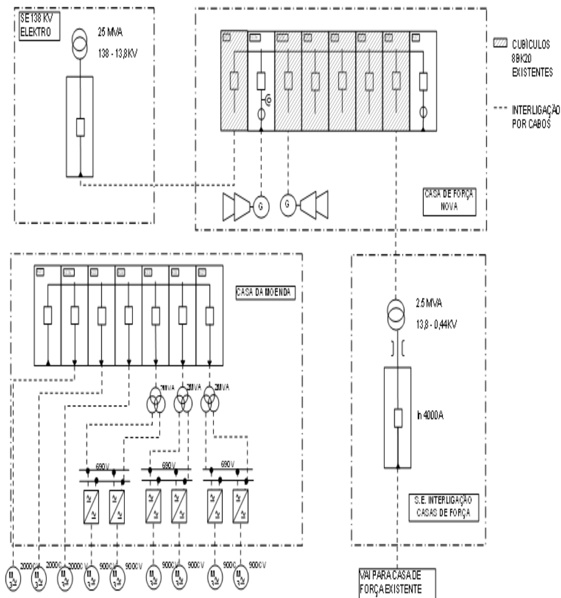
Figura 3.13: Diagrama unifilar simplificado da UTE.
