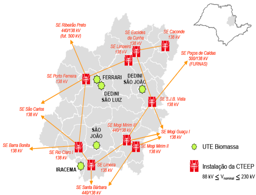
Figura 4.21 – Usinas a biomassa e configuração das DIT na área VI (INTEGRAÇÃO, 2008).
