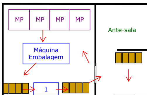
Figura 6.16 – Layout da linha de produção celular de embalagem do produto Isolador de Pressão – Vida Tecnologia Biomédica (2007)
