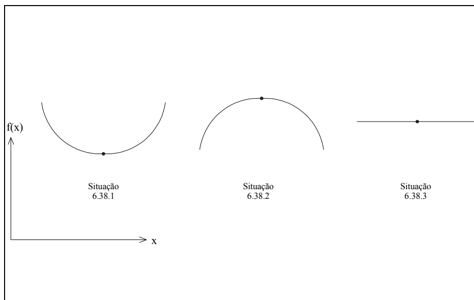
Figura 6.3 - Segunda Derivada de f(x)
