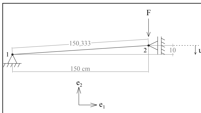
Figura 8.1 - Treça Plana Elástica Abatida
