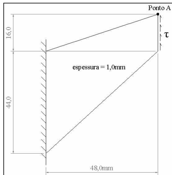
Figura 8.25 - Membrana de Cook
