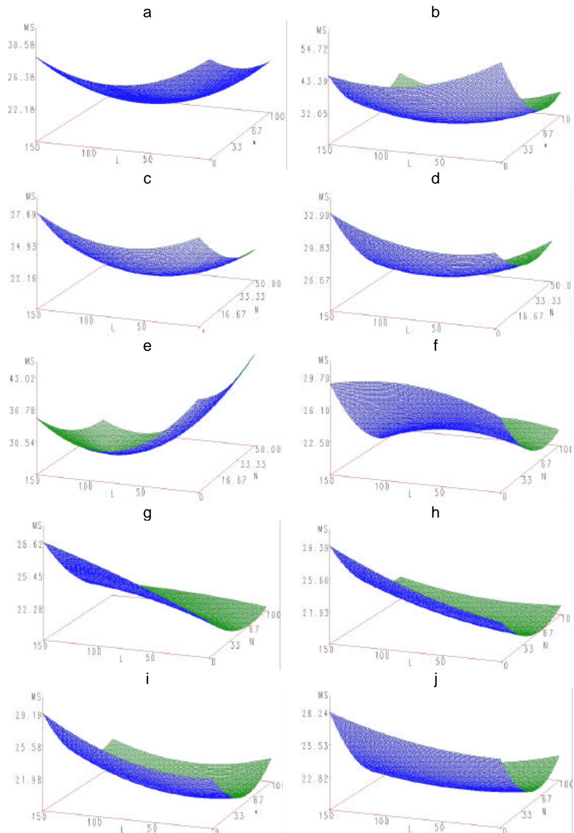
Figura 20. Superfícies de resposta para teores de MS, por época de corte.
