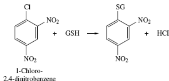
FIGURA 11 - Reação de conjugação da glutathione reduzida com o CNDB realizada pela enzima glutathione - S - transferase (HODGSON, 2004).
