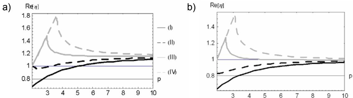
Figura 3.2 – Valor real de \eta em função de p com \xi=0.2 para a integração de Newmark com a) \beta=1/4 e b) \beta=1/12 .
