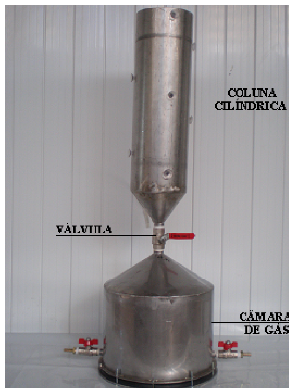
Figura 6 – Protótipo do mecanismo de difusão.
