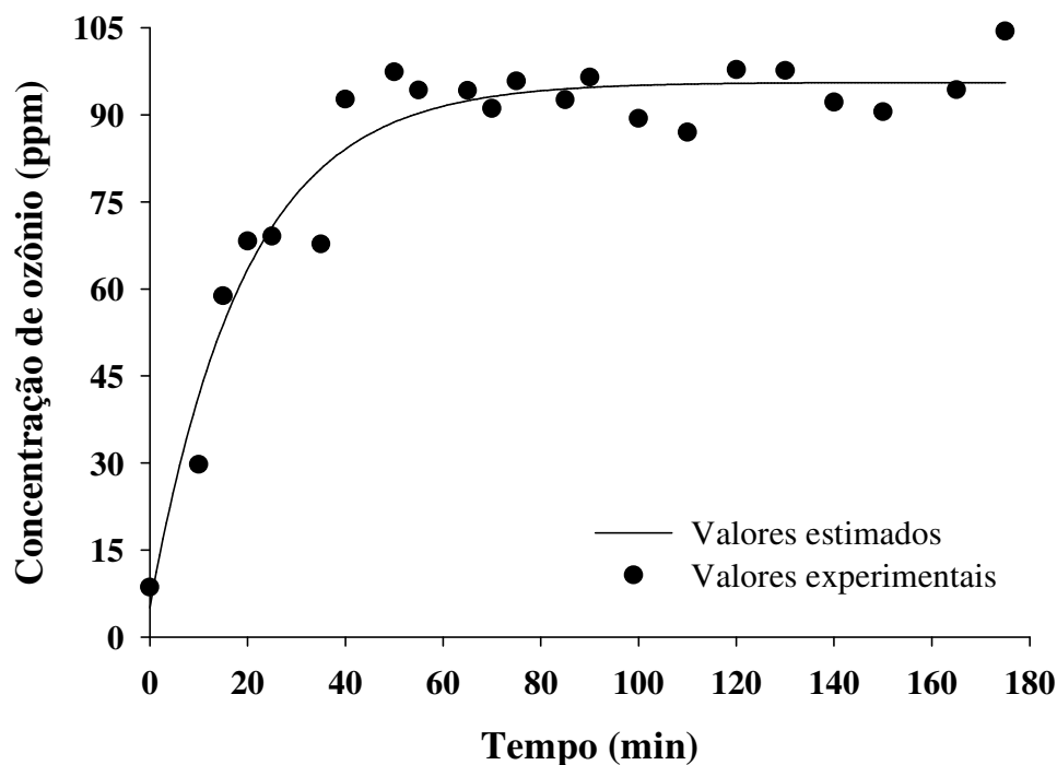
Figura 8 – Concentração residual de ozônio em grãos de milho em função do tempo na etapa de saturação.
