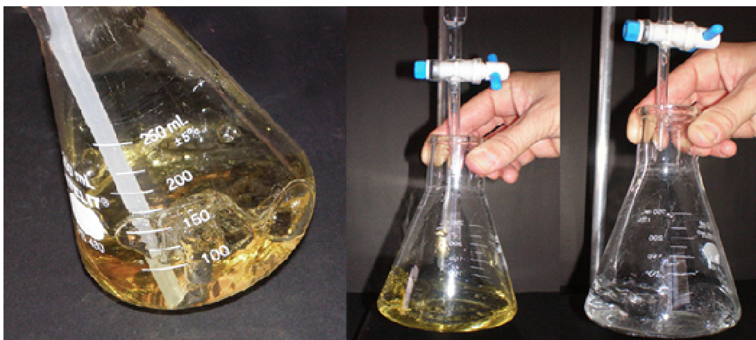
Figura 5 – Procedimento para quantificar o ozônio na corrente gasosa: (A) borbulhamento do O 3 em solução de KI e (B) titulação com Na 2 S 2 O 3 .
