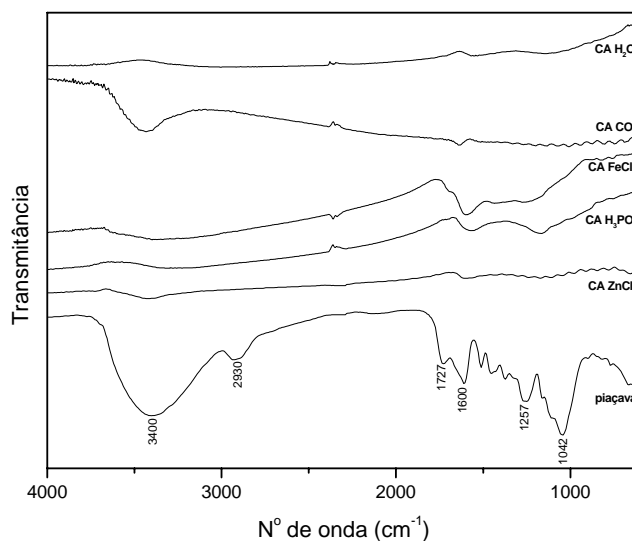
FIGURA 22. Espectros de infravermelho da piaçava, do CA \text{ZnCl}_2 , do CA \text{H}_3\text{PO}_4 , do CA \text{FeCl}_3 , do CA \text{CO}_2 e do CA \text{H}_2\text{O} .
