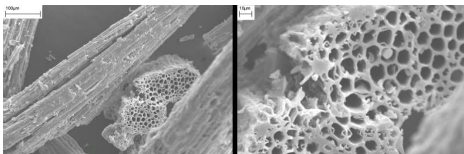
FIGURA 17. Micrografias do CA ZnCl 2 .
