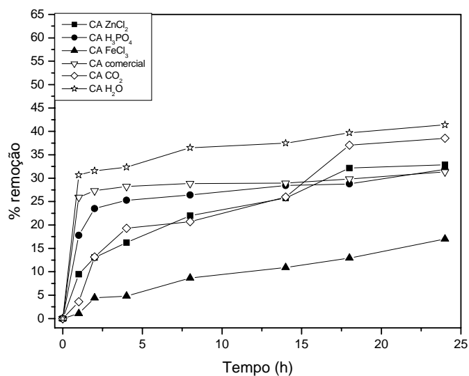
FIGURA 28. Cinética de adsorção de Zn +2 50 mg L -1 (10 mg de CA; 10 mL de solução; pH=4,6; agitação mecânica de 100 rpm; temperatura ambiente).
