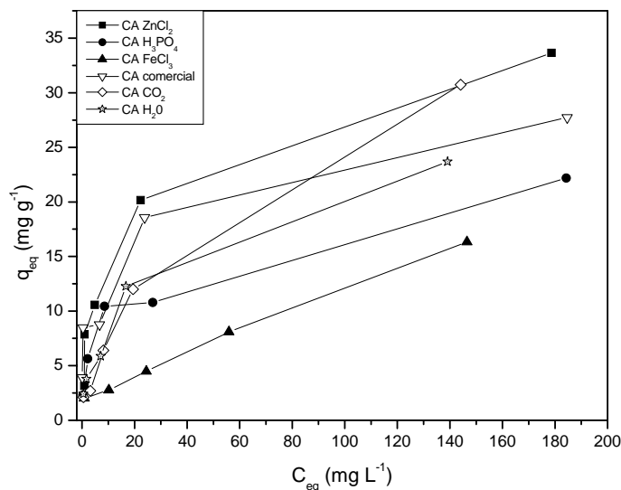
FIGURA 34. Isotermas de adsorção do íon Zn +2 (10 mg de CA; 10 mL de solução; pH=4,6-6,7; agitação mecânica de 100 rpm; temperatura ambiente).
