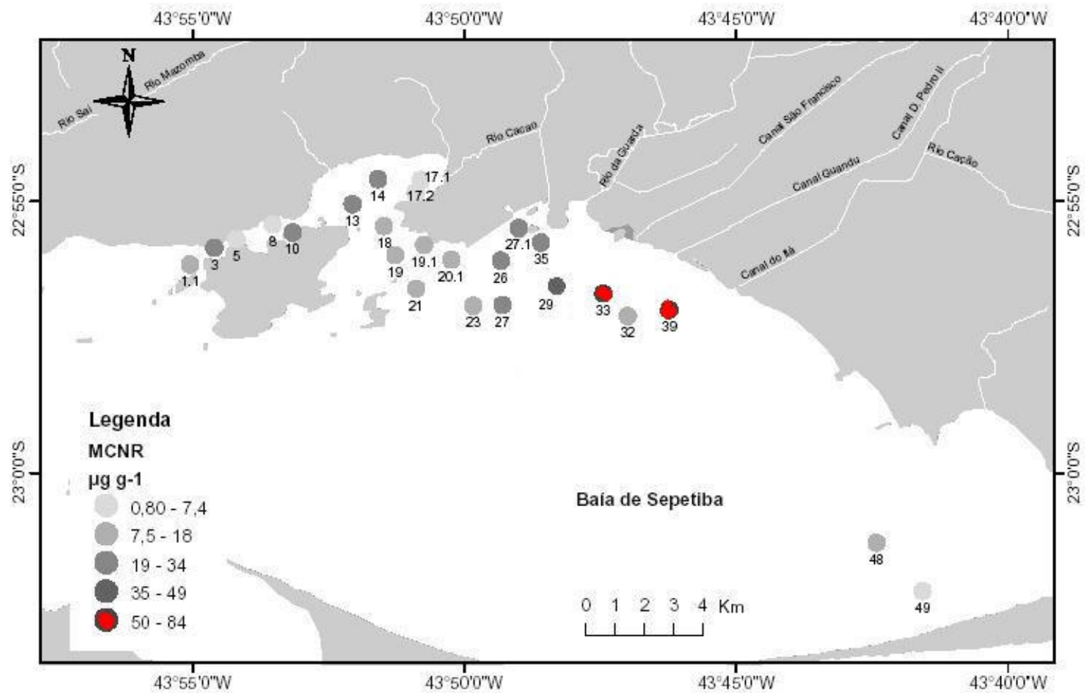
Figura 23 - Distribuição e concentração da mistura complexa não resolvida (MCNR) ( \mu\text{g.g}^{-1} ).
