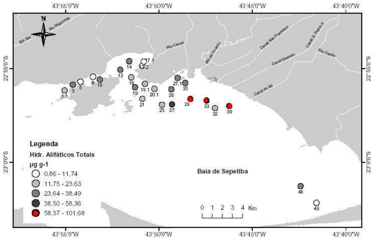
Figura 18 - Distribuição e concentração dos hidrocarbonetos alifáticos totais ( \mu\text{g}\cdot\text{g}^{-1} ).
