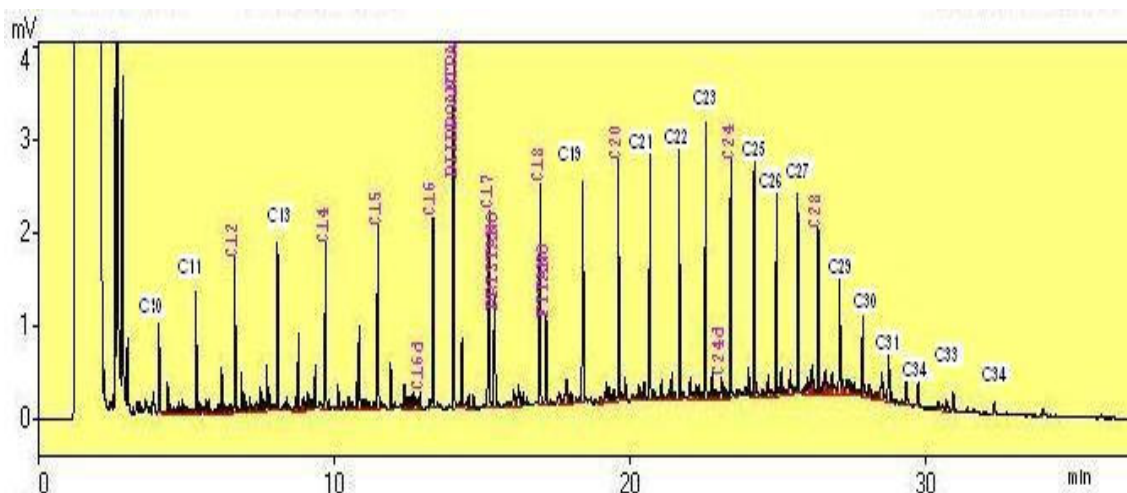
Figura 12 – Cromatograma de uma das amostras utilizadas na obtenção do tempo de retenção.
