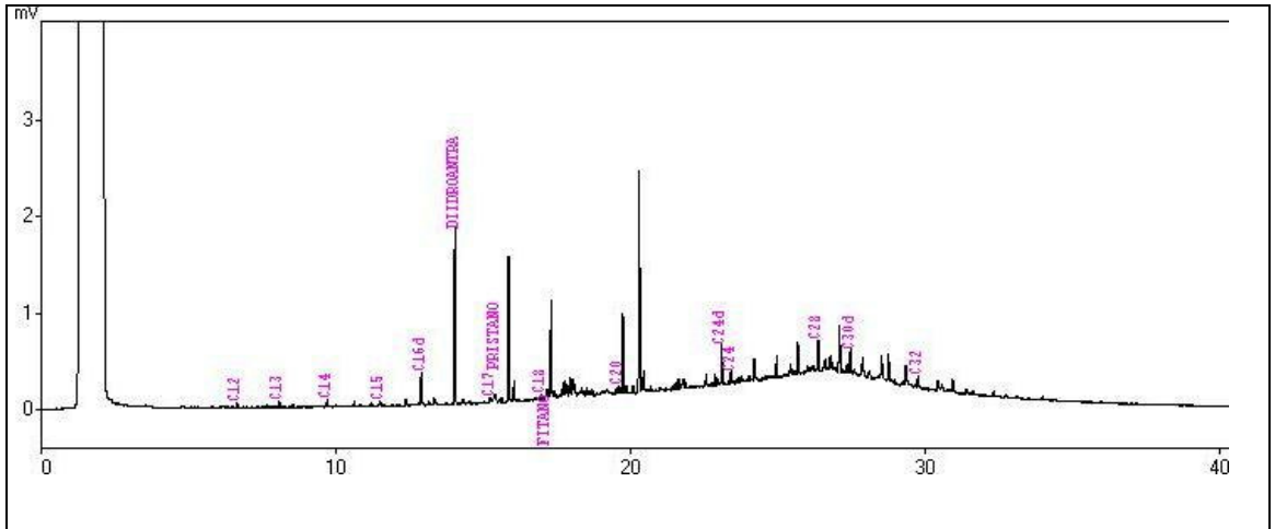
Cromatograma da amostra de sedimento SD1.
