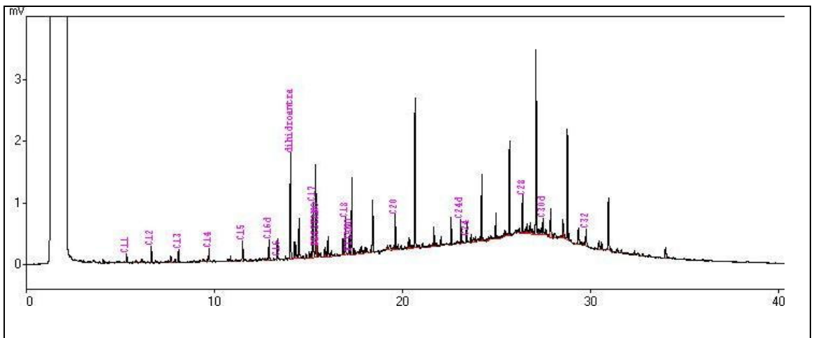
Cromatograma da amostra T4.
