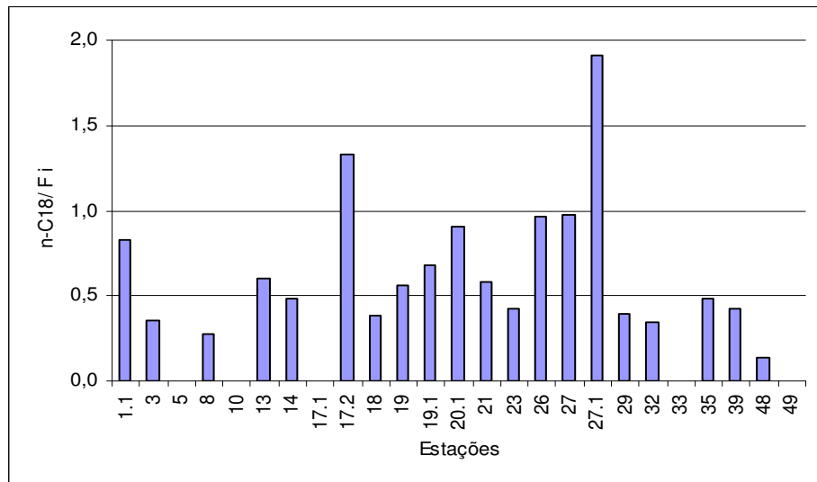
Figura 27 – Razão entre o n\text{-C}_{18} e o Fitano ( n\text{-C}_{18}/\text{Fi} ).
