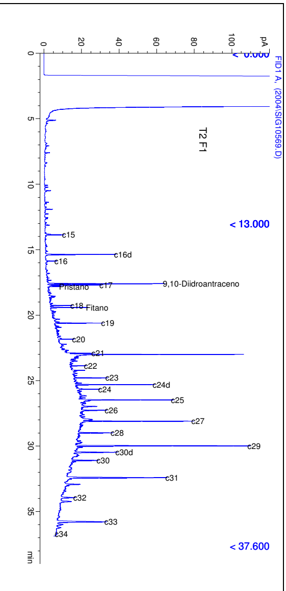
Cromatograma da amostra T2.
