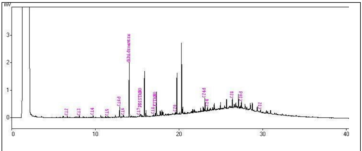
Cromatograma da amostra de sedimento SD2.
