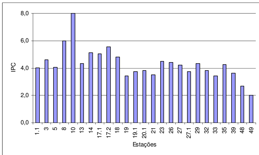
Figura 22 – Valores de IPC na Baía de Sepetiba.
