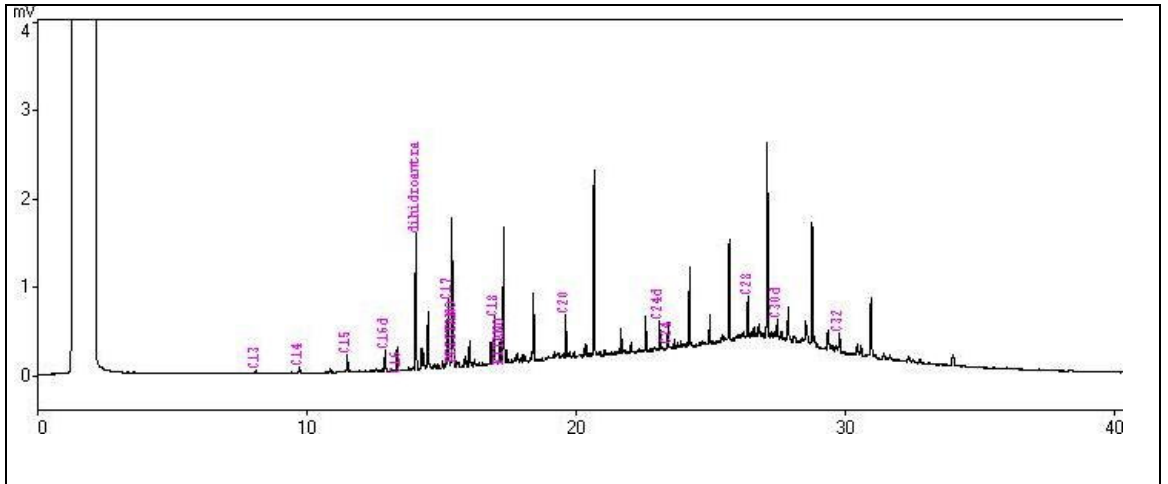
Cromatograma da amostra T1.
