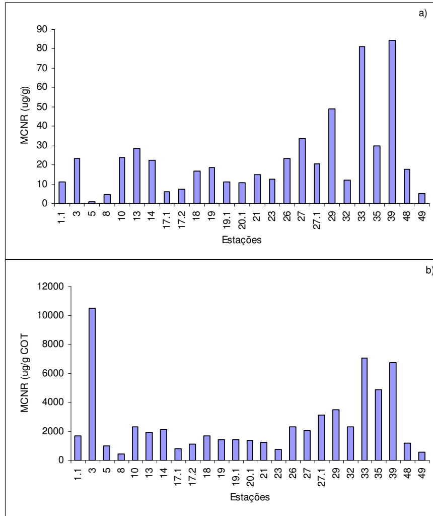
Figura 24 – Concentração da MCNR (a) e concentração da MCNR normalizados em COT (b) ( \mu\text{g.g}^{-1} ).
