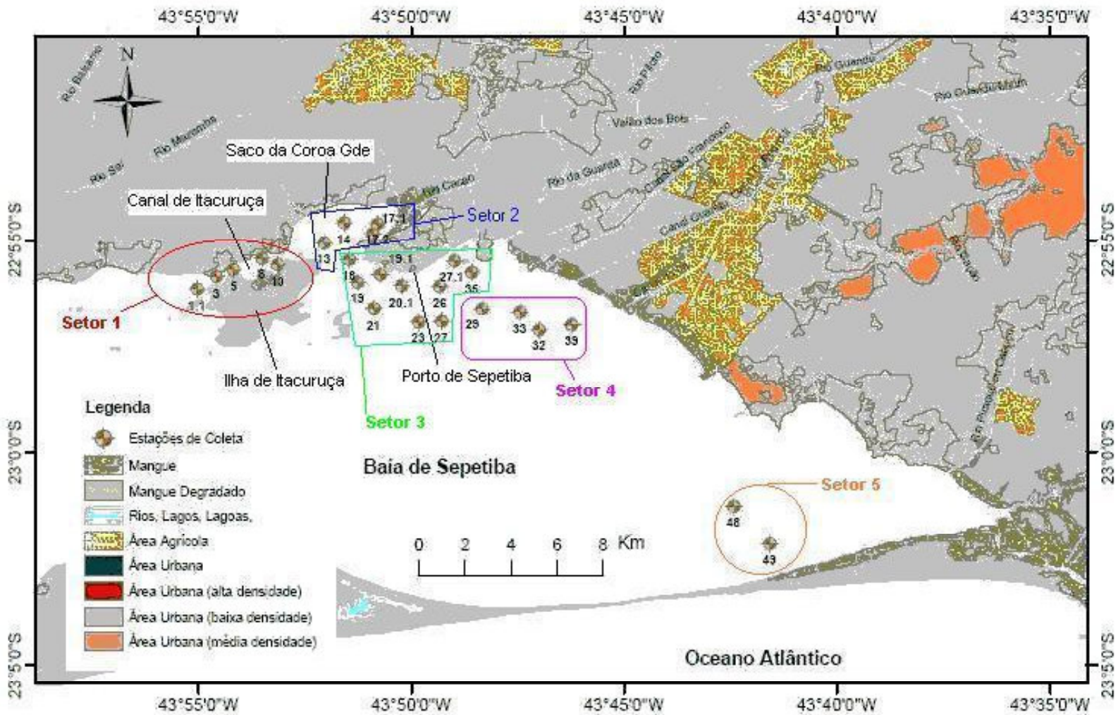
Figura 30 – Mapa dos setores na Baía de Sepetiba.
