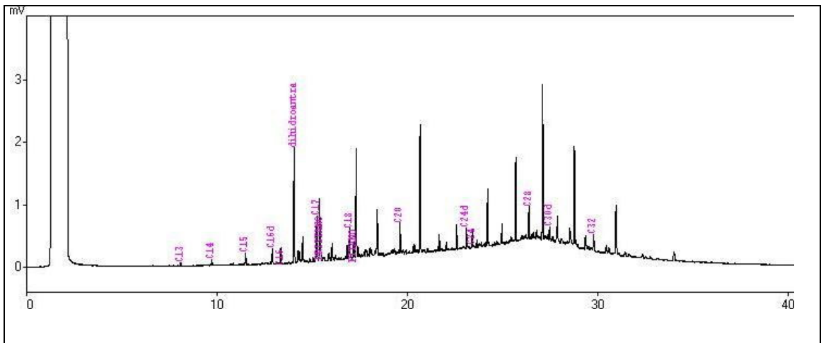
Cromatograma da amostra T3.
