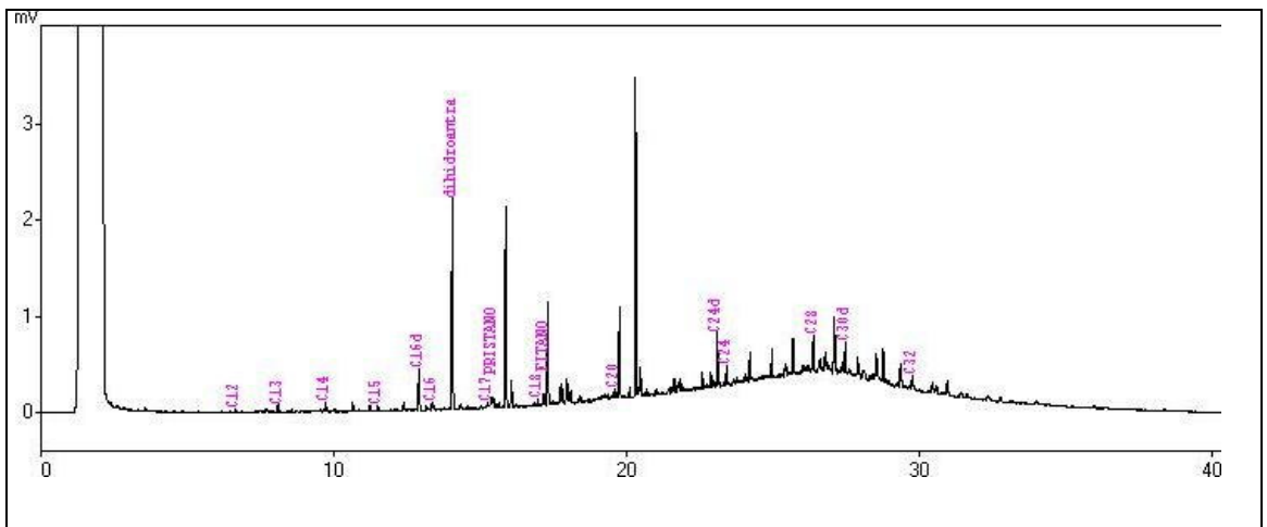
Cromatograma da amostra de sedimento SD3.
