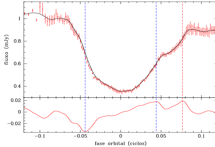
Fig. 6.2: O painel superior mostra os dados (pontos com barras de erro) e a mesma curva após a aplicação de de um filtro de mediana (linha sólida) para a curva de luz média extraída com o G160L e PRISM para a faixa espectral \lambda 1900 - 2500\text{\AA} . O quadro inferior apresenta a derivada da curva filtrada mostrada no painel superior. As linhas tracejadas verticais marcam a posição de ingresso e egresso da fonte central (em cinza escuro) e a posição de egresso de uma fonte assimétrica (em cinza claro).
