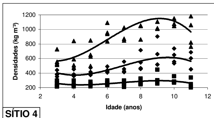
FIGURA 19 - EQUAÇÕES AJUSTADAS PARA DENSIDADE ESPECÍFICA MÁXIMA ( \blacktriangle ), DENSIDADE ESPECÍFICA MÉDIA ( \blacklozenge ) E DENSIDADE ESPECÍFICA MÍNIMA ( \blacksquare ) EM CADA ANEL ANUAL DE CRESCIMENTO DOS 3 AOS 11 ANOS NOS DIFERENTES SÍTIOS PARA O DISCO COLETADO AO DAP
