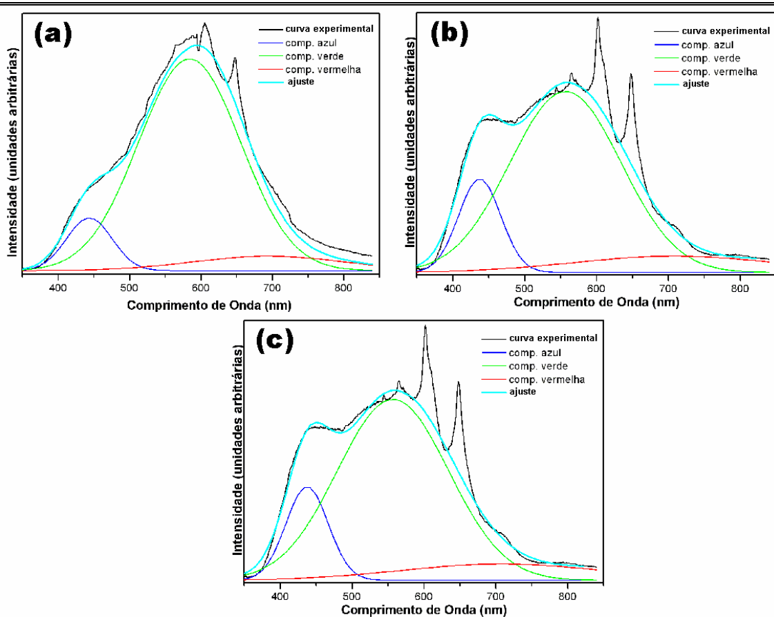
FIGURA 4.14: Decomposição das curvas de emissão FL para o CT:Sm tratado termicamente a (a) 450, (b) 500 e (c) 550 °C.
