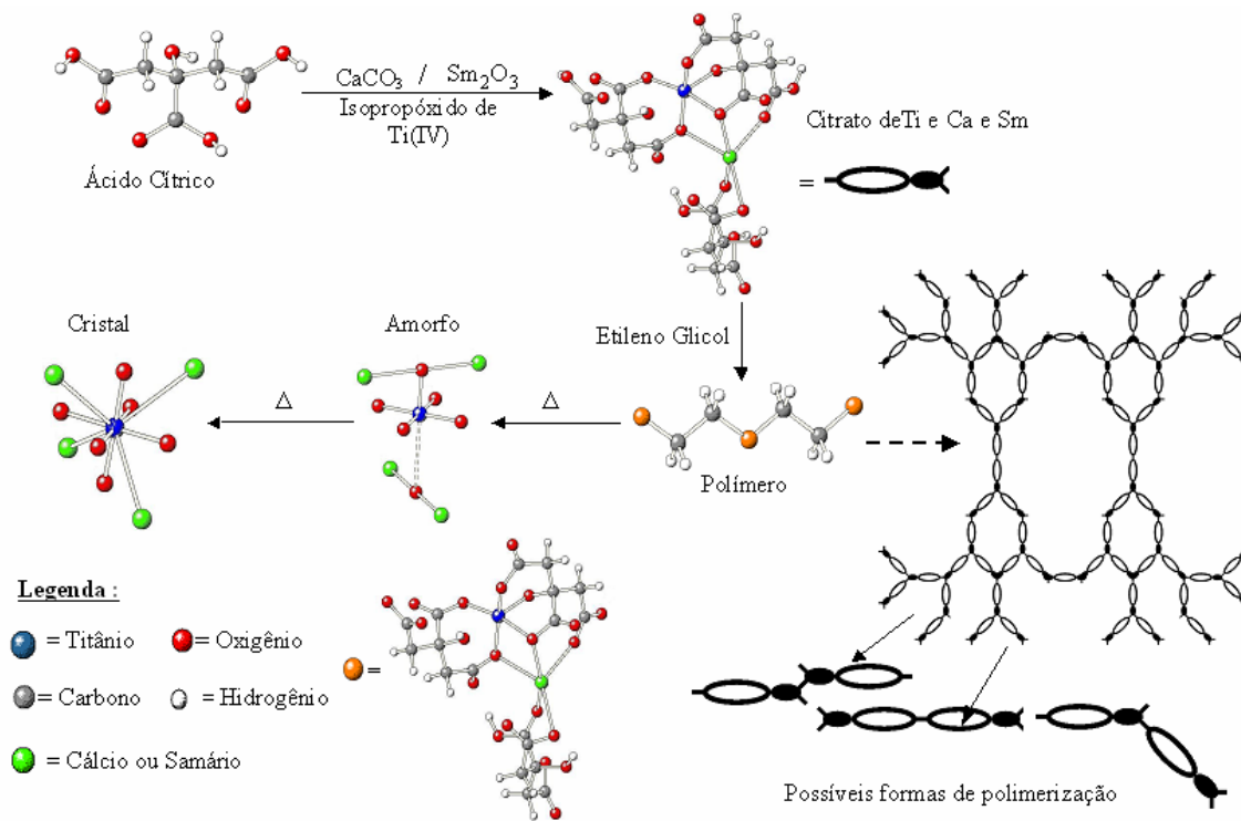
FIGURA 4.1: Esquema de síntese do CT:Sm pelo método Pechini.
