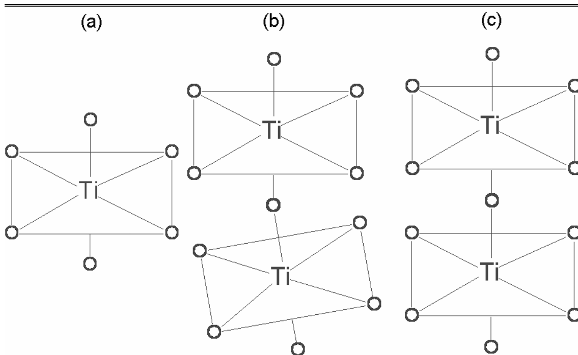
FIGURA 1.6: Ordem estrutural (a) a curta distância, (b) a média distância e (c) a longa distância nos titanatos.
