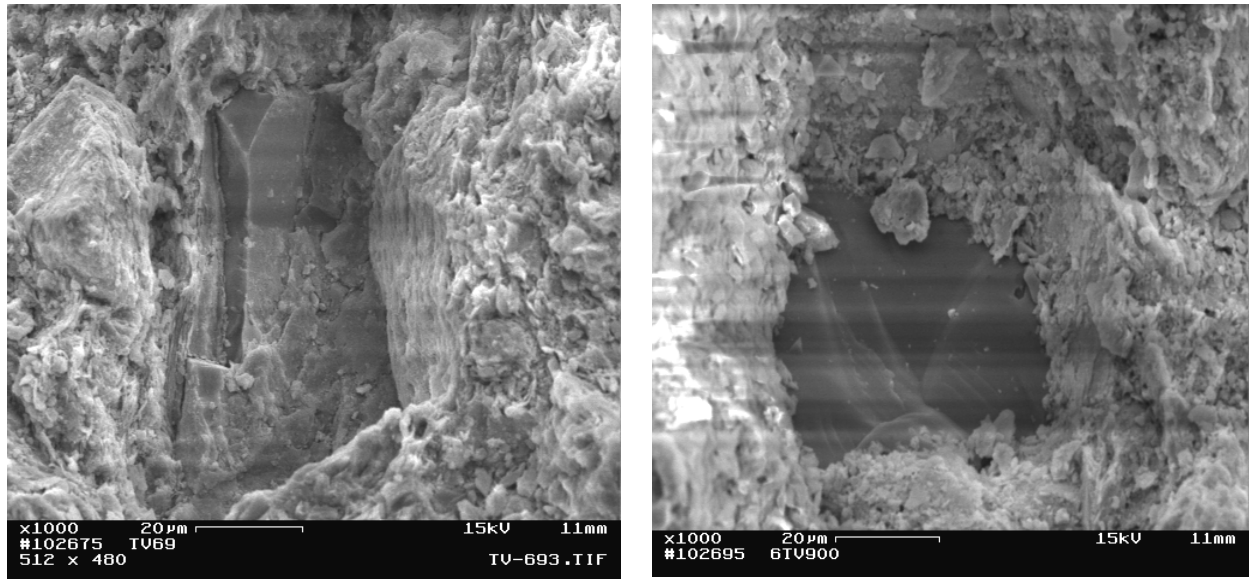
Figura 4.45- Microestrutura da argila com 6% de vidro de tubo de TV, sinterizada a 900°C (1000x).
