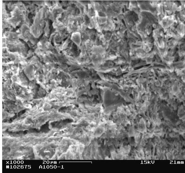
Figura 4.40- Microestrutura da argila pura sinterizada a 1050°C (1000x).
