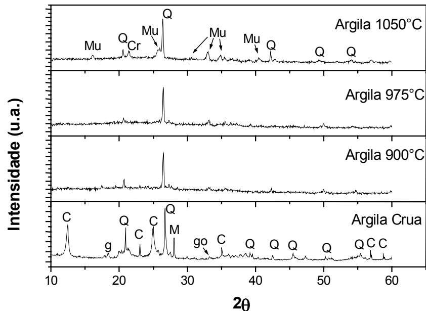
Figura 4.10 – Difratoogramas de raios-X da argila pura utilizada, queimada nas três temperaturas de queima.
