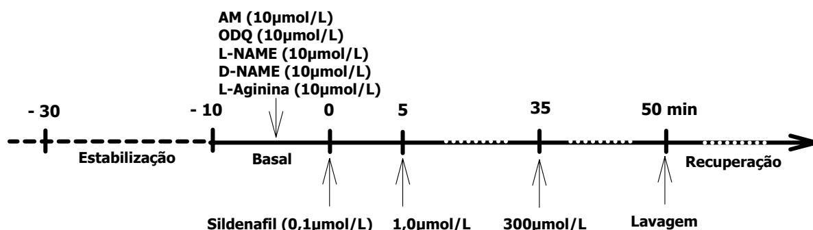
Figura 2.4.4 – Delineamento experimental utilizado para avaliação do efeito do pré-tratamento com azul de metileno (AM) ( 10\mu\text{mol/L} ), ODQ ( 10\mu\text{mol/L} ), L-NAME ( 10\mu\text{mol/L} ), D-NAME ( 10\mu\text{mol/L} ) e L-arginina ( 10\mu\text{mol/L} ) sobre a propriedade mio-relaxante do sildenafil (doses crescentes e cumulativas – 0,1 a 300\mu\text{mol/L} ) observada em tiras isoladas de duodeno de ratos ex vivo .
