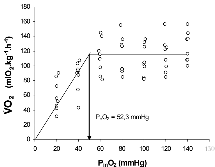
Figura 9- Efeito da redução gradual das tensões de oxigênio da água de entrada do respirômetro ( P_{in}O_2 – mmHg) sobre o consumo de oxigênio ( \dot{V}O_2 – mlO 2 .kg -1 .h -1 ) do grupo exposto ao MP (n = 8) de B. cephalus . A seta representa a P_{c}O_2 .
