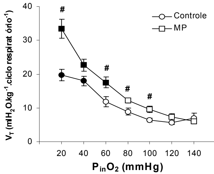
Figura 13- Efeito da redução gradual das tensões de oxigênio da água ( P_{in}O_2 – mmHg) sobre o volume ventilatório ( V_T - mlH_2O.kg^{-1}.ciclo\ respiratório^{-1} ) dos grupos controle ( n = 8 ) e exposto ao MP ( n = 8 ) de B. cephalus . Valores médios \pm 1 E.P.M. #: diferença significativa entre os grupos experimentais. Os símbolos cheios indicam diferença em relação aos valores obtidos em normóxia ( p < 0,05 ).
