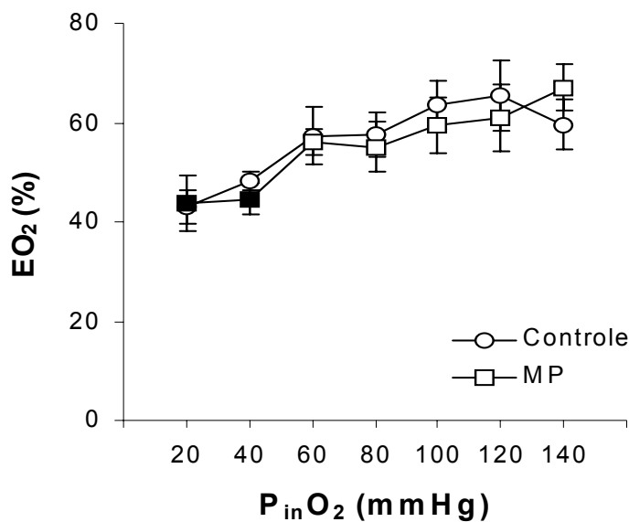
Figura 15- Efeito da redução gradual das tensões de oxigênio da água (P in O 2 – mmHg) sobre a extração de O 2 (EO 2 - %) dos grupos controle (n = 8) e exposto ao MP (n = 8) de B. cephalus . Valores médios ± 1 E.P.M. Os símbolos cheios indicam diferença em relação aos valores obtidos em normóxia (p < 0,05).
