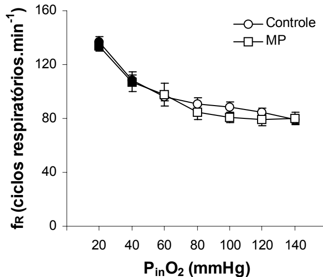
Figura 12- Efeito da redução gradual das tensões de oxigênio da água ( P_{in}O_2 – mmHg) sobre a frequência respiratória ( f_R – ciclos respiratórios.min -1 ) dos grupos controle (n = 8) e exposto ao MP (n = 8) de B. cephalus . Valores médios \pm 1 E.P.M. Os símbolos cheios indicam diferença em relação aos valores obtidos em normóxia ( p < 0,05 ).
