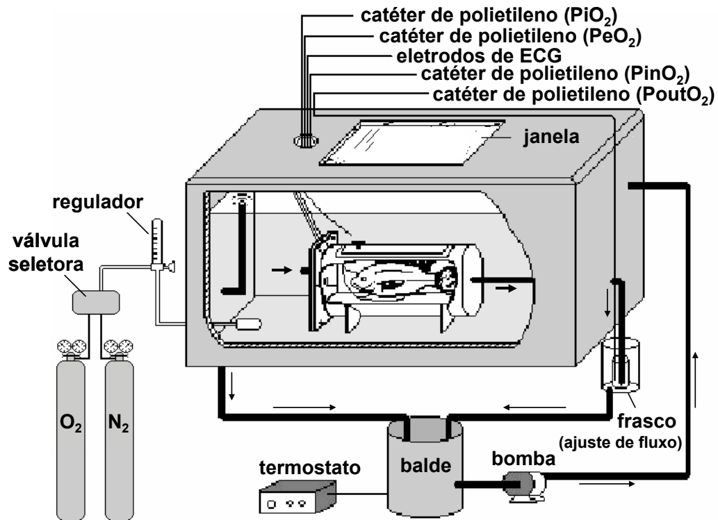
Figura 4- Esquema do sistema experimental utilizado nos experimentos in vivo .
