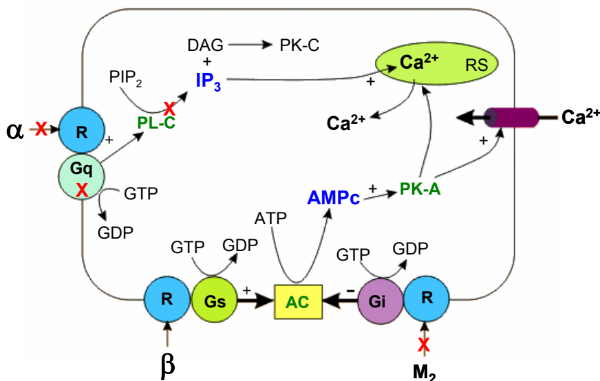
Figura 36- Esquema das vias de ativação adrenérgica em um miócito cardíaco e dos locais de ação de inseticidas organofosforados (OPs). Os sítios de inibição pelos OPs estão assinalados com um X vermelho. PL-C – fosfolipase C; PK-C – proteína-quinase C; AC – adenil-ciclase; AMPc – adenosina monofosfato cíclico; M 2 – receptor muscarínico tipo 2; \alpha - receptores \alpha -adrenérgicos; \beta - receptores \beta -adrenérgicos.
