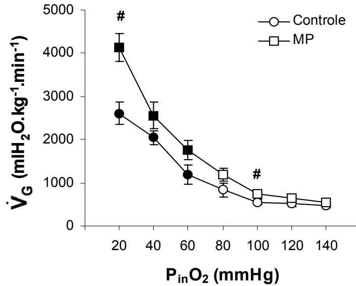
Figura 11- Efeito da redução gradual das tensões de oxigênio da água ( P_{in}O_2 – mmHg) sobre a ventilação branquial ( \dot{V}_G - mlH 2 O.kg -1 .min -1 ) dos grupos controle (n = 8) e exposto ao MP (n = 8) de B. cephalus . Valores médios \pm 1 E.P.M. #: diferença significativa entre os grupos experimentais. Os símbolos cheios indicam diferença em relação aos valores obtidos em normóxia ( p < 0,05 ).
