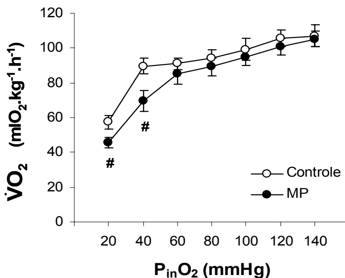
Figura 10- Efeito da redução gradual das tensões de oxigênio da água de entrada do respirômetro ( P_{in}O_2 – mmHg) sobre o consumo de oxigênio ( \dot{V}O_2 – mlO 2 .kg -1 .h -1 ) dos grupos controle (n = 8) e exposto ao MP (n = 8) de B. cephalus . Valores médios \pm 1 E.P.M. #: diferença significativa entre os grupos experimentais ( p < 0,05 ).
