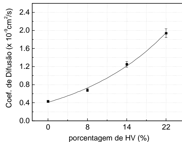
Figura 55 – Gráfico do coeficiente de difusão do dióxido de carbono em função do conteúdo de hidroxivalerato em copolímeros com poli(3-hidroxi-3-butirato) de estrutura P3(HB-x%HV).
