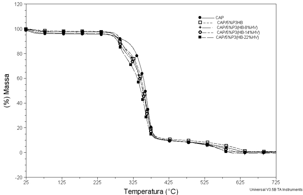
Figura 35 – Perfil TGA das misturas CAP e 5% m/m de P3HB, P3(HB-8%HV), P3(HB-14%HV) e P3(HB-22%HV) respectivamente.
