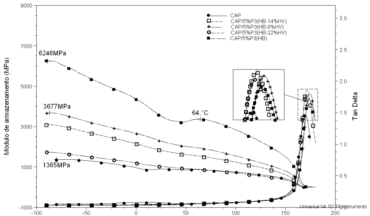
Figura 43 – Termograma de DMA relativo aos módulos de perda e \tan \delta relativo dos filmes densos do CAP e as misturas com 5% de poli(3-hidroxicanoatos) em função da temperatura.
