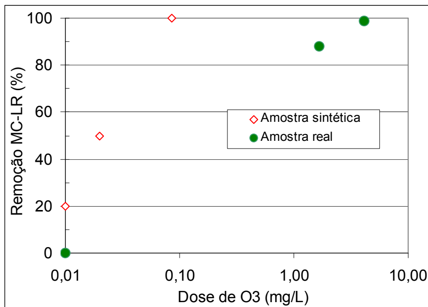
Figura 5.16. Percentual de remoção de MC-LR ( 0,03 \text{ mg L}^{-1} ) em amostra real e amostra sintética ( 0,1 \text{ mg L}^{-1} ) para diferentes doses de ozônio.
