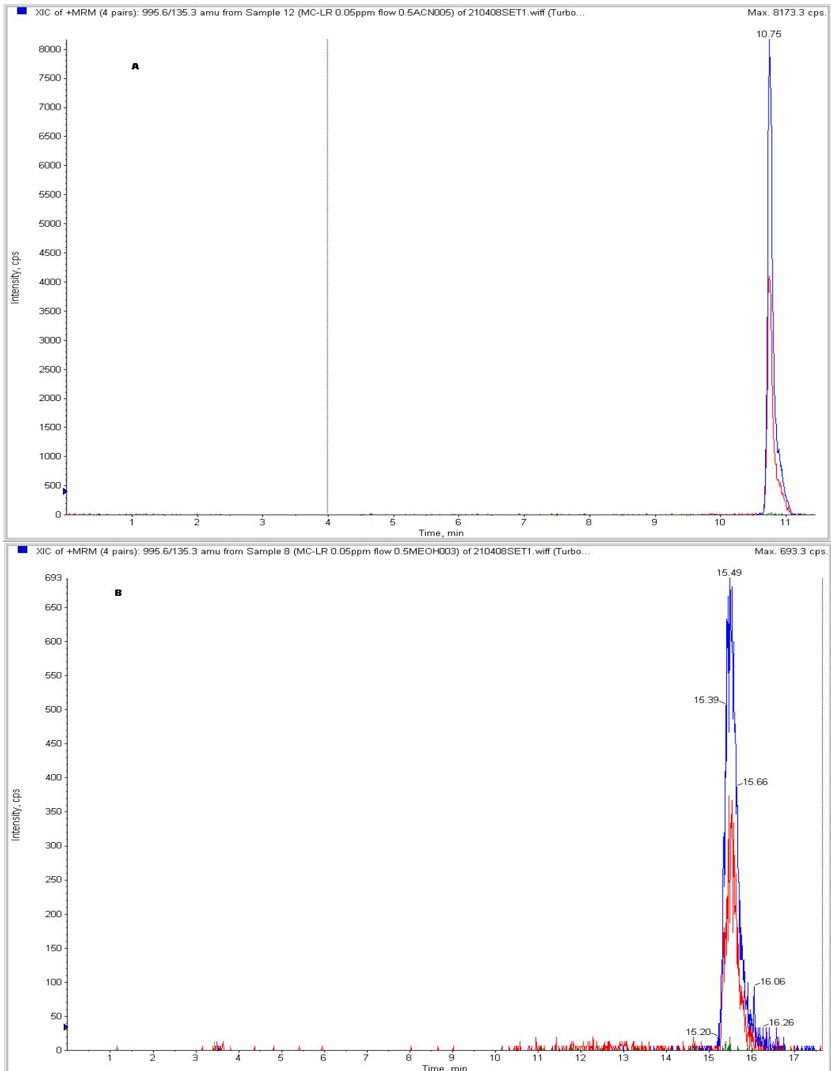
Figura 5.4. Cromatogramas de análise de MC-LR utilizando-se como componentes da fase móvel acetonitrila (A) e metanol (B) juntamente com água, ambos com 2mM de acetato de amônio e 0,1 % ácido fórmico.
