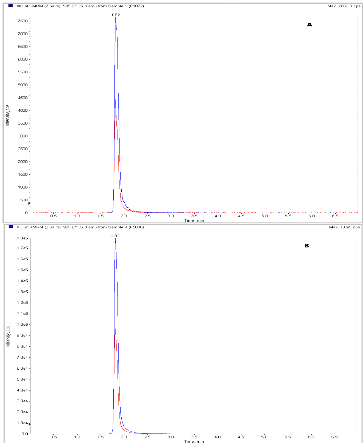
Figura 5.10. Cromatogramas de análise do primeiro nível de fortificação com MC-LR ( 0,1 \mu\text{g L}^{-1} ) (A) e do último nível de fortificação ( 1,0 \mu\text{g L}^{-1} ) (B).
