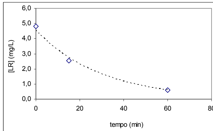
Figura 5.11. Decréscimo da concentração de MC-LR através da reação com ozônio ( 0,3 \text{ mg L}^{-1} ), durante 15 e 60 min.
