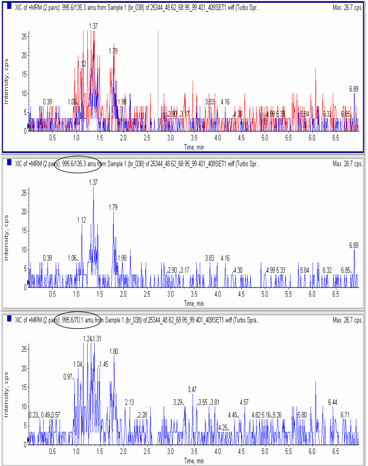
Figura 5.7. Cromatograma de análise do branco de matriz, água potável indicando as duas fragmentações monitoradas (135,3 e 70,1).
