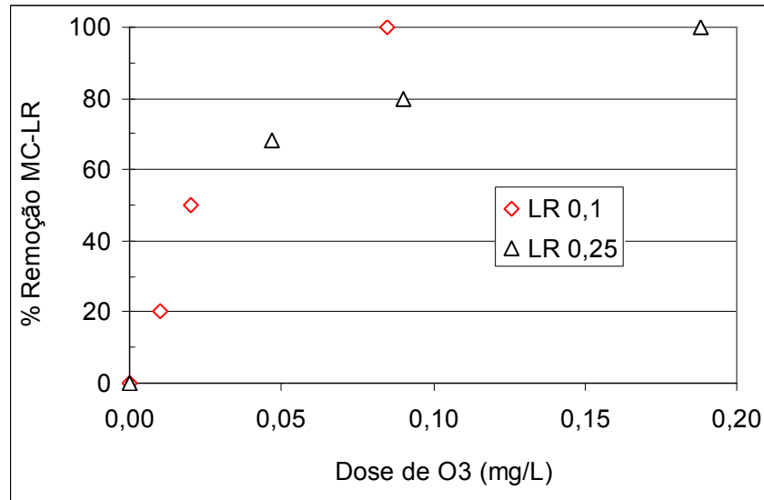
Figura 5.14. Percentual de remoção de MC-LR nas concentrações de 0,1 e 0,25 mg L -1 para diferentes doses de ozônio.
