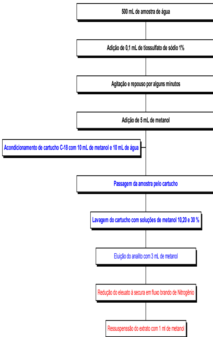
Figura 4.1. Fluxograma do procedimento de preparação de amostras de águas para análise de MC-LR.
