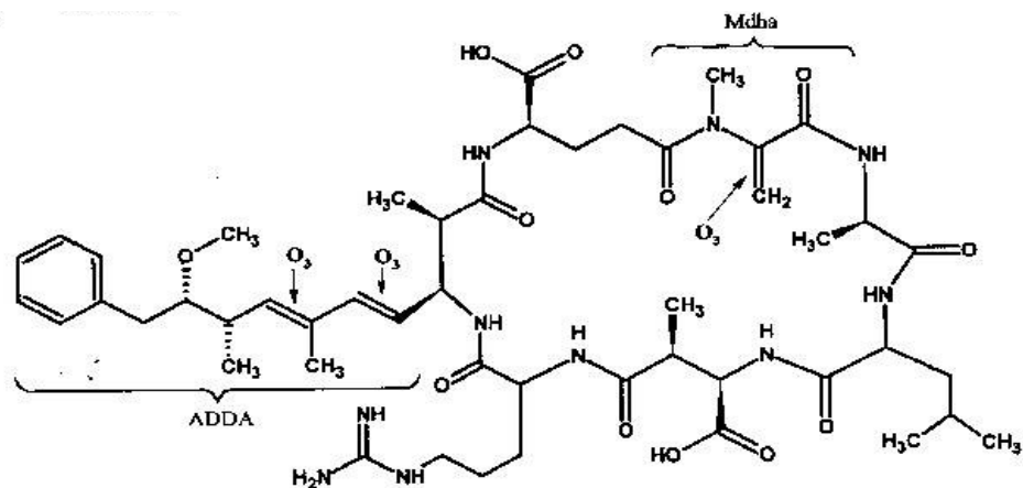
Figura 3.7. Proposta de sítios de ataque do ozônio( \text{O}_3 ) para a molécula de MC-LR (Onstad et al. , 2007).
