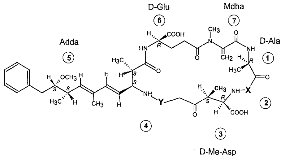
Figura 3.1. Estrutura geral de microcistinas. (Dahlmann et al. , 2003).
