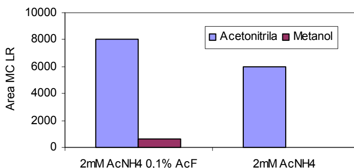
Figura 5.3. Representação gráfica da otimização da fase móvel utilizando acetonitrila e metanol como componente orgânico e acetato de amônio (AcNH4) e ácido fórmico (AcF) como aditivos.
