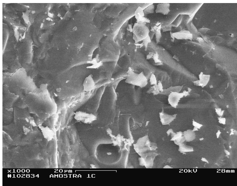
Figura 50 – Amostra 1Ca (granulometria do diamante = 40/28 µm, arranjo tipo a , P = 5,0 GPa, T = 1450^{\circ}\text{C} , t = 10\text{s} ) amostra não retificada.
