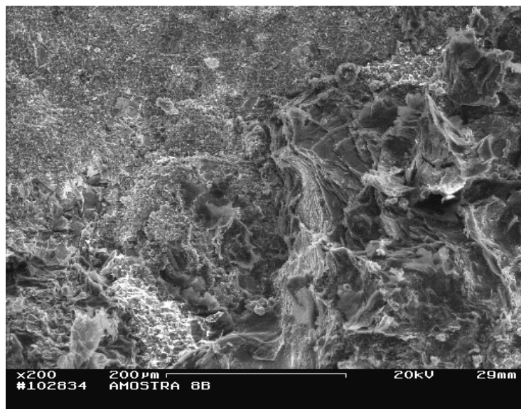
Figura 51 – Amostra 8Bb (granulometria do diamante = 14/10 μm, arranjo tipo b, P = 6,0 GPa, T = 1800°C, t = 30s) amostra não retificada.
