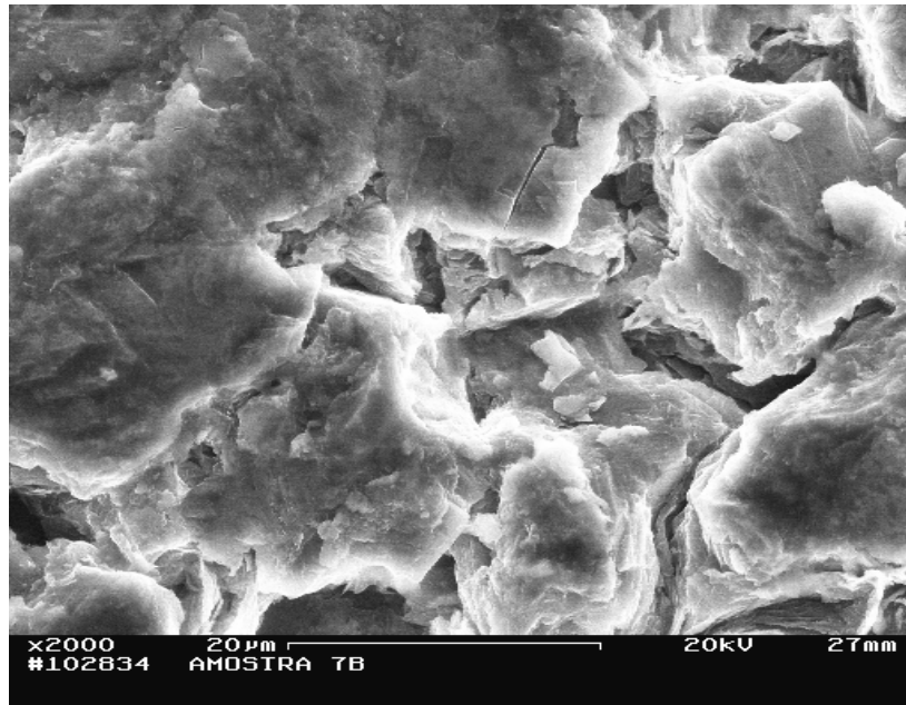
Figura 49 – Amostra 7Bb (granulometria do diamante = 14/10 µm, arranjo tipo b , P = 6,0 GPa, T = 1800^{\circ}\text{C} , t = 30\text{s} ) amostra não retificada.
