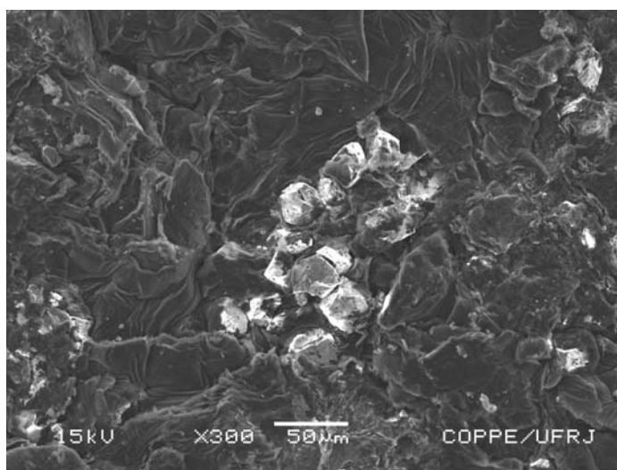
Figura 52 – Amostra 11Ab (granulometria do diamante = 40/28 μm, arranjo tipo b, P = 7,7 GPa, T = 1600°C, t = 20s) amostra não retificada.
