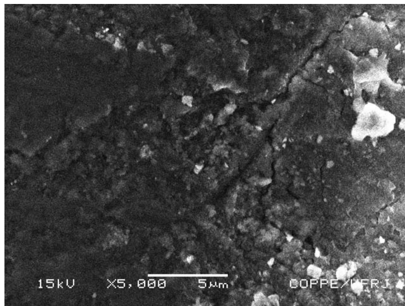
Figura 34 – Amostra 3Ab (granulometria do diamante = 40/28 \mu\text{m} , arranjo tipo b , P = 6,0 GPa, T = 1400^\circ\text{C} , t = 20\text{s} ) amostra retificada.
