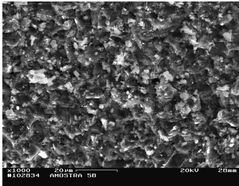
Figura 32 – Amostra 5Bb (granulometria do diamante = 14/10 μm, arranjo tipo b , P = 7,7 GPa, T = 1800^{\circ}\text{C} , t = 30\text{s} ) amostra não retificada.
