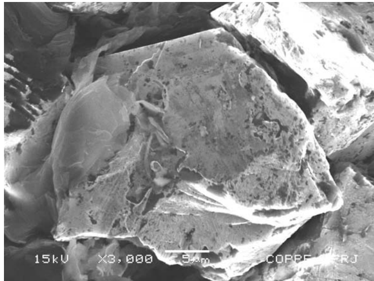
Figura 47 – Amostra 11Ab (granulometria do diamante = 40/28 \mu\text{m} , arranjo tipo b , P = 7,7 GPa, T = 1600^\circ\text{C} , t = 20\text{s} ) amostra não retificada.
