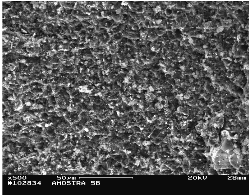
Figura 31 – Amostra 5Bb (granulometria do diamante = 14/10 μm, arranjo tipo b , P = 7,7 GPa, T = 1800^{\circ}\text{C} , t = 30\text{s} ) amostra não retificada.
