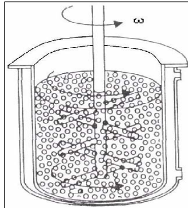
Figura 2.6 – Esquema de um Moinho Atritor (Janot et al, 2005).
