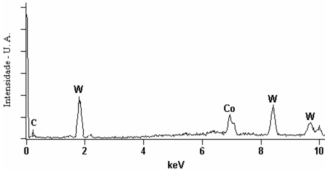
Figura 4.20 – EDS dos pós com PM=3:1 e 5h de MAE.
