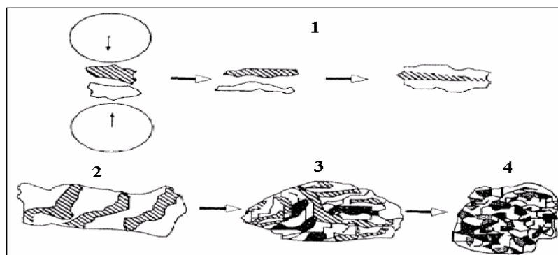
Figura 2.3 – Evolução típica da mistura de pós durante a MAE (Gaffet et al, 2002).
