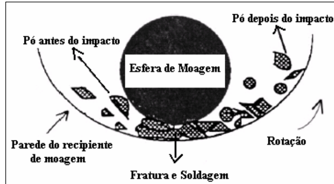
Figura 2.2 - Colisão entre esfera - pó - parede do recipiente em MAE (Janot et al, 2005).
