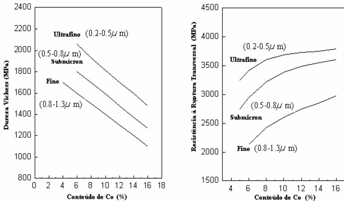
Figura 2.13 – Dependência da dureza e resistência à ruptura transversal de WC-Co com diferentes tamanhos de grão em função da porcentagem de conteúdo do cobalto (Zhang et al, 2003).
