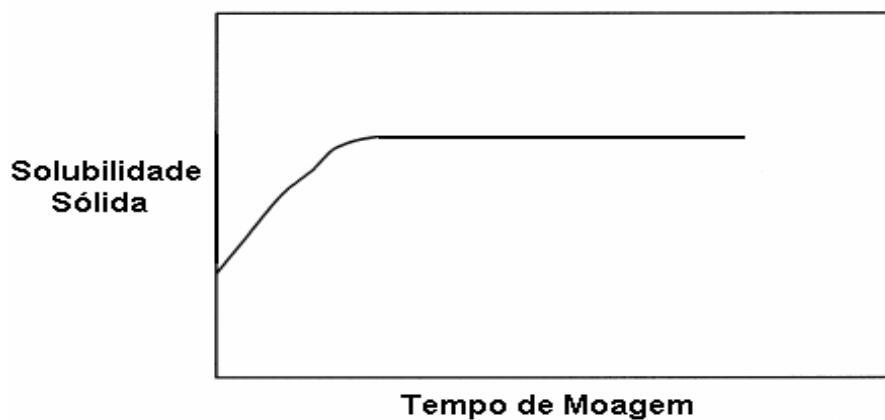
Figura 2.10 – Solubilidade Sólida em função do tempo de moagem (Suryanarayana, 2001).
