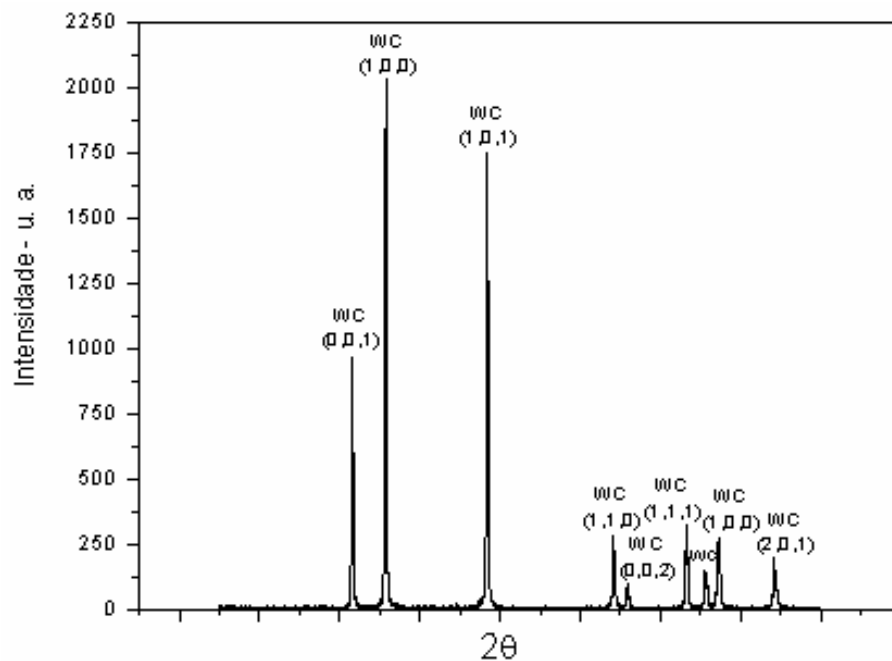
Figura 4.3 - Difratoograma de raios-X do pó de WC-10%Co apenas misturado.
