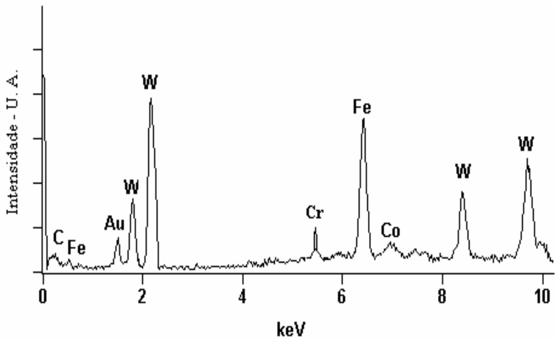
Figura 4.23 – EDS dos pós com PM = 3:1 e 150h de MAE.
