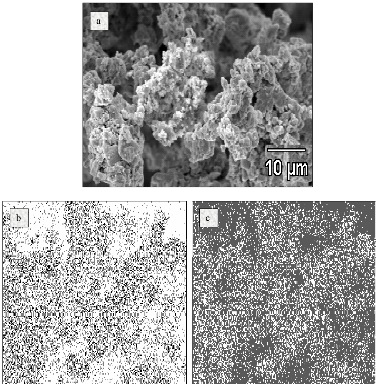
Figura 4.19 – EDS nas partículas de WC-10Co (4000X), com 150 horas de MAE, para PM = 3:1: a) WCCo; b) W; c) Co.
