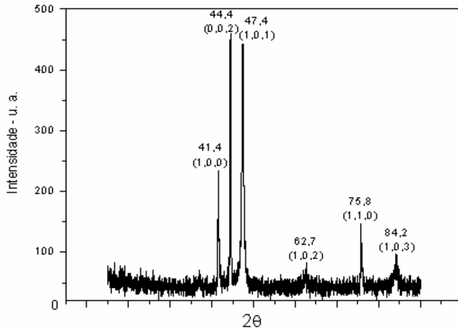
Figura 4.2 - Difratoograma de raios-X do pó de Co usado como matéria-prima na preparação do pó de metal duro por MAE.
