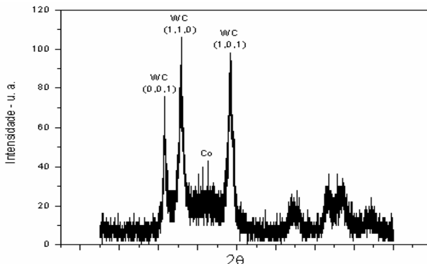
Figura 4.27 – Difratoograma de raios-X do pó composto WC-10%Co preparado por MAE a úmido durante 150 h.
