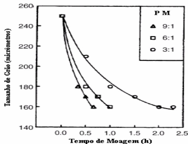
Figura 2.9 – Refino do tamanho de partícula com o tempo de moagem e poder de microforjamento (apud Schaffer et al, 1992; Janot et al, 2005).
