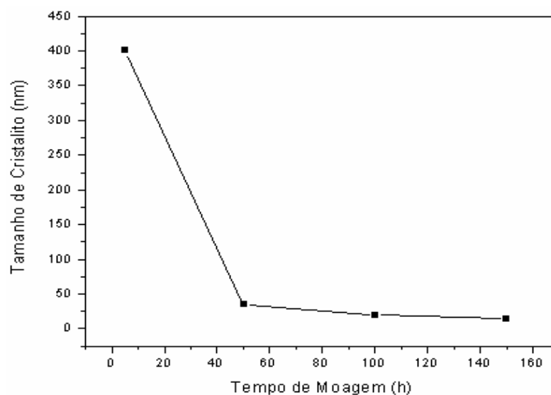
Figura 4.11 – Variação do tamanho de cristalito da fase WC (100) com o tempo de moagem do pó compósito WC-10%Co preparado por MAE com PM = 3:1.
