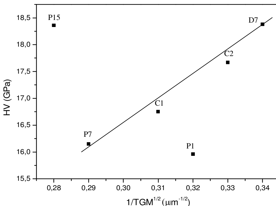
Figura 94 - Relação de Hall-Petch para as amostras C1, C2, P1, P7, P15 e D7.
