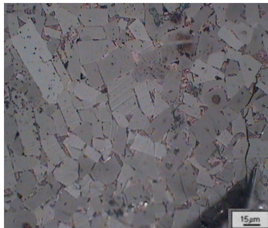
Figura 44 - Micrografia da amostra D1 (5GPa/1300°C/2min) - 400X.
