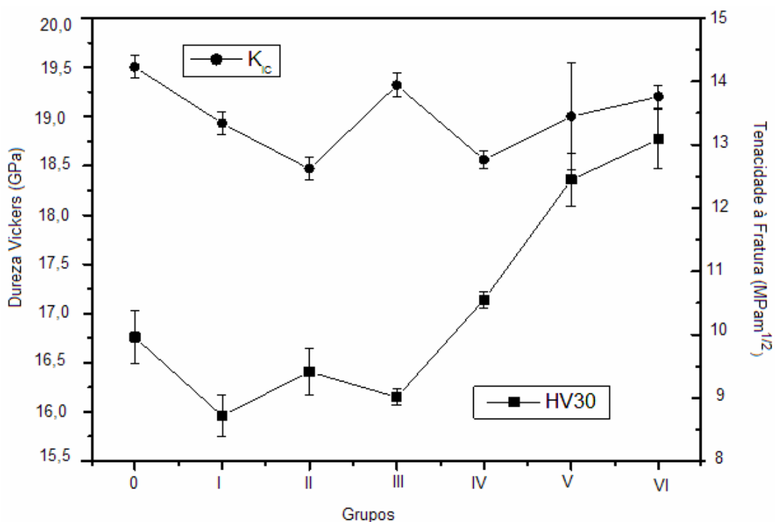
Figura 92 – Variação da Dureza Vickers versus Tenacidade à Fratura dos grupos das amostras puras.
