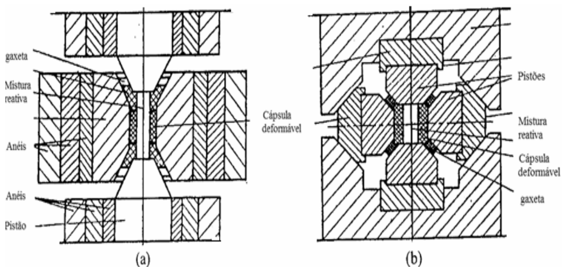
Figura 23 - Esquemas dos dispositivos de alta pressão do tipo: (a) Belt e (b) Multipistões [Novikov et al. , 1991].
