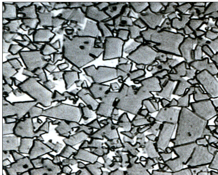
Figura 2 - Fotomicrografia de um carbeto cementado WC-Co. Ampliação de 100× [Callister, 2002].
