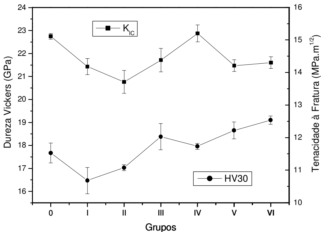
Figura 93 – Variação da Dureza Vickers versus Tenacidade à Fratura dos grupos das amostras dopadas.
