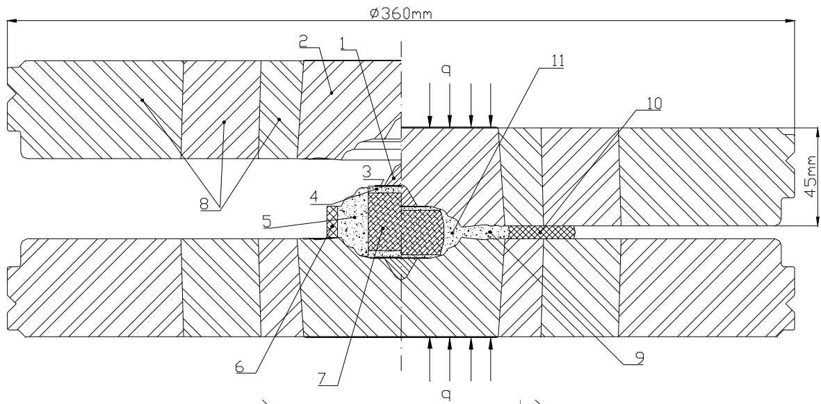
Figura 26 - Esquema mostrando a deformação da célula reativa no DAP. (1) Cone protetor (2) Bigorna (3) Disco de molibdênio (4) Tampa de calcita (5) Cápsula deformável de calcita (6) Anel de PVC (7) Mistura (8) Anéis de cintamento (9) Gaxeta formada (10) Anel de PVC deformado (11) Cápsula após deformação (q) Carga aplicada [Bobrovnitchii, 1998].
