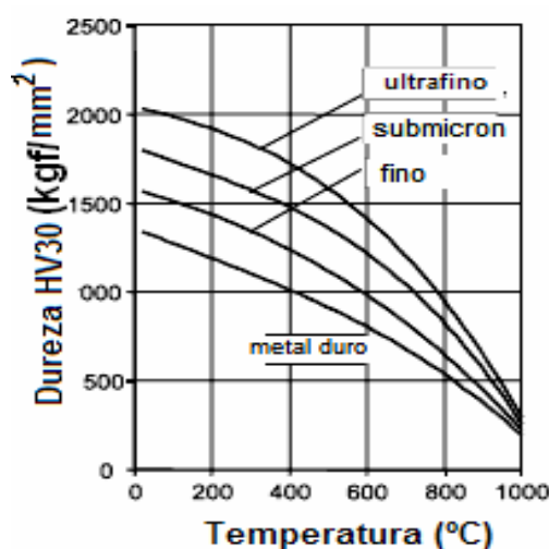
Figura 8 - Dureza Vickers em função da temperatura de trabalho do metal duro convencional, fino, submicron e ultrafino. [Gille et al. , 2002].
