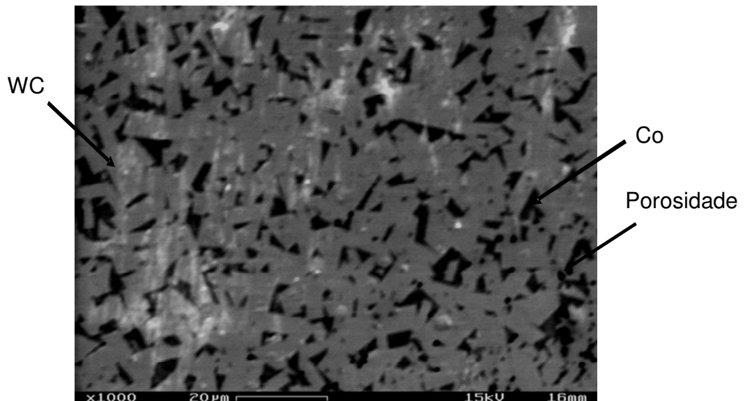
Figura 54 - Micrografia da amostra convencional dopada C2
