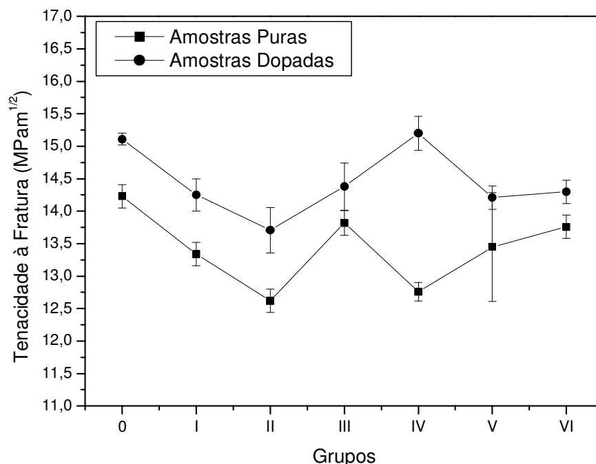
Figura 90 - Tenacidade à Fratura das amostras de metal duro sinterizadas.
