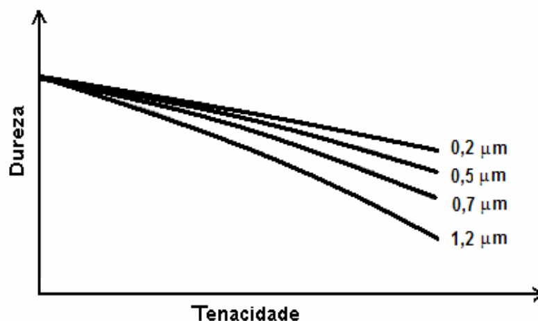
Figura 4 - Dureza e Tenacidade de carbetos cementados produzidos com pós de WC com diferentes granulometrias [North et al. , 1991].
