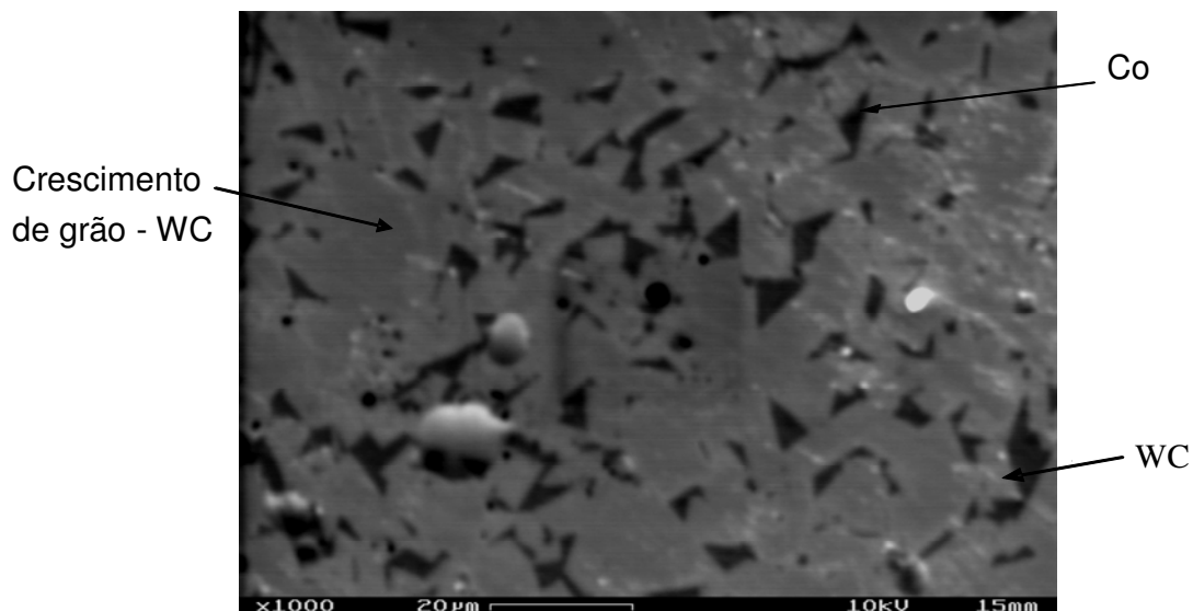
Figura 55 - Micrografia da amostra P1 (5GPa/1300°C/2min).
