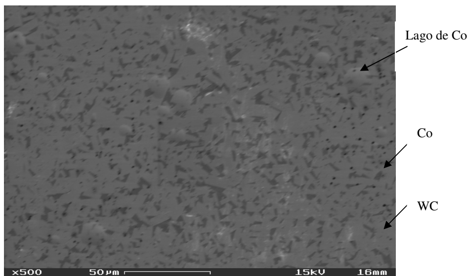
Figura 59 - Micrografia da amostra D7 (5GPa/1400°C/2min).
