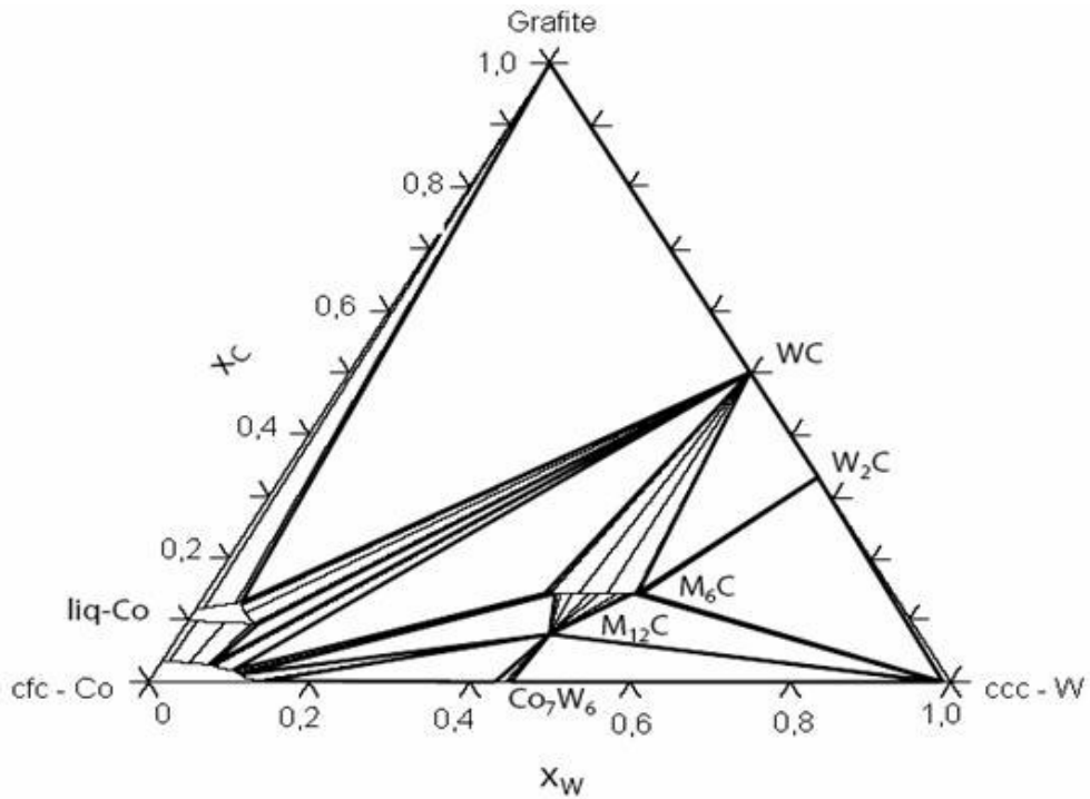
Figura 77 - Seção isotérmica do diagrama Co-W-C a 1350°C [Pettersson, 2004].
