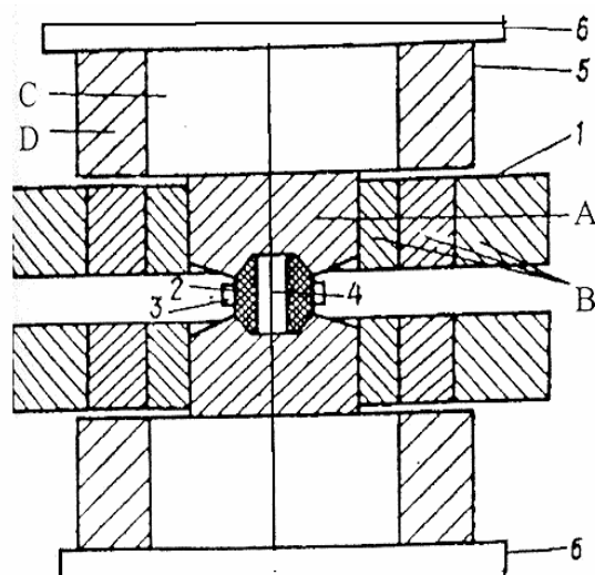
Figura 22 - Esquema do dispositivo Bigorna com concavidade. (1,5) Bloco de apoio (2) Cápsula deformável (3) Anel de formação da gaxeta (4) Mistura reativa (6) Base da prensa (A) Bigorna (B, D) Anéis de apoio (C) Disco [Novikov et al. , 1991].
