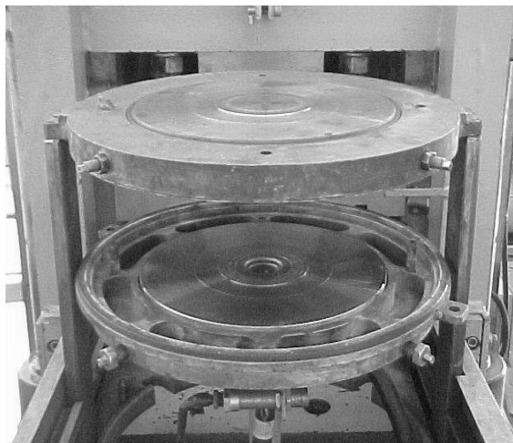
Figura 24 - DAP tipo Bigorna com concavidade.
