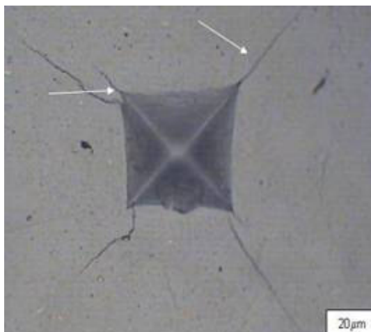
Figura 86 - Indentação na amostra C1 (convencional pura).
