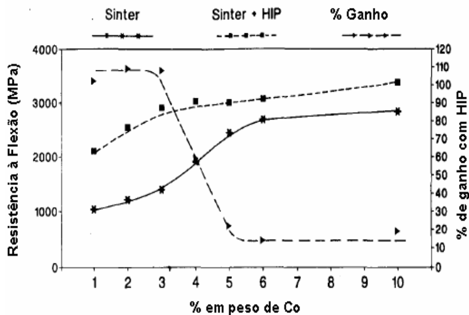
Figura 13 - Efeito do teor de Co no aumento da resistência à flexão por meio da sinter-HIP no metal duro [North et al. , 1991].
