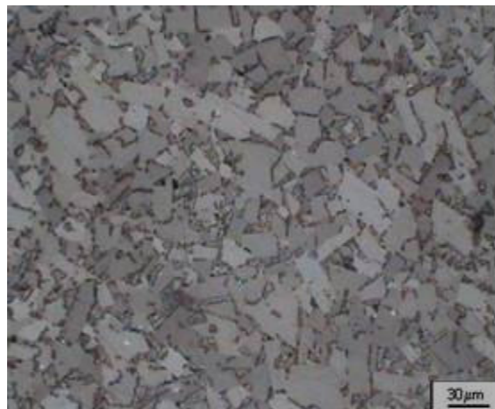
Figura 42 - Micrografia da amostra convencional dopada C2 - 250X.
