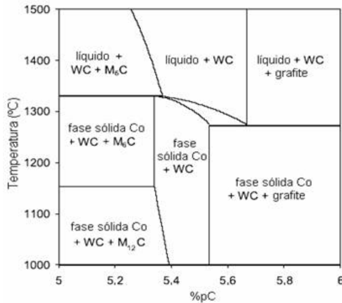
Figura 78 - Seção vertical de WC/10%pCo para uma razão atômica W/Co = 2,71 [Allibert, 2001].
