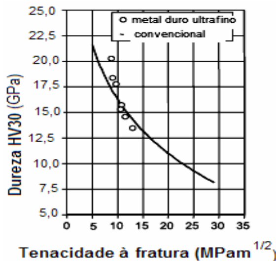
Figura 7 - Dureza e Tenacidade à Fratura do metal duro (WC/10%pCo) convencional e ultrafino [Gille et al. , 2002].
