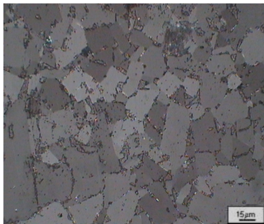
Figura 43 - Micrografia da amostra P1 (5GPa/1300°C/2min) - 400X.
