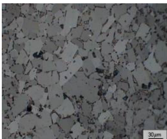
Figura 45 - Micrografia da amostra P6 (5GPa/1300°C/4min) - 250X.
