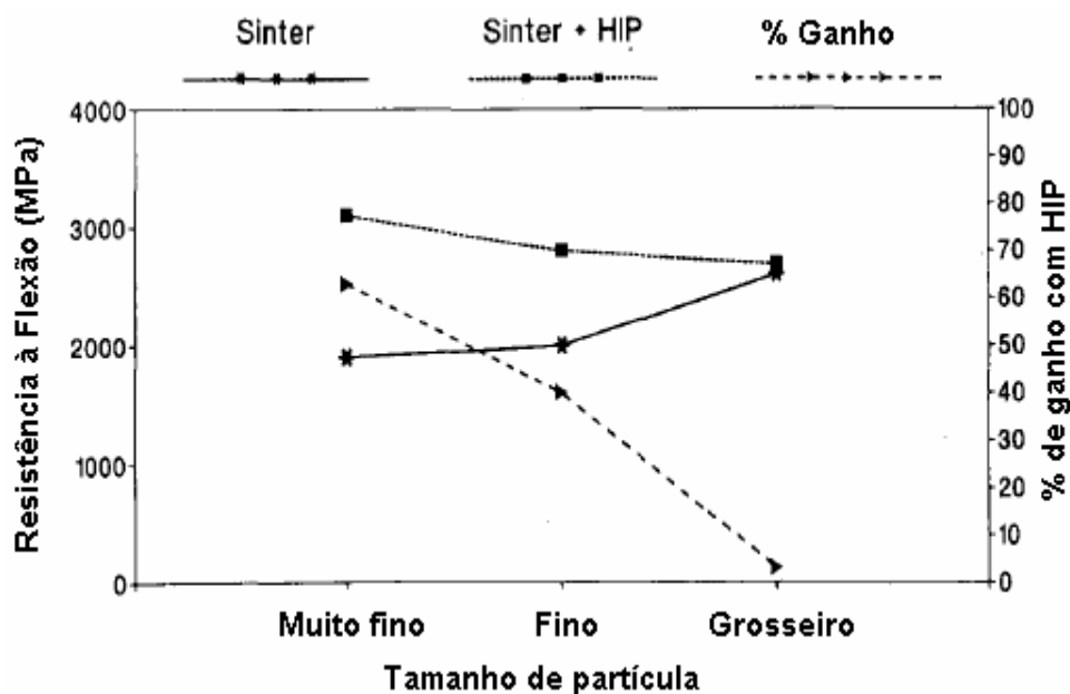
Figura 14 - Efeito do tamanho de grão no aumento da resistência à flexão por meio da sinter-HIP no metal duro [North et al. , 1991].
