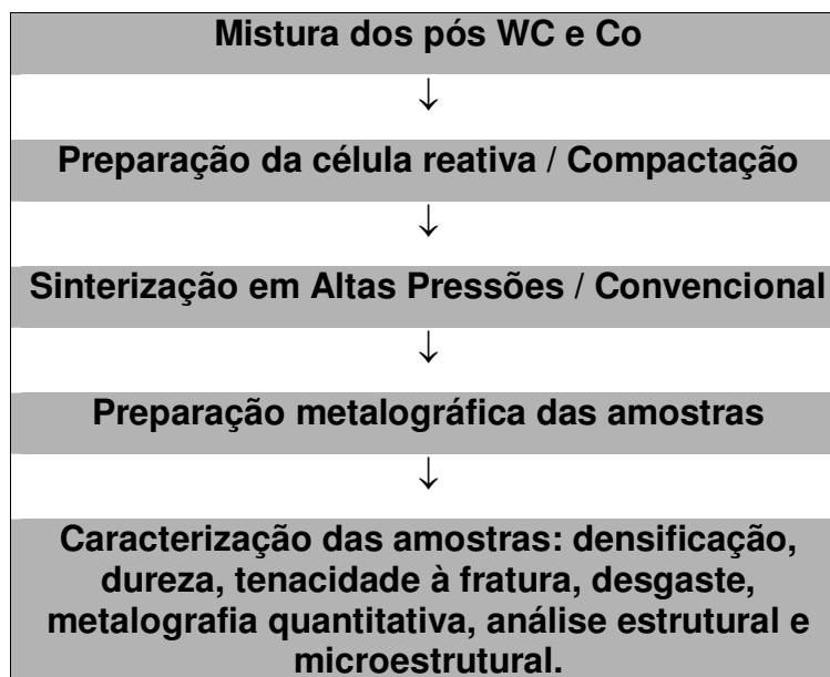
Figura 27 - Fluxograma da rota experimental neste trabalho.
