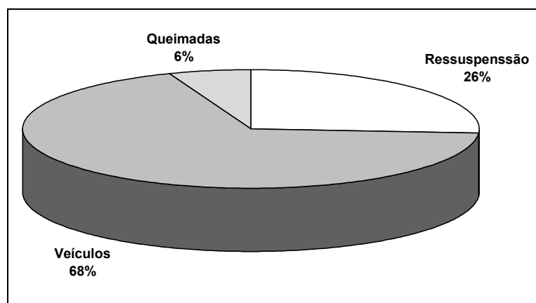
Figura 5.19: Contribuição de cada fonte para MP fino no período seco
