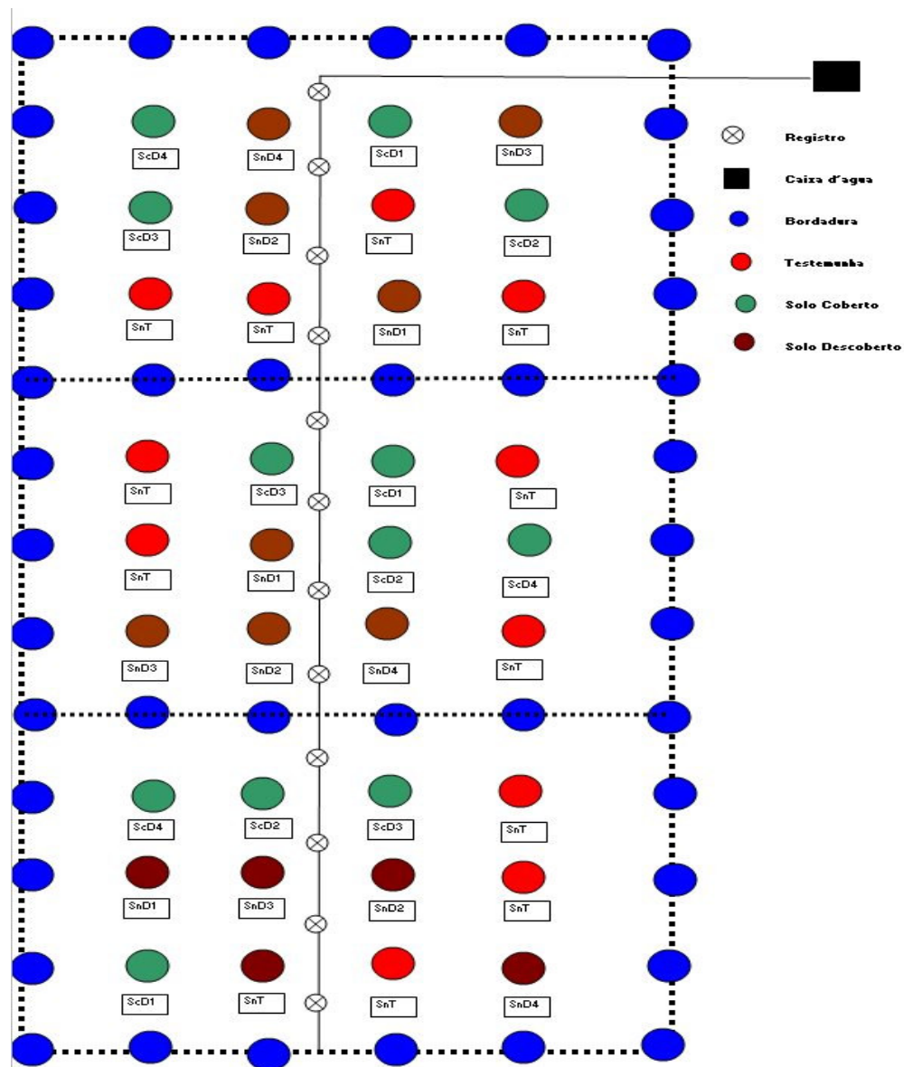
Figura 2. Layout da área do experimento.
