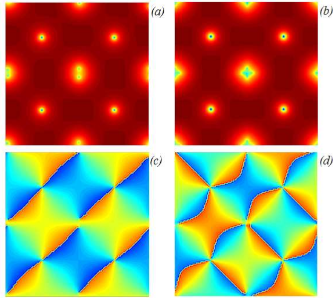
Figura 4.20: Logaritmo do módulo do parâmetro de ordem para uma célula de lados 32\xi(0) \times 32\xi(0) , T = 0.88T_c e d = 4\xi(0) , para (a) m = 10 , (b) m = 13 . Mudança na fase do parâmetro de ordem para os mesmos valores (c) m = 10 e (d) m = 13 .
