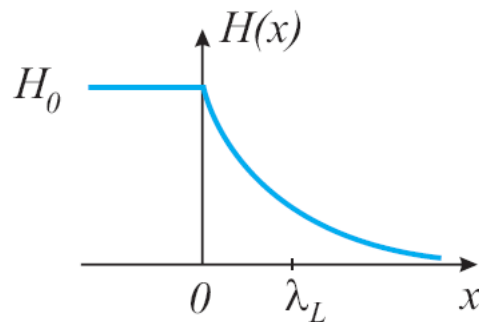
Figura 2.5: Penetração de campo magnético num supercondutor. O campo decresce a partir da superfície se tornando muito pequeno numa pequena profundidade \lambda_l .
