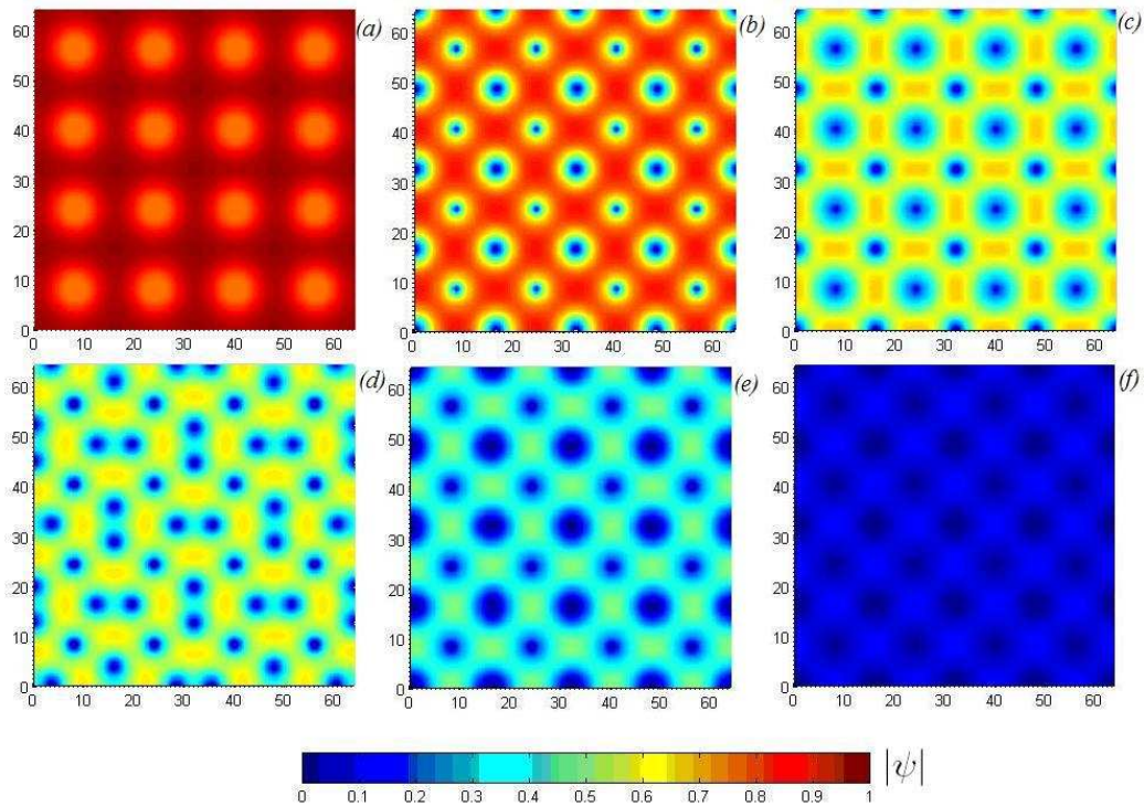
Figura 4.9: Módulo do parâmetro de ordem para uma célula unitária de lados 64\xi(0) \times 64\xi(0) , T = 0.9T_c e d = 6\xi(0) , para diferentes momentos magnéticos aplicados: (a) m = 30 , (b) m = 65 , (c) m = 90 , (d) m = 95 , (e) m = 115 , (f) m = 130 . Os cores indicam: Vermelho |\psi| = 1 , Azul |\psi| = 0 .
