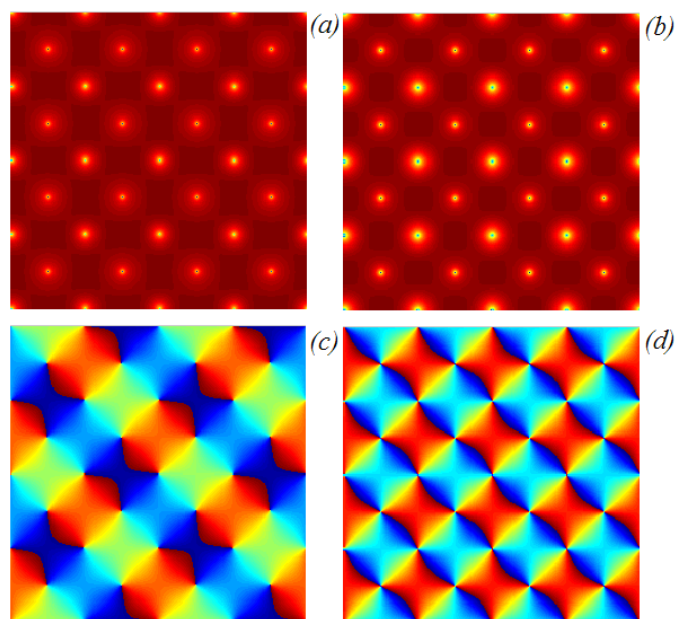
Figura 4.12: Logaritmo do módulo \psi para uma amostra de lados 64\xi(0) \times 64\xi(0) , T = 0.88T_c e d = 4\xi(0) , para (a) m = 7.5 e (b) m = 11.1 . Mudança na fase de \psi para os mesmos valores (c) m = 7.5 , (d) m = 11.1 .
