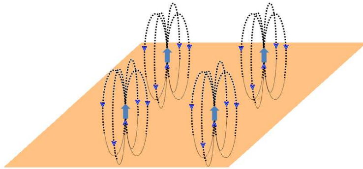
Figura 4.6: Rede de dipolos magnéticos acima de uma superfície supercondutora.
