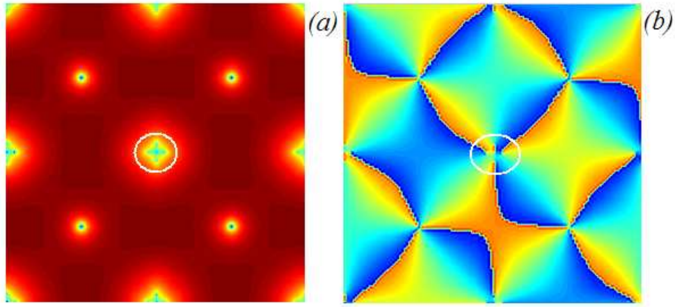
Figura 4.14: Ampliação do estado N = 4 ( m=12.9 ) da amostra de lados 64\xi(0) \times 64\xi(0) , T = 0.88T_c e d = 4\xi(0) . (a) Logaritmo de \psi (b) Mudança na fase de \psi .
