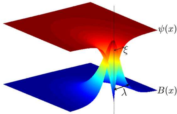
Figura 2.12: Campo magnético B(x) e parâmetro de ordem \psi(x) de uma linha de fluxo.
