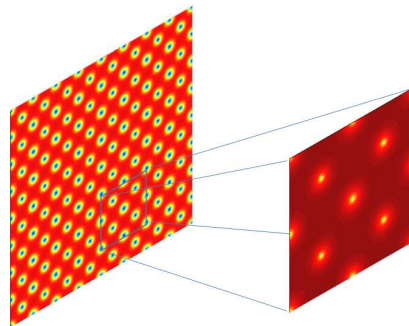
Figura 4.17: Região de análise para o estudo da nucleação de pares V-AV dependente da distância.
