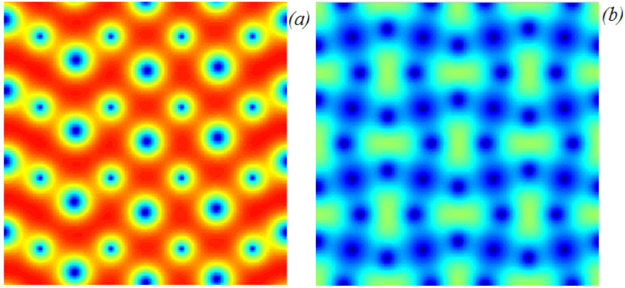
Figura 4.26: Configurações de pares de V-AV para os estados de transição em: (a) d = 1.8\xi(0) e m = 2.2 ; (b) d = 2.4\xi(0) e m = 5.6 ;
