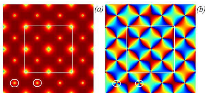
Figura 4.13: (a) Logaritmo do módulo \psi para o estado N = 4 ( m=12.9 ) da amostra de lados 64\xi(0) \times 64\xi(0) , T = 0.88T_c e d = 4\xi(0) . (b) Mudança na fase de \psi para o estado N = 4 da mesma amostra.
