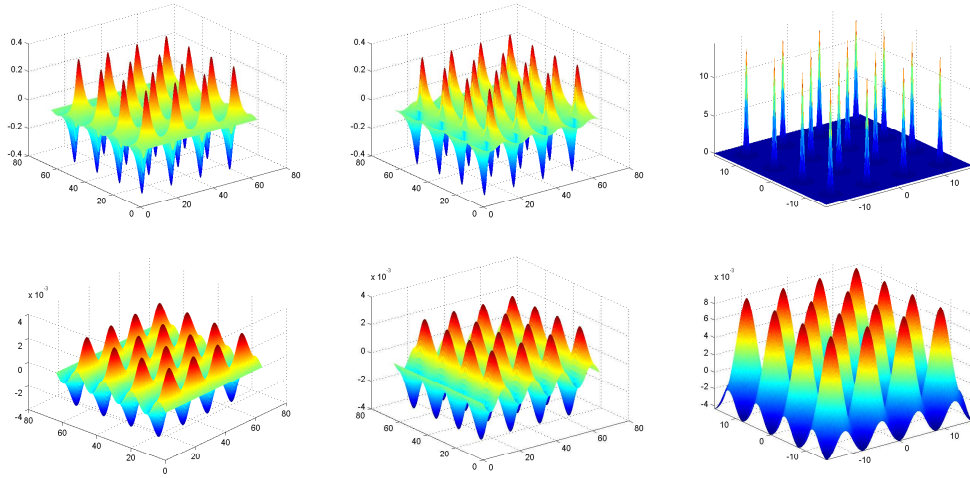
Figura 4.7: Acima Simulações para d = 1\xi(0) , Embaixo Simulações para d = 10\xi(0) esquerda Componente x do potencial vetor, centro Componente y do potencial vetor, direita Campo magnético.
