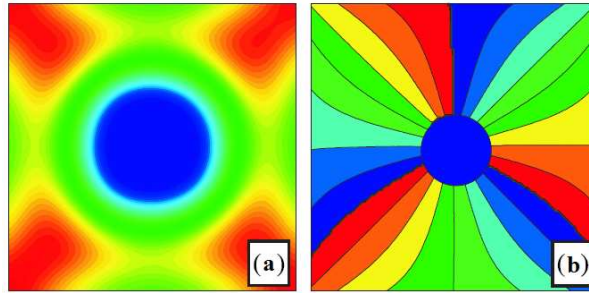
Figura 2.15: Estado de vórtice gigante em amostra quadrada com n = 3 , (a) Densidade de pares de Cooper, vermelho densidade alta, azul densidade baixa. (b) Mudança de 6\pi na fase SC [45].
