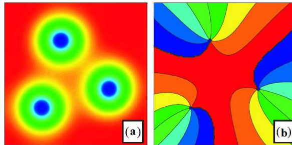
Figura 2.14: Estado de multi-vórtices numa amostra quadrada com vorticidade n = 3 , (a) Densidade de pares de Cooper, vermelho densidade alta, azul densidade baixa. (b) Mudança de 6\pi na fase SC [45].
