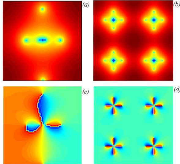
Figura 4.22: Logaritmo do módulo do parâmetro de ordem para uma célula de lados 32\xi(0) \times 32\xi(0) , T = 0.88T_c e d = 2\xi(0) , para (a) \vec{m} = 5 , (b) \vec{m} = 6 . Mudança na fase do parâmetro de ordem para os mesmos valores (c) \vec{m} = 5 e (d) \vec{m} = 6 .
