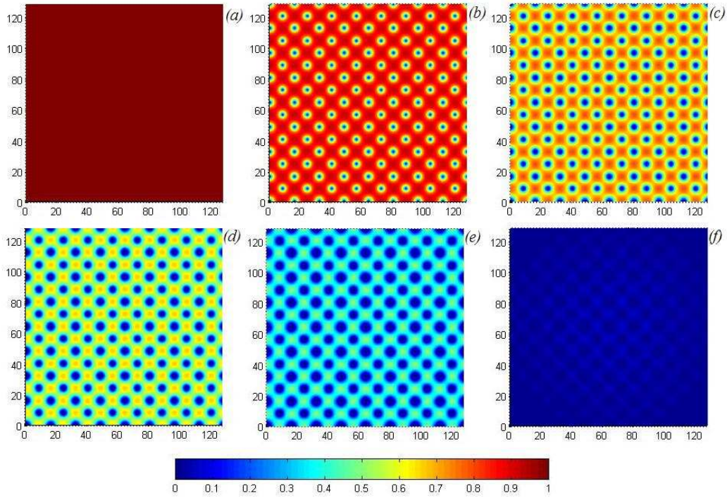
Figura 4.16: Módulo do parâmetro de ordem para uma célula unitária de lados 128\xi(0) \times 128\xi(0) , T = 0.88T_c e d = 12\xi(0) , para diferentes momentos magnéticos aplicados: (a) m = 0 , (b) m = 115 , (c) m = 240 , (d) m = 320 , (e) m = 380 , (f) m = 480 . A magnitude do parâmetro de ordem é dada pela barra de cores.
