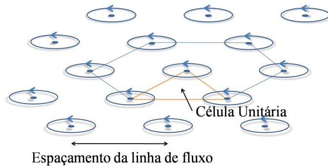
Figura 2.13: Rede Triangular de linhas de fluxo.
