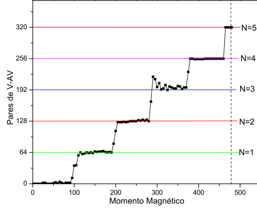
Figura 4.15: Número de pares de vórtice-antivórtice (V-AV) em função do momento magnético para uma amostra de 128\xi(0) \times 128\xi(0) para T = 0.88T_c e d = 12\xi(0) .
