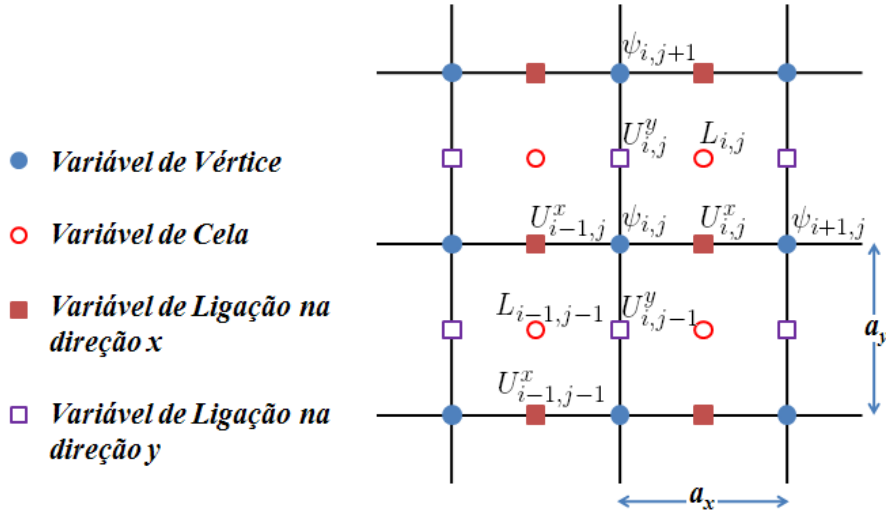
Figura 3.1: Esquema do método de variáveis de ligação.
