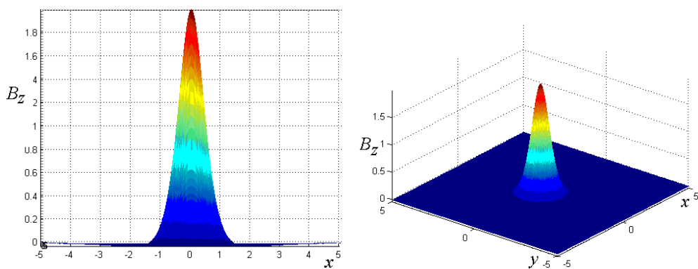
Figura 4.5: Componente z do campo magnético no plano xy devido ao dipolo magnético.
