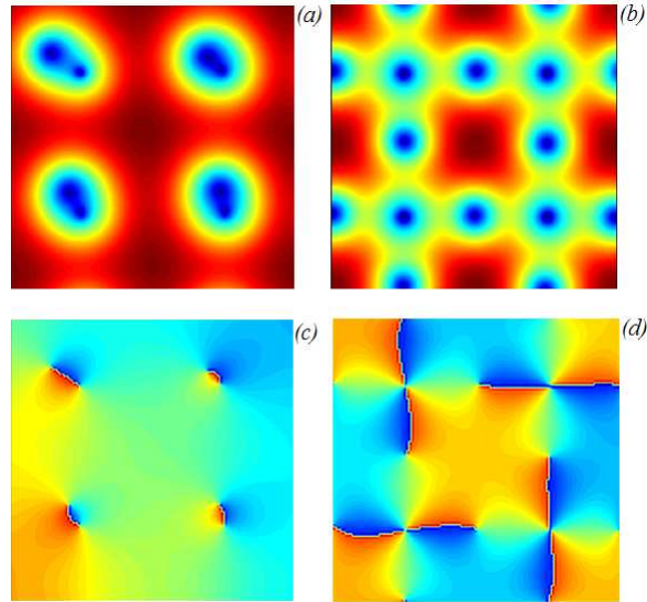
Figura 4.21: Módulo do parâmetro de ordem para uma célula de lados 32\xi(0) \times 32\xi(0) , T = 0.88T_c e d = 2\xi(0) , para (a) m = 2 , (b) m = 4 . Mudança na fase do parâmetro de ordem para os mesmos valores (c) m = 2 e (d) m = 4 .
