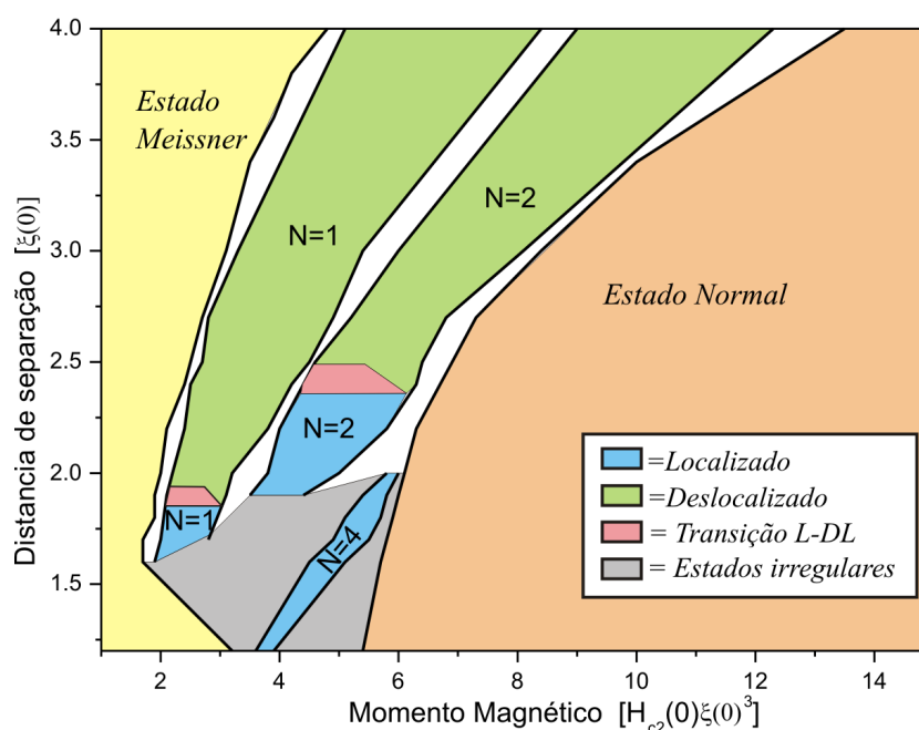
Figura 4.24: Diagrama de fases para os pares de V-AV numa amostra de 64\xi(0) \times 64\xi(0) com uma rede 4 \times 4 de dipolos magnéticos pontuais.
