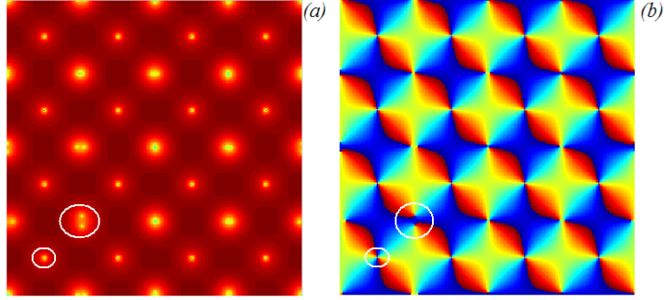
Figura 4.10: (a) Logaritmo do parâmetro de ordem (b) Mudança de fase, para uma célula unitária de lados 64\xi(0) \times 64\xi(0) , T = 0.9T_c e d = 6\xi(0) . Círculo menor Posição dos Vórtices, Círculo maior Posição dos Antivórtices.
