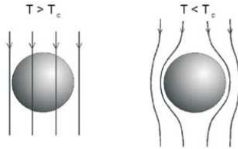
Figura 2.3: Efeito Meissner numa esfera supercondutora resfriada abaixo da temperatura crítica em um campo magnético constante. Embaixo da temperatura de transição as linhas de campo são expulsas da esfera.
