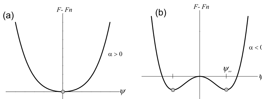
Figura 2.6: Funções da energia livre de Ginzburg-Landau para (a) T > T_c ( \alpha > 0 ) e para (b) T < T_c ( \alpha < 0 ). Os pontos indicam as posições de equilíbrio.
