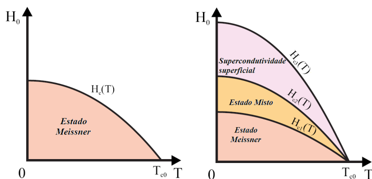
Figura 2.10: Diagrama de fase H - T para supercondutores tipo I (esquerda) e tipo-II (direita).
