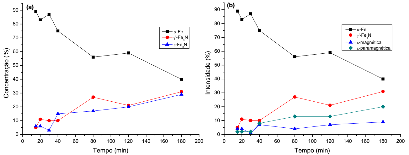
Figura 4.10: Gráfico da concentração das fases nitretadas em função do tempo da série CC. Na figura a) não é feita distinção entre a fase \epsilon magnética da fase \epsilon paramagnética e na figura b) as duas fases \epsilon estão separadas.
