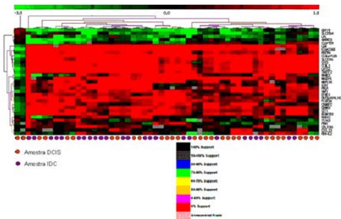
Figura 18 - A: Clusterização hierárquica com os 33 genes diferencialmente expressos entre DCIS e IDC (grupo pareado). B: Legenda do suporte do cluster avaliado pela técnica do Bootstrap .
