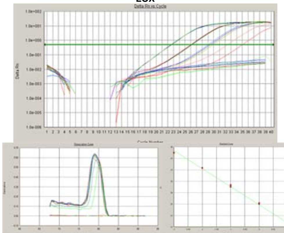
Figura 11 - Os gráficos de amplificação ( Amplification Plot ), especificidade da reação ( Dissociation curve ) e diluições de curva padrão respectivamente para os normalizadores GAPDH e HPRT1 e para os genes C16orf5 e LOX .
