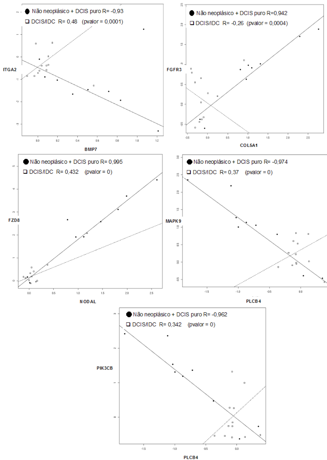
Figura 33 - Gráficos scatter-plot's para os pares de genes que apresentaram uma melhor clusterização das amostras ao longo das retas entre amostras não-neoplásica e DCIS puro versus DCIS/IDC.
