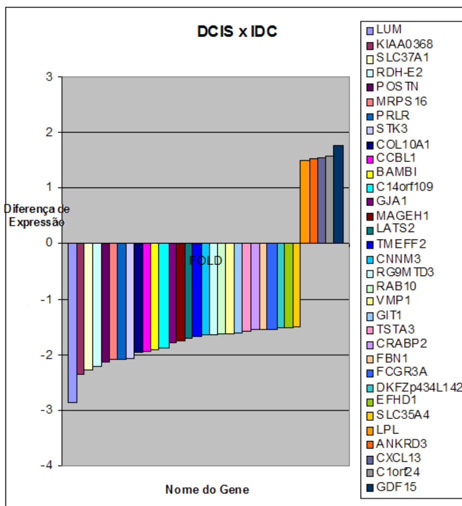
Figura 17 - Genes diferencialmente expressos na comparação entre DCIS e IDC coexistindo na mesma amostra ( fold > |1,5| e p < 0,01 ).
