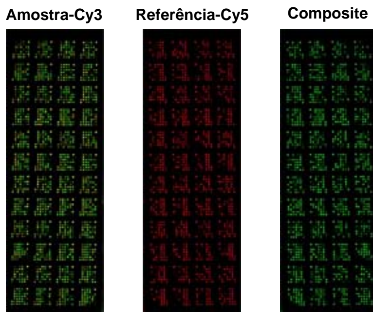
Figura 8 - Representação da lâmina contendo genes pertencentes às vias de sinalização WNT, PI3K e processo EMT hibridizada com amostra de carcinoma ductal in situ marcada com Cy3, referência com Cy5 e imagem sobreposta respectivamente.
