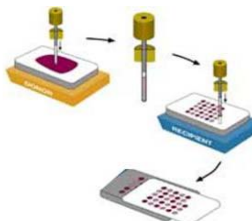
Figura 14 - Esquema mostrando a montagem do bloco do tissue microarray e a lâmina para a análise.
