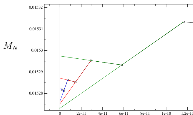
Figuras 19: Mostramos nesta figura a magnetização para tamanhos naturais, usando a seqüência de Rudin-Shapiro no modelo de Ising com r = 1 e K_A = 0,71 .
