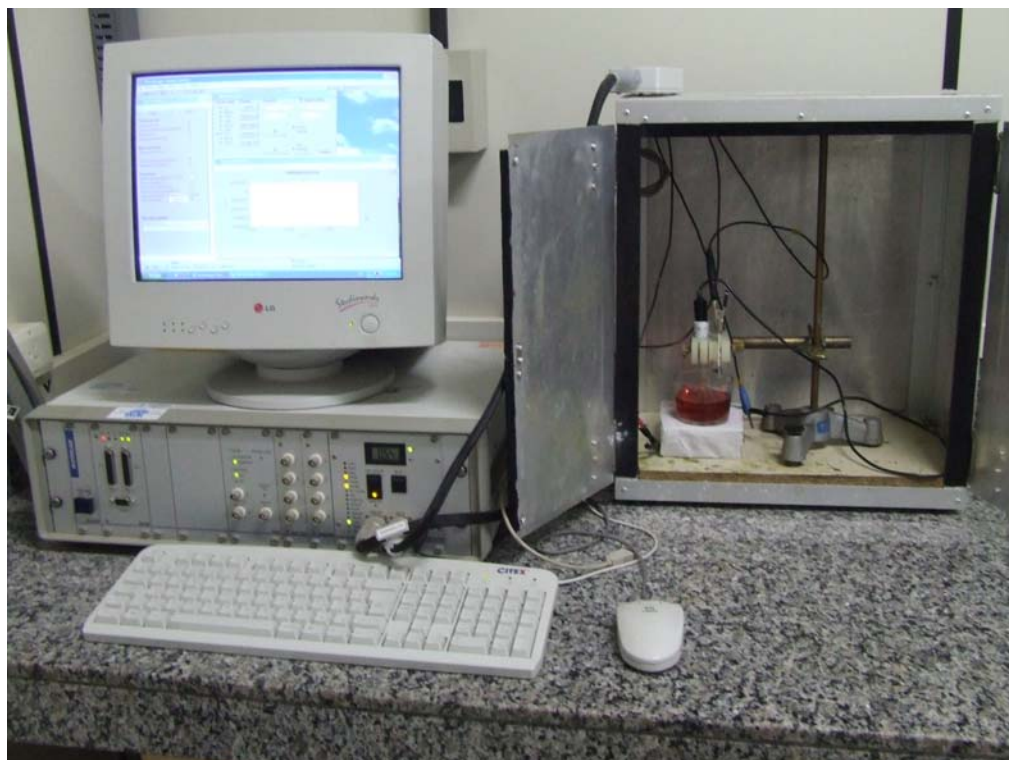
Figura II.2: Foto do aparato experimental utilizado nos experimentos eletroquímicos. Nela temos uma célula eletroquímica de três eletrodos colocada dentro de uma caixa de alumínio. A célula eletroquímica esta conectada a um potenciostato, interfaceado com um microcomputador.
