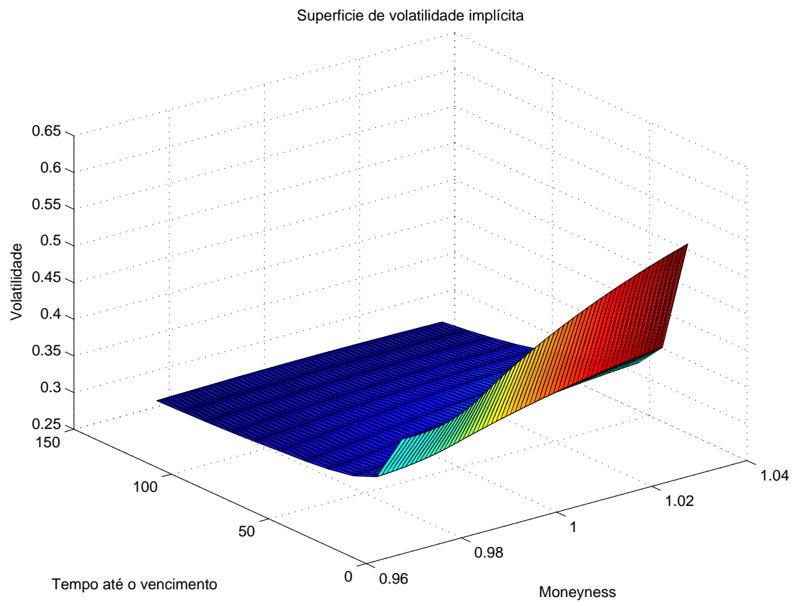
Figura 6.4: Superfície de volatilidade implícita para opções sobre o IBOVESPA, no dia 04/02/2005, com o índice IBOVESPA cotado a 24548.18
