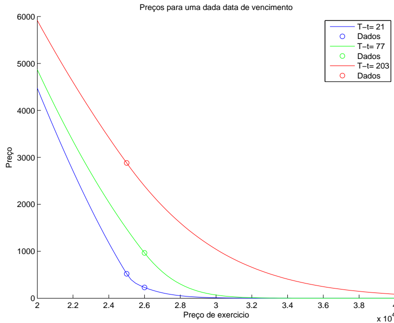
Figura 6.1: Curva de preços para opções no dia 24/01/2005, com o índice IBOVESPA cotado a 23812.51
