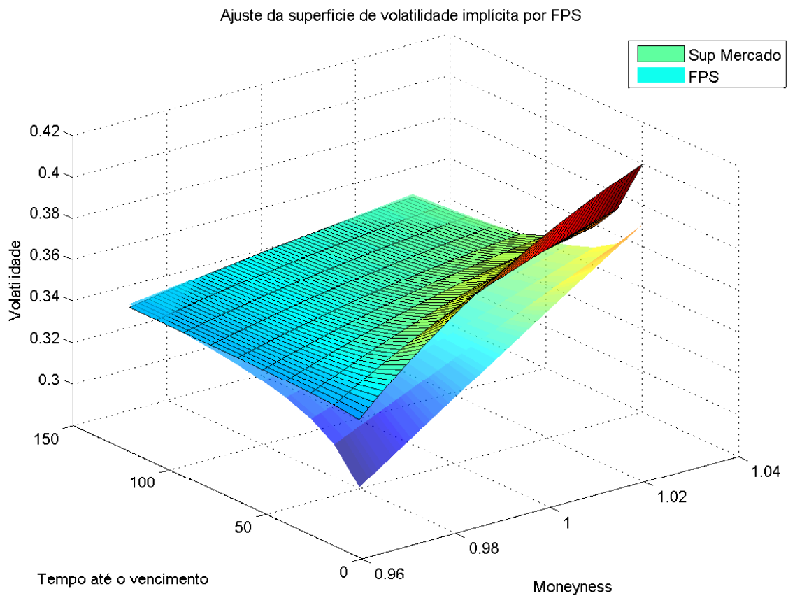
Figura 7.2: Ajuste da superfície de volatilidade implícita do mercado pela superfície estimada segundo FPS, no dia 11/04/2006, com o índice IBOVESPA cotado a 37823.02
