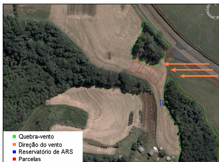
Figura 14: Influência do vento na uniformidade de distribuição.
