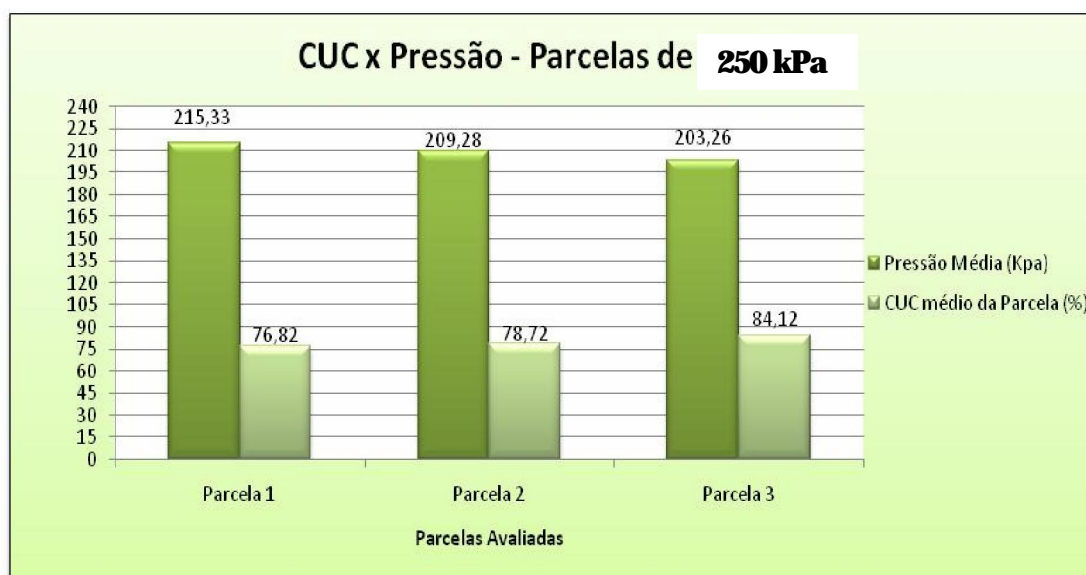
Figura 19: Valores médios de CUC em função da pressão média dos aspersores correspondentes às parcelas avaliadas para 250 kPa.
