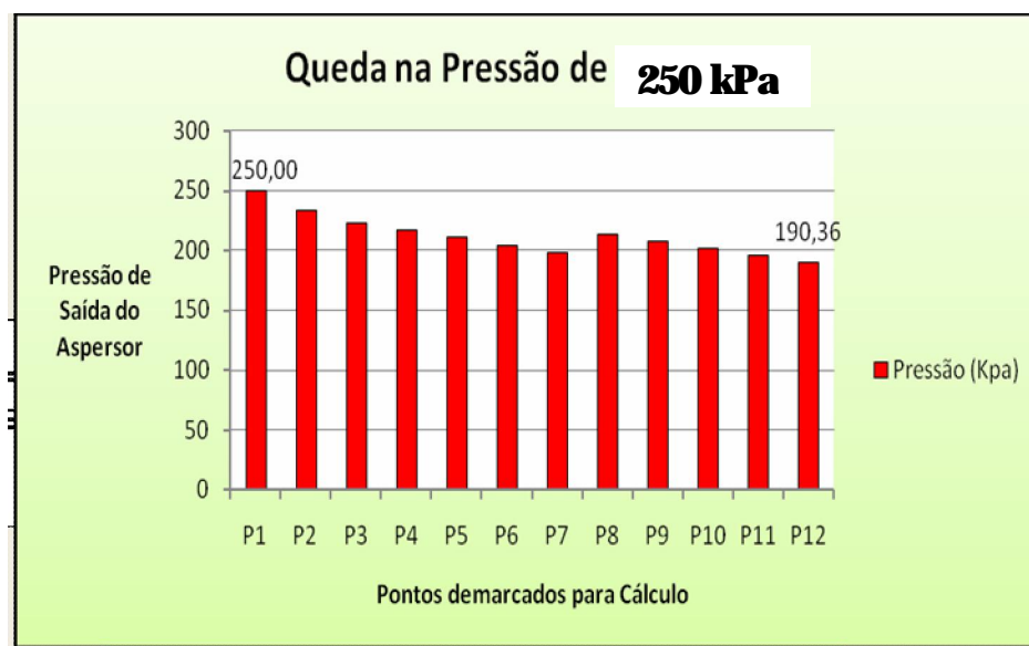
Figura 18: Redução da pressão ao longo das linhas principais e laterais para 250 kPa.
