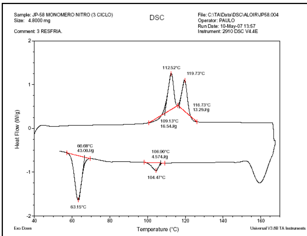
(DSC). Termograma do composto 38a - 3º Ciclo (10°C/min)
