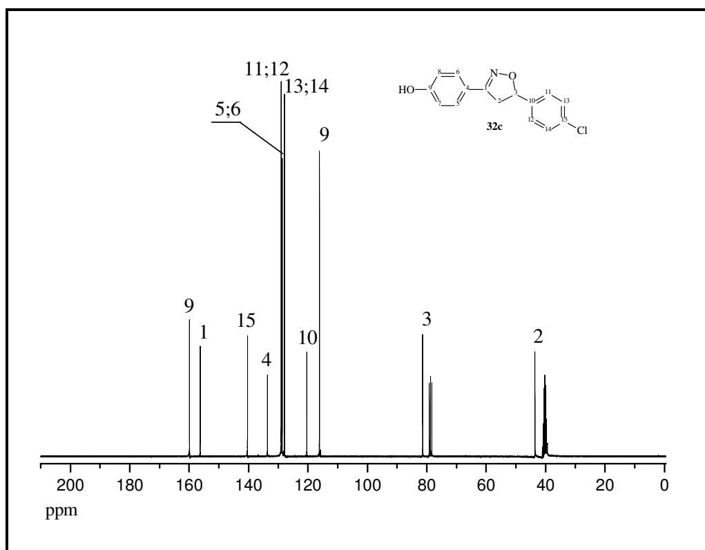
Espectro de RMN 13 C (CDCl 3 /DMSO d6 ), 75 MHz do composto 32c
