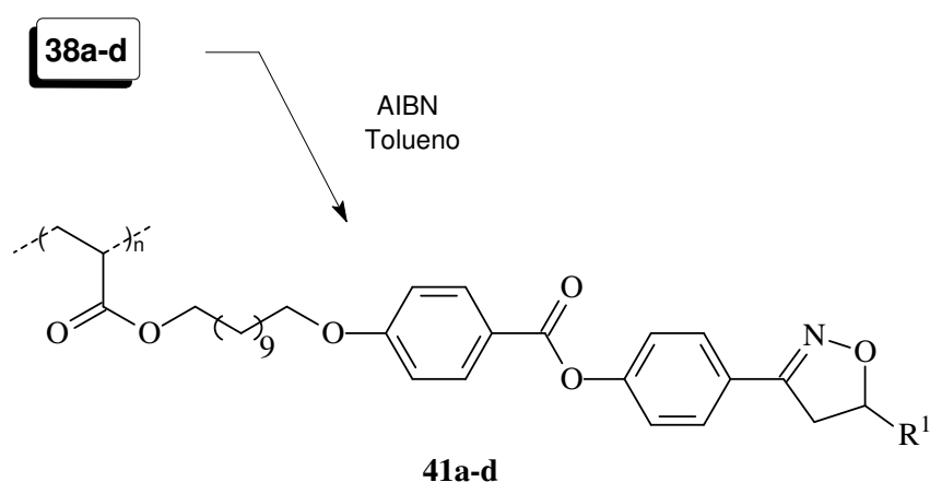
Esquema 19: Síntese dos Polímeros 41a-d .
