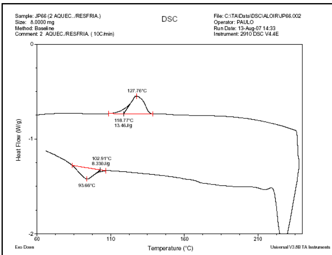
(DSC). Termograma do composto 41c - 2° Ciclo (10°C/min)
