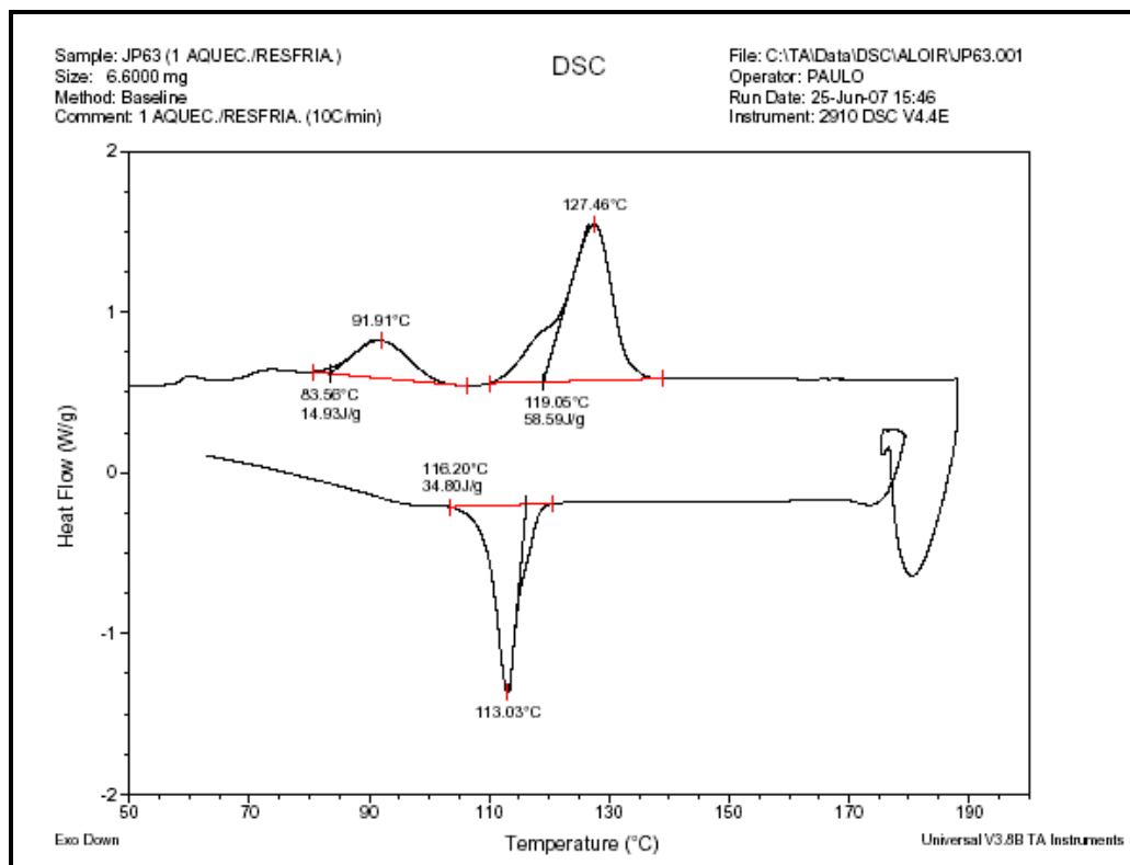
(DSC). Termograma do composto 38b - 1º Ciclo (10°C/min)
