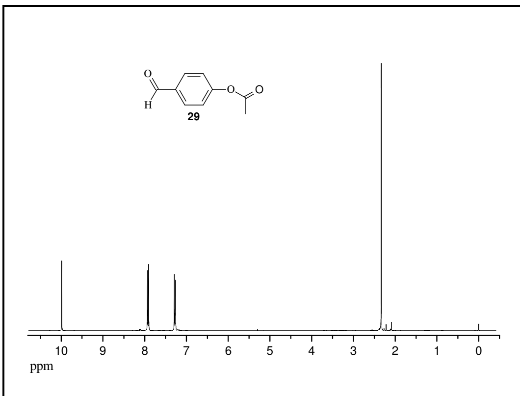
Espectro de RMN ^1\text{H} (CDCl 3 ), 300 MHz do composto 29
