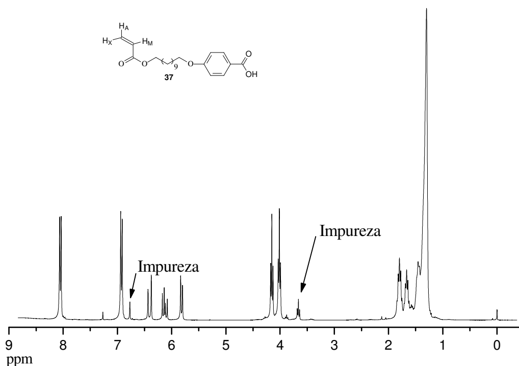
Figura 26. Espectro de RMN ^1\text{H} (300 MHz, \text{CDCl}_3 ) do ácido 37
