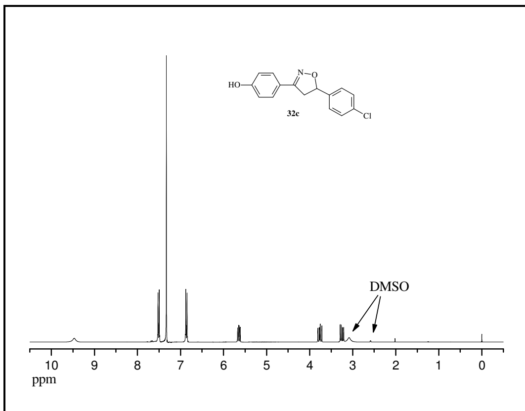
Espectro de RMN 1 H (CDCl 3 /DMSO d6 ), 300 MHz do composto 32c
