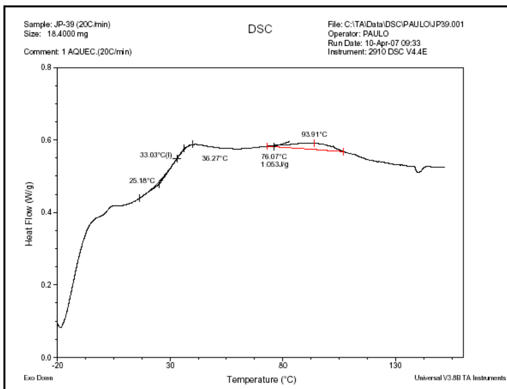
(DSC). Termograma do composto 41d - 1° Ciclo: Aquecimento (20°C/min)
