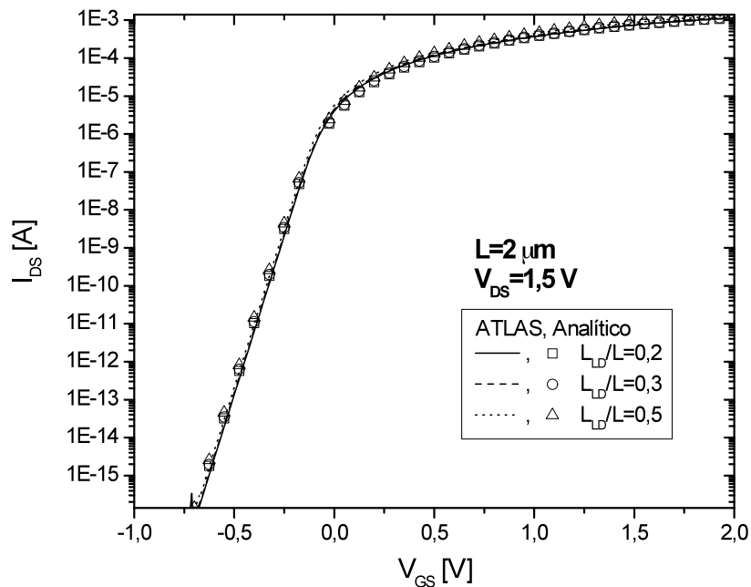
Figura 4.34 - Característica I_{DS} \times V_{GS} em sublimar com V_{DS}=1,5 V, para L = 2 \mu\text{m} .
