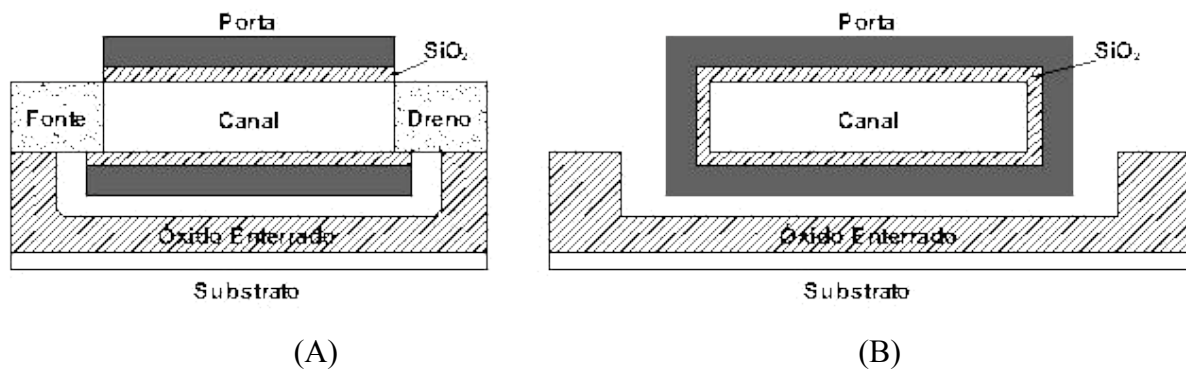
(A) (B) Figura 2.1 – Dispositivo GAA: vista frontal (A) e lateral (B).
