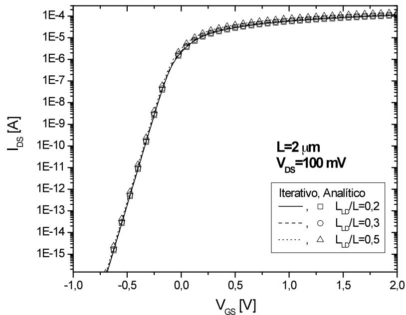
Figura 4.10 - Característica I_{DS} \times V_{GS} em sublimiar com V_{DS} = 100 \text{ mV} , para L = 2 \mu\text{m} .
