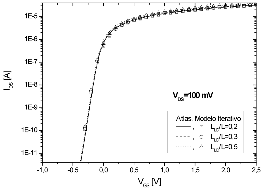
Figura 3.4 - Característica I_{DS} \times V_{GS} em sublimiar com V_{DS} = 100 \text{ mV}
