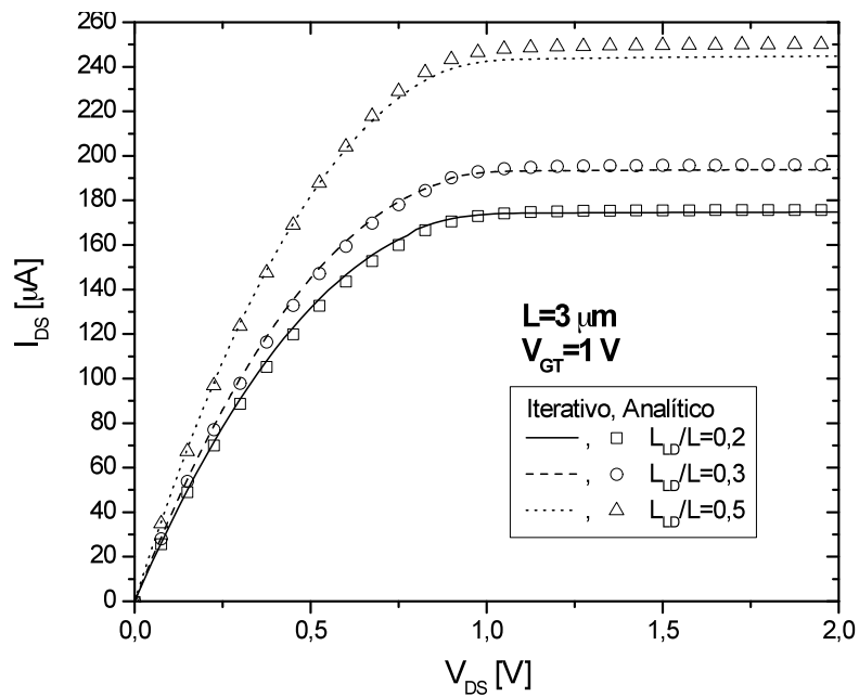
Figura 4.21 - Característica I_{DS} \times V_{DS} com sobretensão V_{GT}=1 V, para L = 3 \mu\text{m} .
