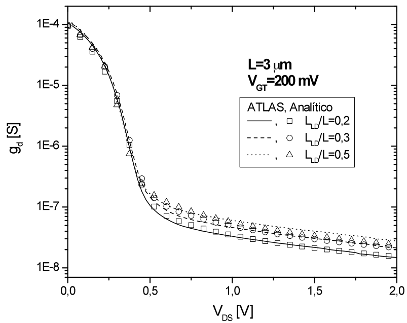
Figura 4.48 - Condutância g_d \times V_{DS} com V_{GT}=200 mV, para L = 3 \mu\text{m} .
