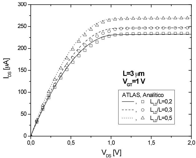
Figura 4.45 - Característica I_{DS} \times V_{DS} com sobre-tensão V_{GT}=1 V, para L = 3 \mu\text{m} .
