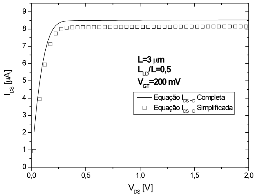
Figura 4.1 – Comparação da característica I_{DS} \times V_{DS} para simplificação na equação de I_{DS,HD}
