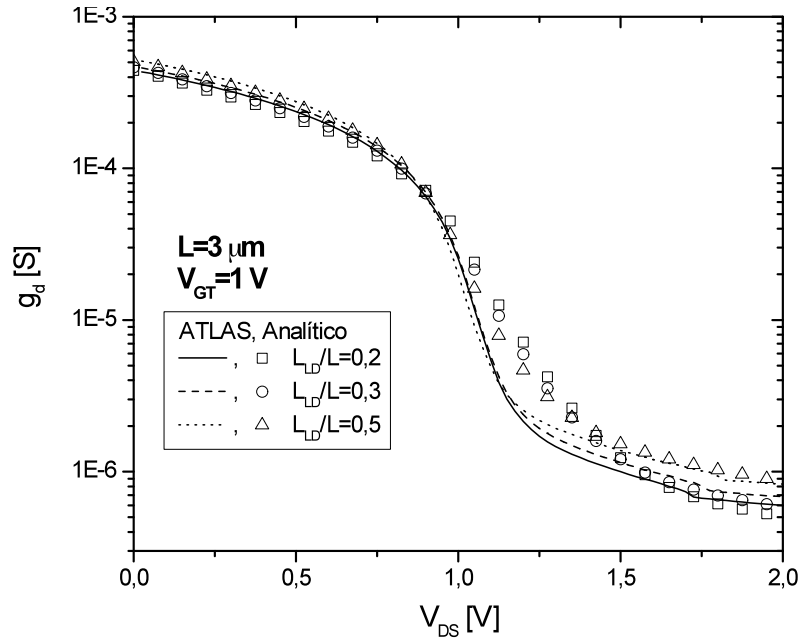
Figura 4.51 - Condutância g_d \times V_{DS} com V_{GT}=1 V, para L = 3 \mu\text{m} .
