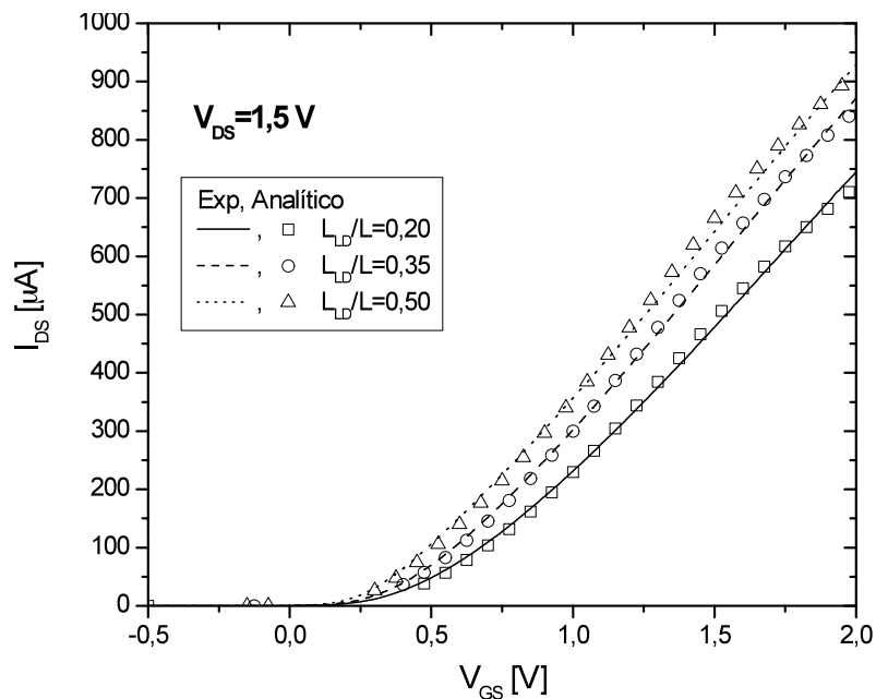
Figura 4.55 - Característica I_{DS} \times V_{GS} com V_{DS}=1,5 V.
