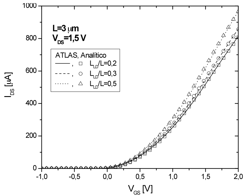
Figura 4.30 - Característica I_{DS} \times V_{GS} com V_{DS}=1,5 V, para L = 3 \mu\text{m} .
