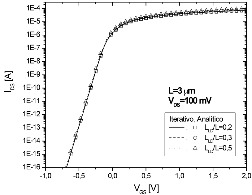
Figura 4.9 - Característica I_{DS} \times V_{GS} em sublimiar com V_{DS} = 100 \text{ mV} , para L = 3 \mu\text{m} .
