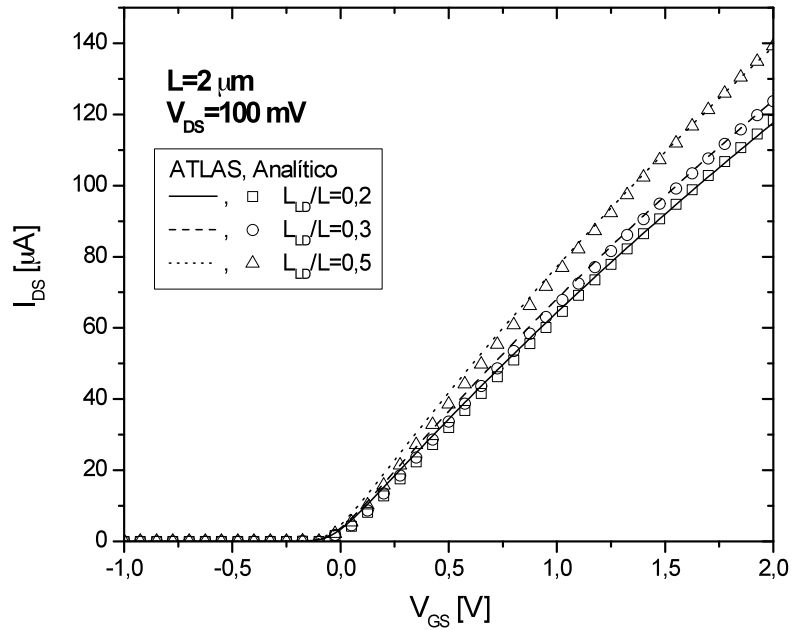
Figura 4.25 - Característica I_{DS} \times V_{GS} com V_{DS} = 100 \text{ mV} , para L = 2 \mu\text{m} .
