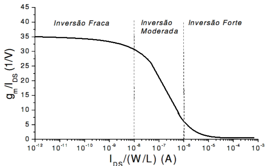
Figura 2.8 - Representação esquemática para relação g_m/I_{DS} para transistores SOI MOS.
