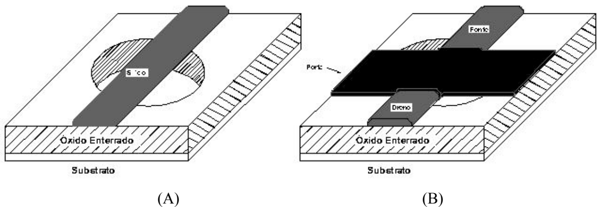
Figura 2.3 - Perspectiva da lâmina: após a corrosão da cavidade (A), e após definição de fonte e dreno (B).
