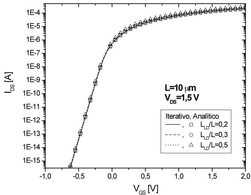
Figura 4.14 - Característica I_{DS} \times V_{GS} em sublimiar com V_{DS}=1,5 V, para L = 10 \mu\text{m} .
