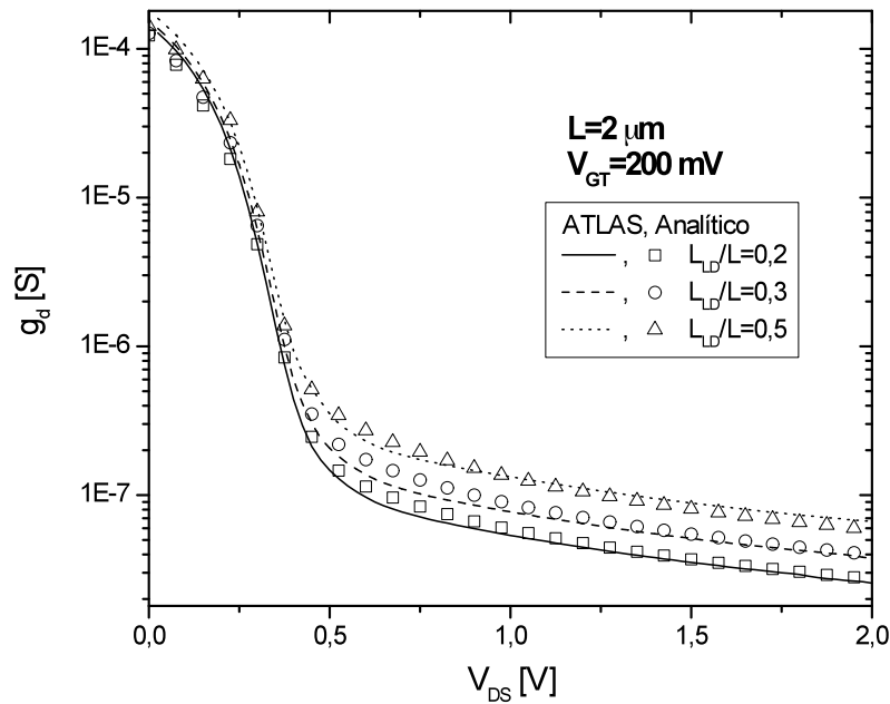
Figura 4.49 - Condutância g_d \times V_{DS} com V_{GT}=200 mV, para L = 2 \mu\text{m} .
