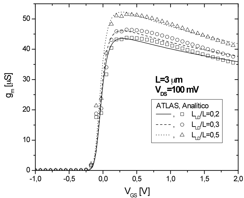
Figura 4.36 - Transcondutância g_m \times V_{GS} com V_{DS}=100 mV, para L = 3 \mu\text{m} .
