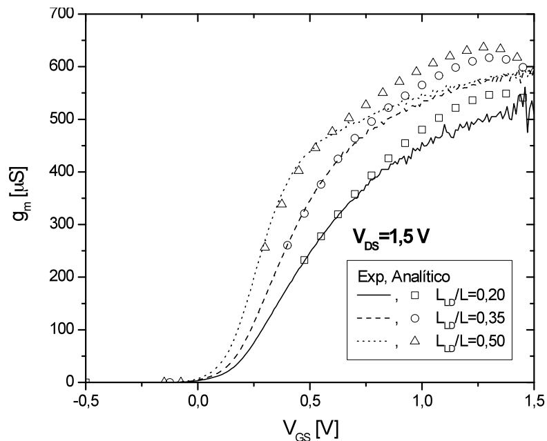
Figura 4.57 - Transcondutância g_m \times V_{GS} com V_{DS}=1,5\text{ V} .
