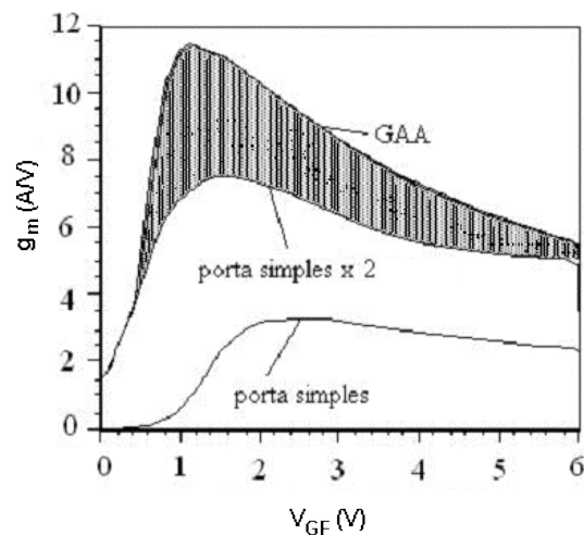
Figura 2.4 - Transcondutância em função da tensão de porta com V_{DS}=100\text{mV} para um transistor SOI de porta simples e um GAA [5].
