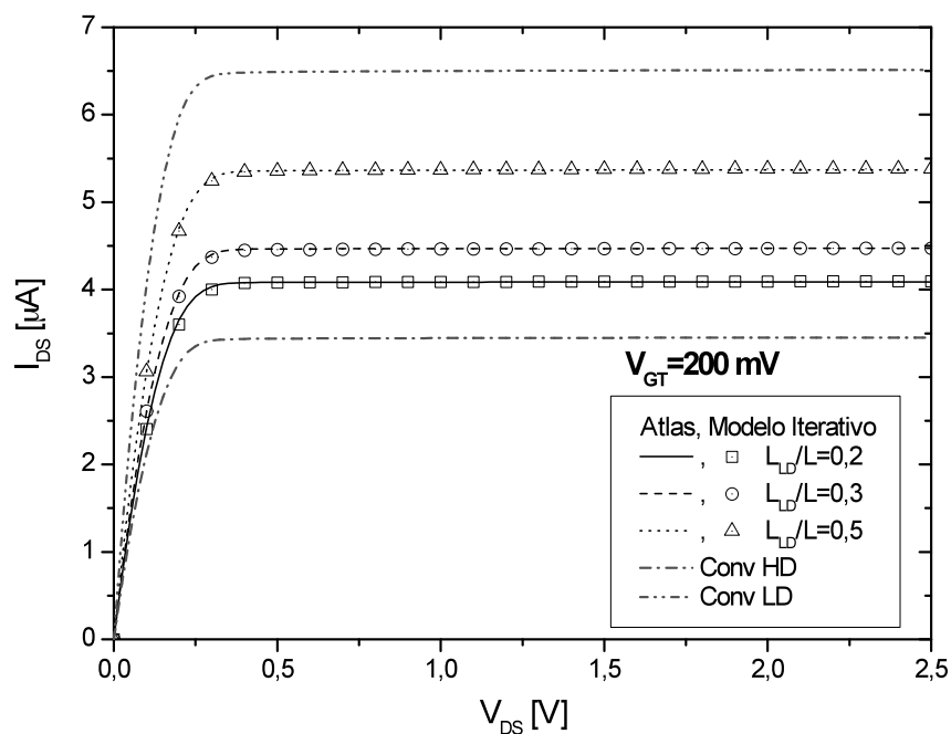
Figura 3.6 - Característica I_{DS} \times V_{DS} com sobre-tensão V_{GT}=200 mV
