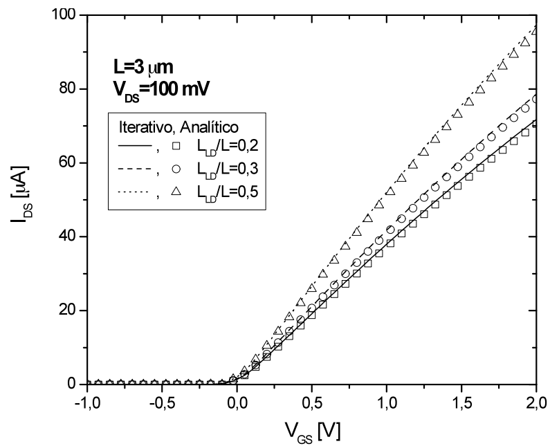
Figura 4.6 - Característica I DS xV GS com V DS =100 mV, para L = 3 \mu\text{m} .
