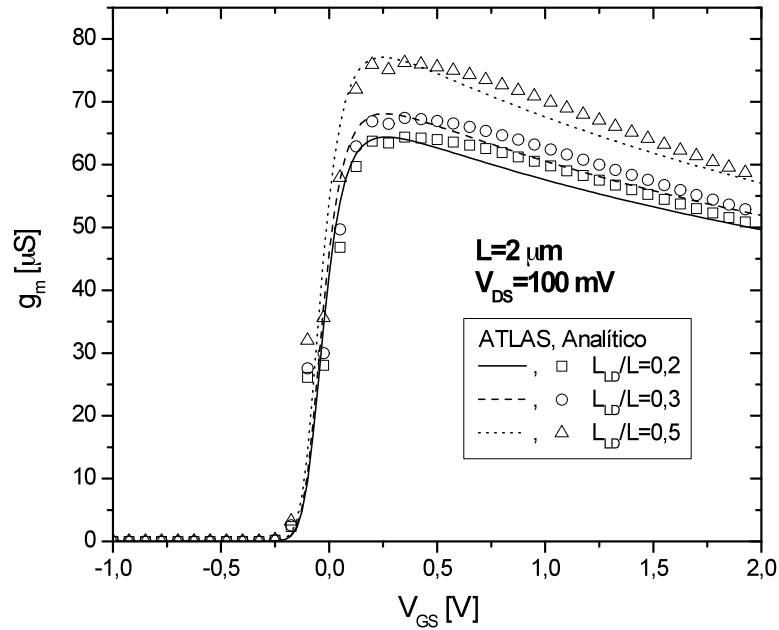
Figura 4.37 - Transcondutância g_m \times V_{GS} com V_{DS}=100 mV, para L = 2 \mu\text{m} .
