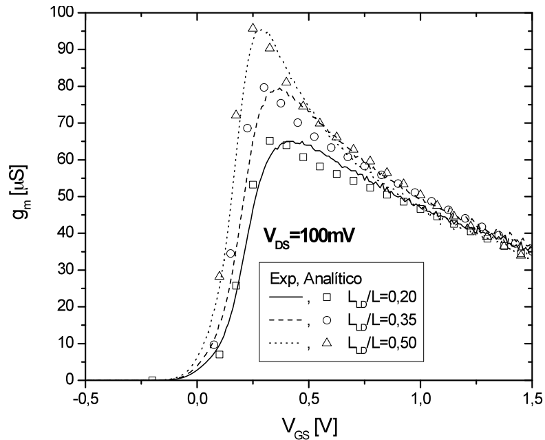
Figura 4.56 - Transcondutância g_m \times V_{GS} com V_{DS}=100\text{ mV} .
