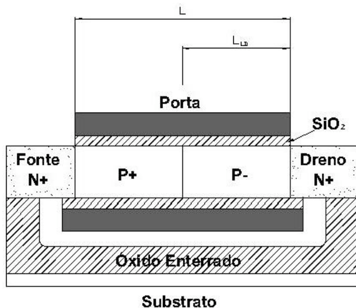
Figura 2.6 - Perfil transversal do transistor GAA SOI MOSFET canal n totalmente depletado com perfil de dopantes assimétrico na região de canal (GC GAA SOI nMOSFET).
