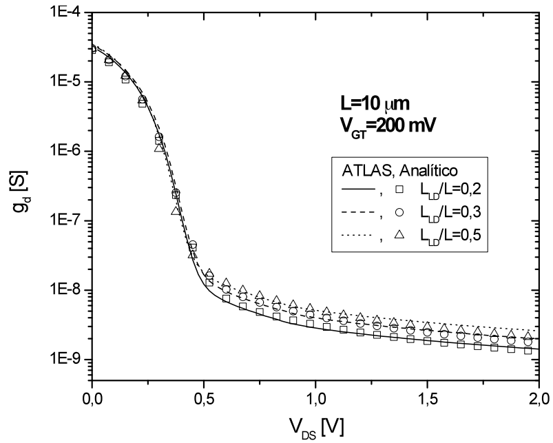
Figura 4.47 - Condutância g_d \times V_{DS} com V_{GT}=200 mV, para L = 10 \mu\text{m} .
