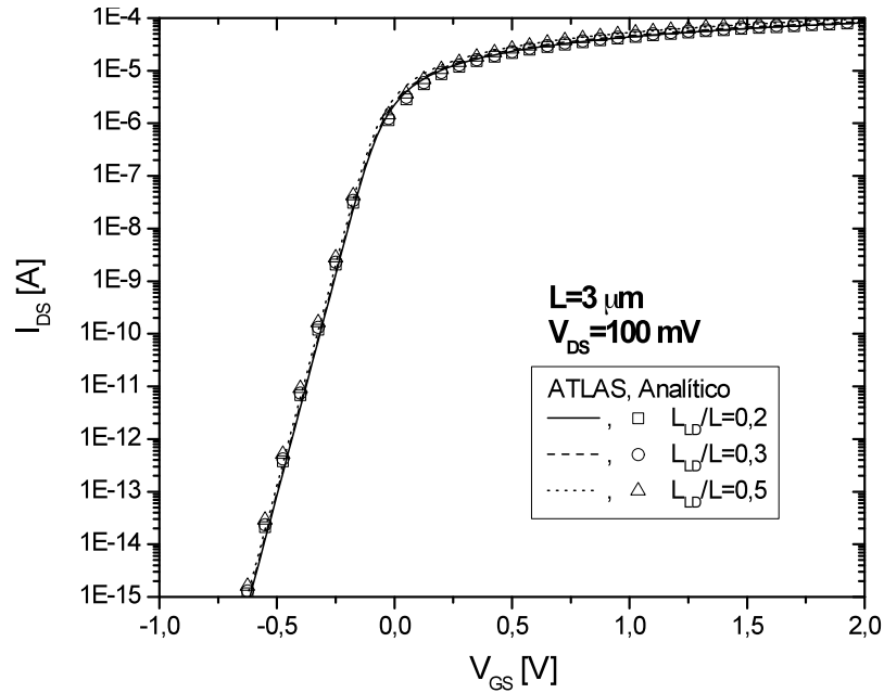
Figura 4.27 - Característica I_{DS} \times V_{GS} em sublimiar com V_{DS}=100 mV, para L = 3 \mu\text{m} .
