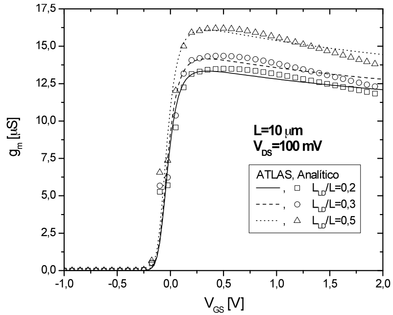
Figura 4.35 - Transcondutância g_m \times V_{GS} com V_{DS}=100 mV, para L = 10 \mu\text{m} .
