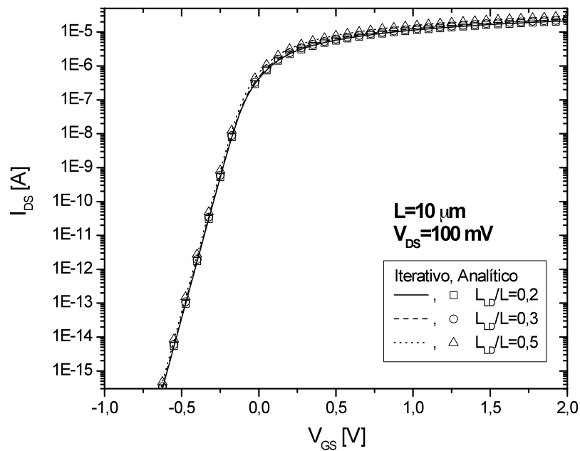
Figura 4.8 - Característica I_{DS} \times V_{GS} em sublimiar com V_{DS} = 100 \text{ mV} , para L = 10 \mu\text{m} .
