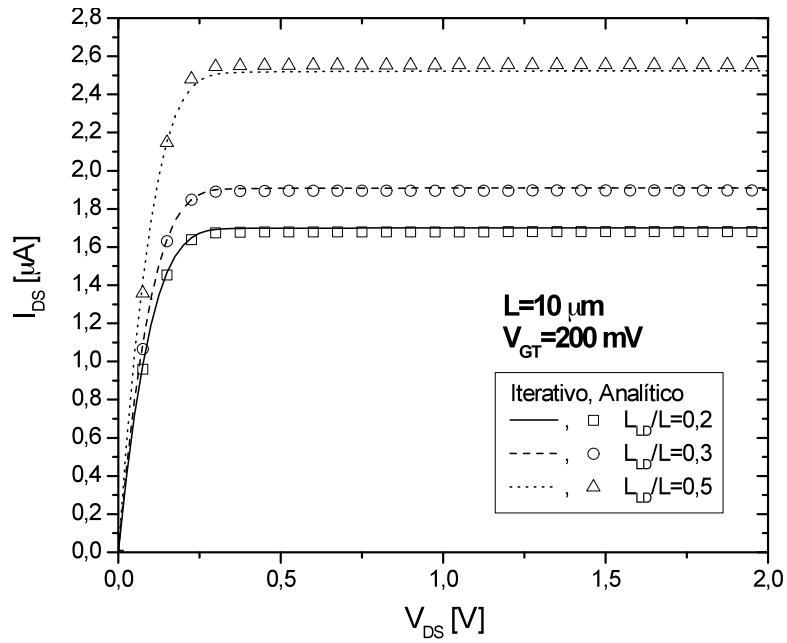
Figura 4.17 - Característica I_{DS} \times V_{DS} com sobretensão V_{GT}=200 \text{ mV} , para L = 10 \mu\text{m} .
