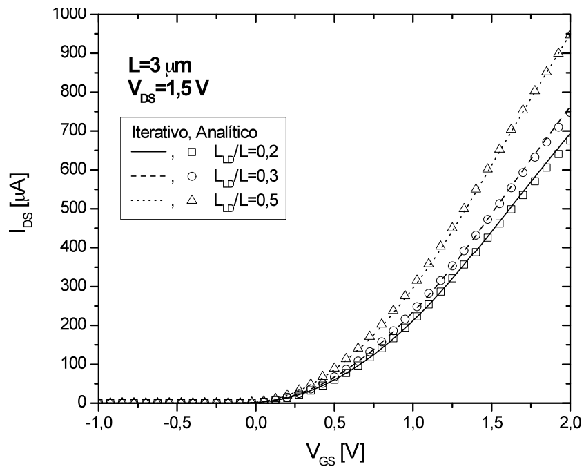
Figura 4.12 - Característica I_{DS} \times V_{GS} com V_{DS}=1,5 V, para L = 3 \mu\text{m} .
