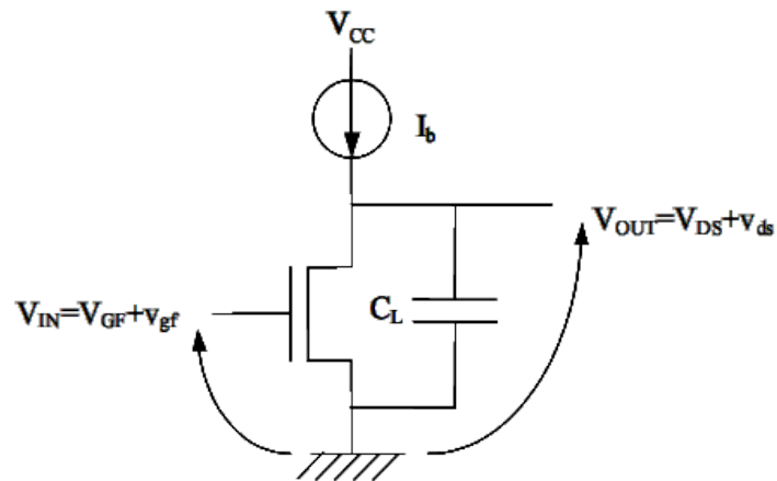
Figura 2.7 - Amplificador de tensão com um único transistor MOS.
