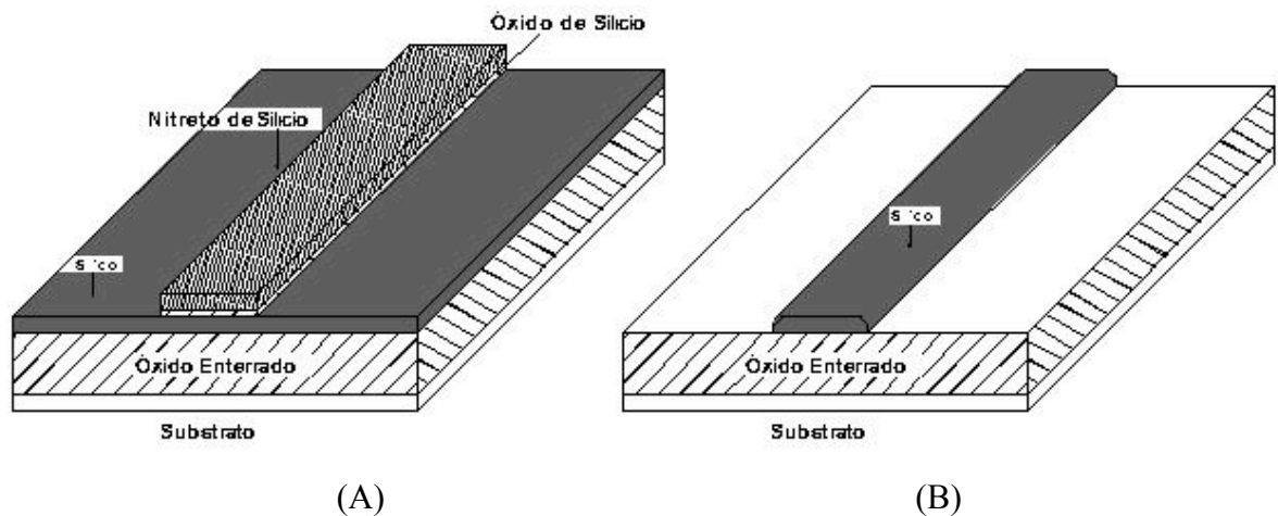
Figura 2.2 - Perspectiva da lâmina: após a definição da região ativa (A), e após o arredondamento dos cantos (B).
