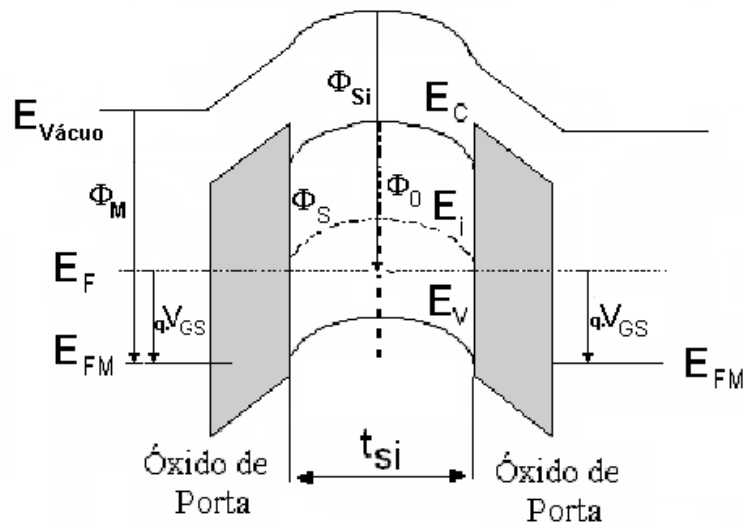
Figura 2.10 - Diagrama de faixas de energia do transistor DG.
