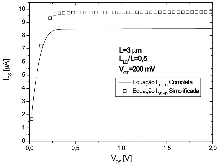
Figura 4.2 - Comparação da característica I_{DS} \times V_{DS} para simplificação na equação de Q_{D,HD}
