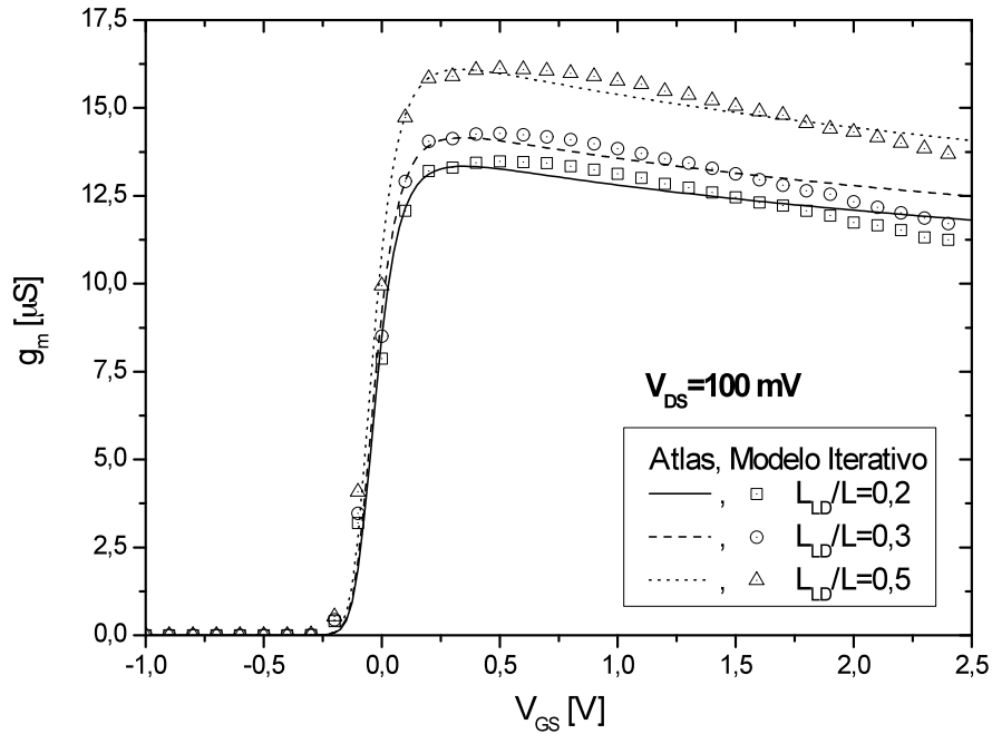
Figura 3.8 - Transcondutância g_m \times V_{GS} com V_{DS}=100 \text{ mV}
