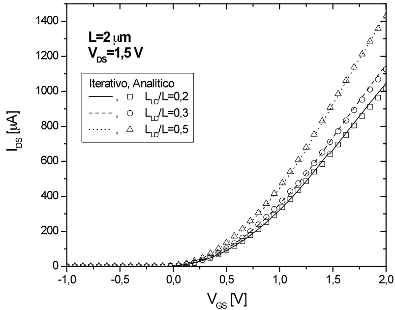
Figura 4.13 - Característica I_{DS} \times V_{GS} com V_{DS}=1,5 V, para L = 2 \mu\text{m} .
