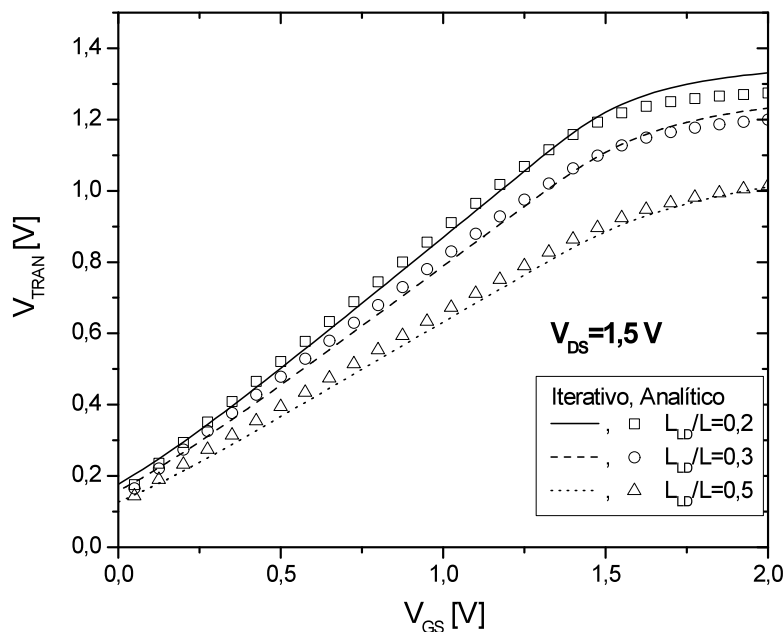
Figura 4.3 - Tensão de transição pela tensão de porta com V_{DS}=1,5 V.
