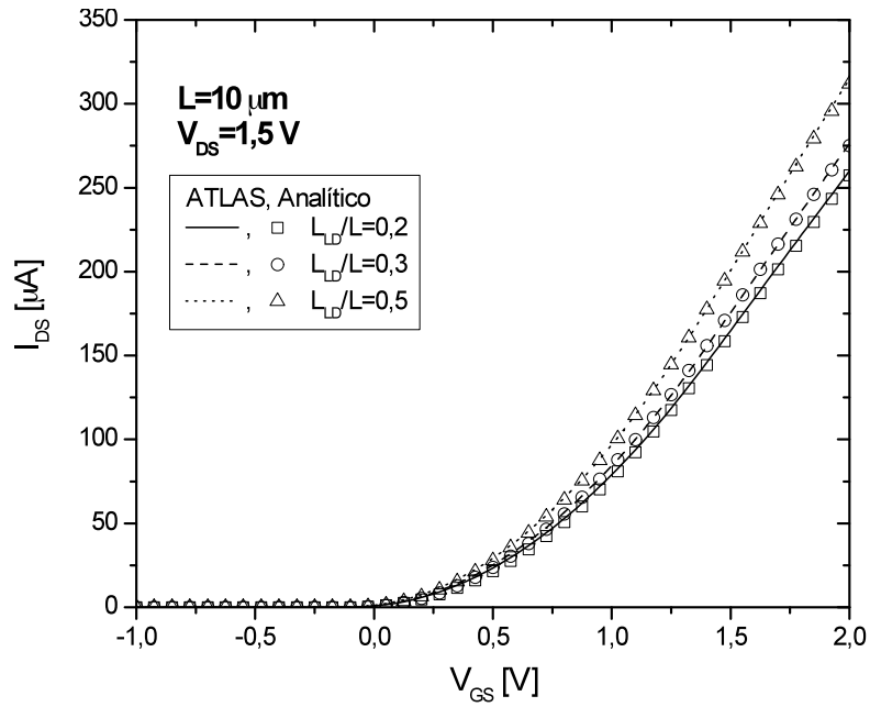
Figura 4.29 - Característica I_{DS} \times V_{GS} com V_{DS}=1,5 V, para L = 10 \mu\text{m} .
