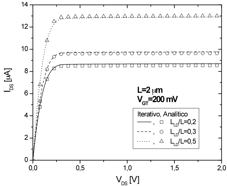
Figura 4.19 - Característica I_{DS} \times V_{DS} com sobretensão V_{GT}=200 \text{ mV} , para L = 2 \mu\text{m} .
