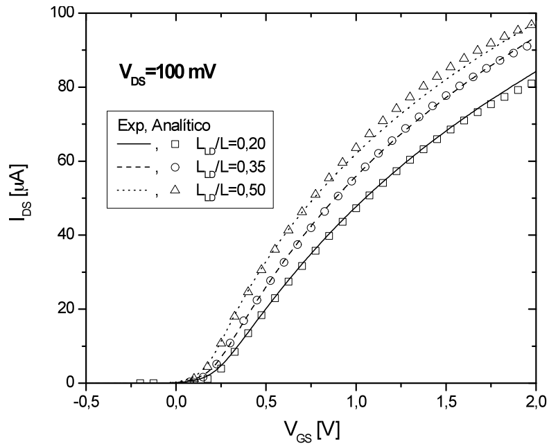
Figura 4.54 - Característica I_{DS} \times V_{GS} com V_{DS}=100 mV.
