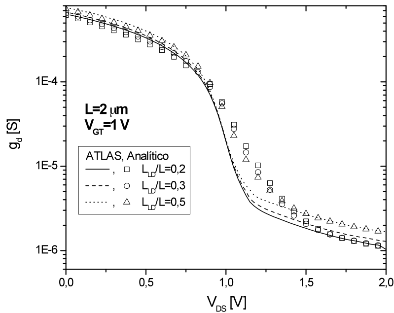
Figura 4.52 - Condutância g_d \times V_{DS} com V_{GT}=1 V, para L = 2 \mu\text{m} .
