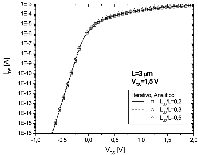
Figura 4.15 - Característica I_{DS} \times V_{GS} em sublimiar com V_{DS}=1,5 V, para L = 3 \mu\text{m} .
