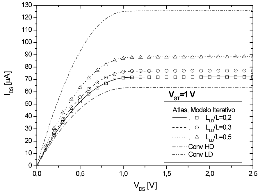
Figura 3.7 - Característica I_{DS} \times V_{DS} com sobretensão V_{GT}=1 V
