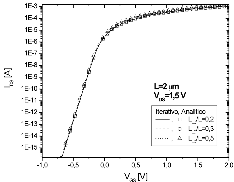
Figura 4.16 - Característica I_{DS} \times V_{GS} em sublimiar com V_{DS}=1,5 V, para L = 2 \mu\text{m} .
