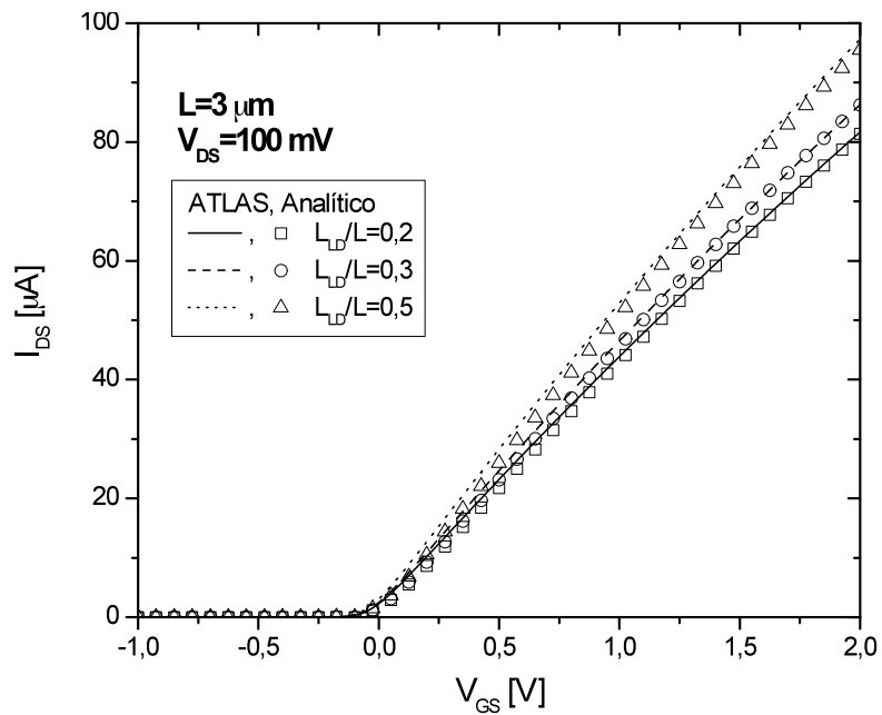
Figura 4.24 - Característica I_{DS} \times V_{GS} com V_{DS}=100 mV, para L = 3 \mu\text{m} .
