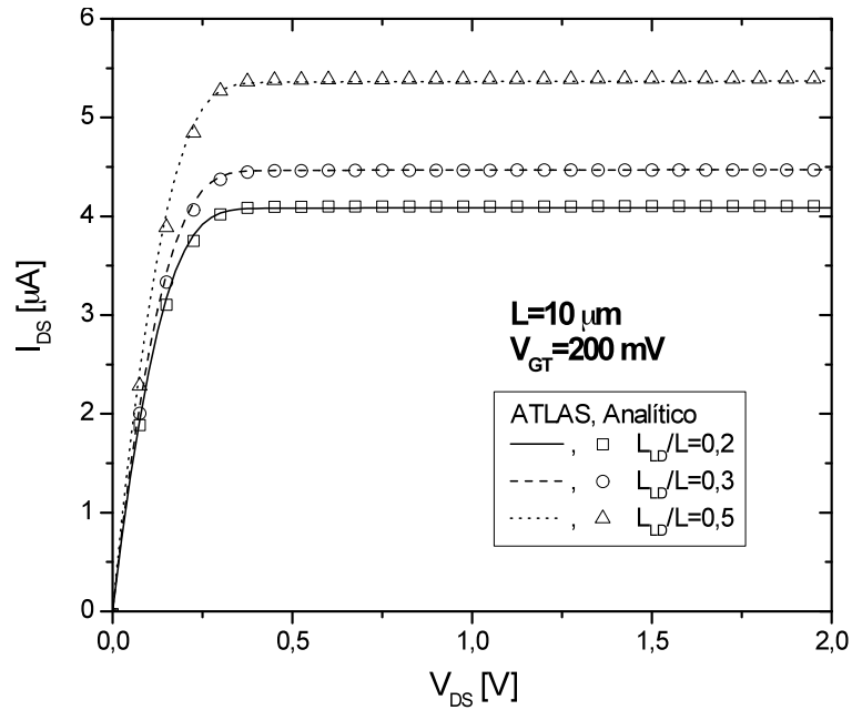
Figura 4.41 - Característica I_{DS} \times V_{DS} com sobretensão V_{GT}=200 mV, para L = 10 \mu\text{m} .
