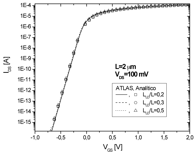
Figura 4.28 - Característica I_{DS} \times V_{GS} em sublimiar com V_{DS}=100 mV, para L = 2 \mu\text{m} .
