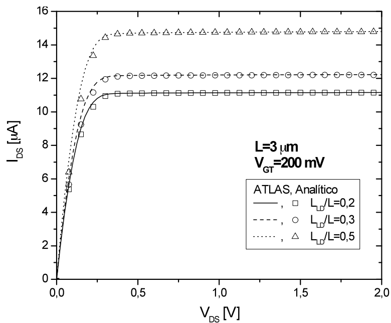
Figura 4.42 - Característica I_{DS} \times V_{DS} com sobretensão V_{GT}=200 mV, para L = 3 \mu\text{m} .
