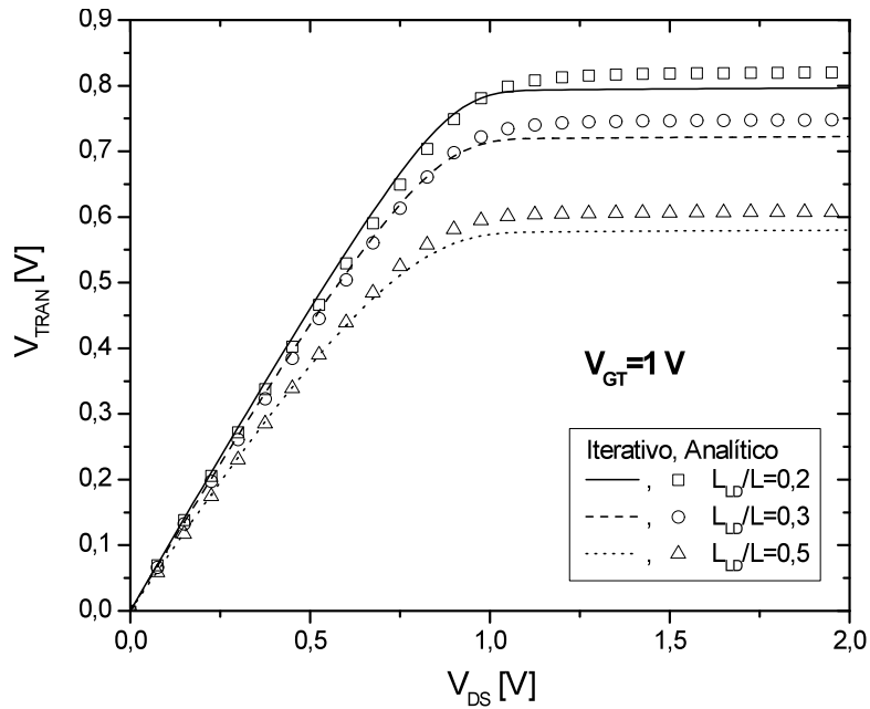
Figura 4.4 - Tensão de transição pela tensão de dreno com V_{GT}=1 V.
