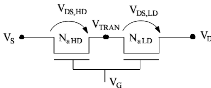
Figura 3.1 - Circuito equivalente ao transistor GC GAA
