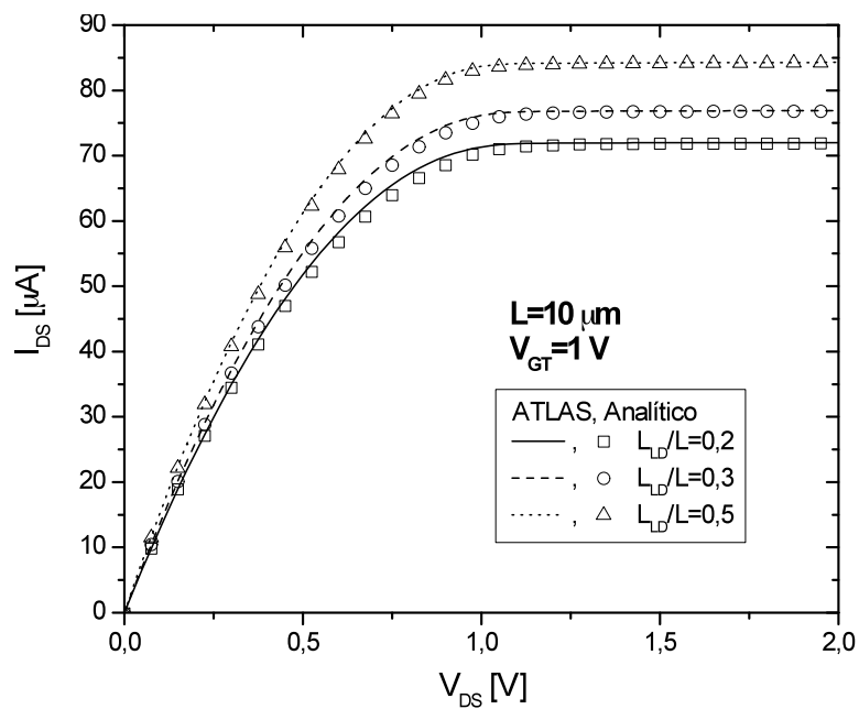
Figura 4.44 - Característica I_{DS} \times V_{DS} com sobretensão V_{GT}=1\ \text{V} , para L = 10\ \mu\text{m} .
