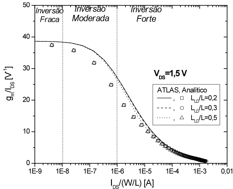
Figura 4.53 - Relação g_m/I_{DS} pela corrente de dreno normalizada para transistores GC GAA.
