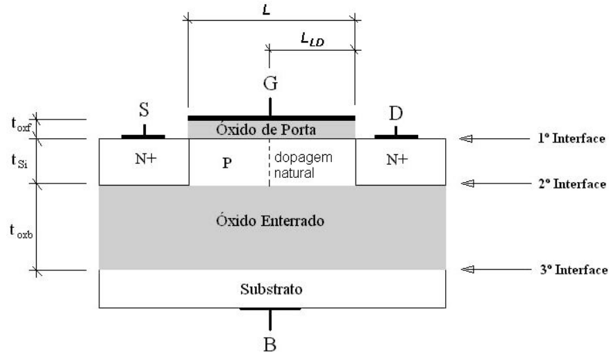
Figura 2.5 - Perfil do transistor SOI MOSFET canal n totalmente depletado com perfil de dopantes assimétrico na região de canal (GC SOI nMOSFET).
