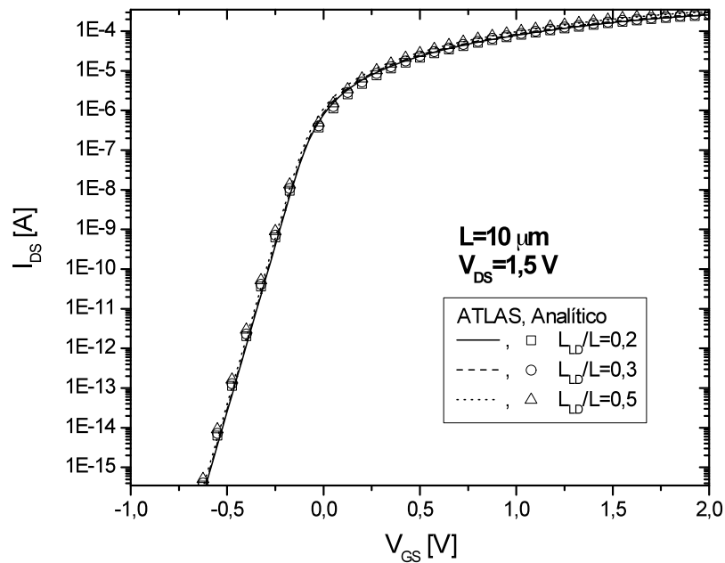
Figura 4.32 - Característica I_{DS} \times V_{GS} em sublimiar com V_{DS}=1,5 V, para L = 10 \mu\text{m} .
