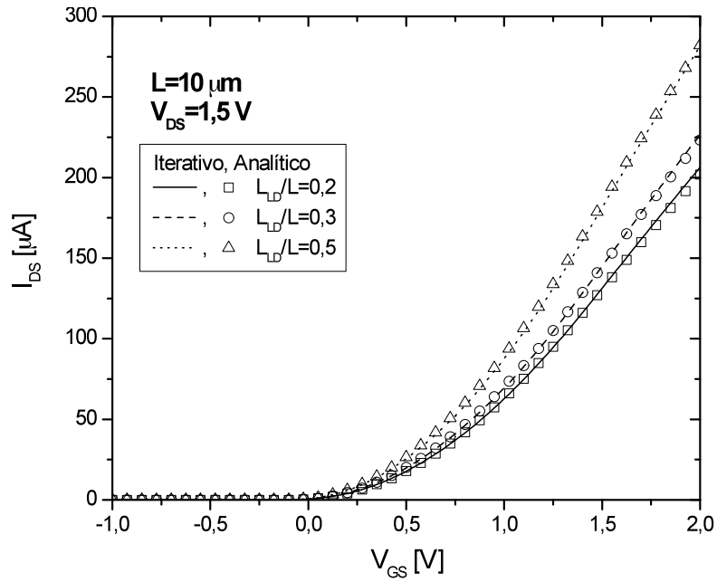
Figura 4.11 - Característica I_{DS} \times V_{GS} com V_{DS}=1,5 V, para L = 10 \mu\text{m} .
