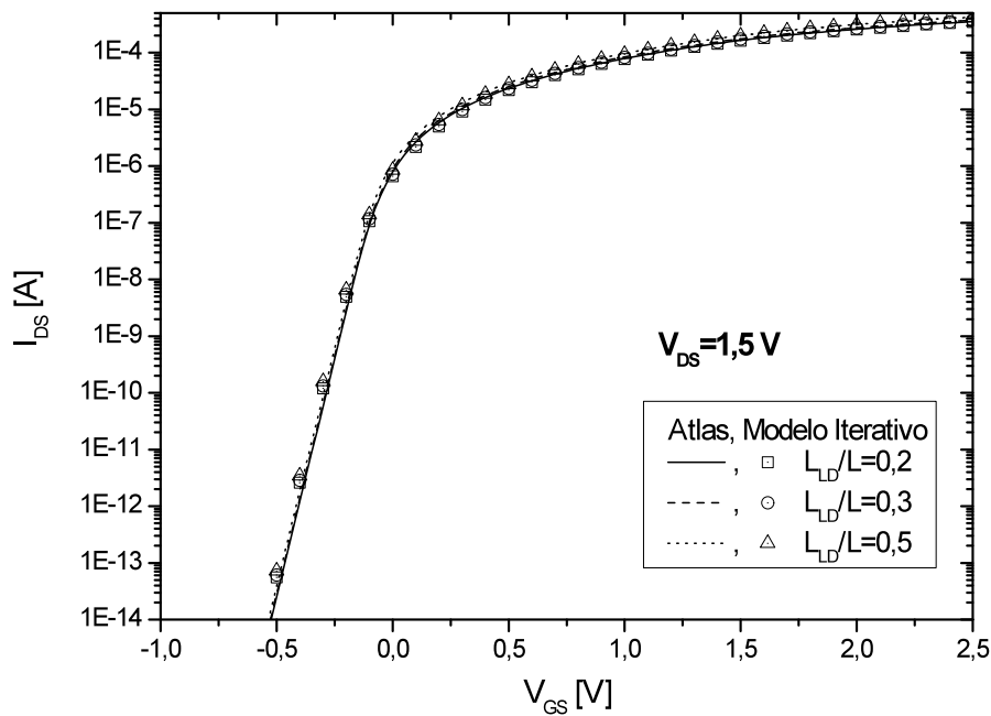
Figura 3.5 - Característica I_{DS} \times V_{GS} em sublimiar com V_{DS} = 1,5 \text{ V}
