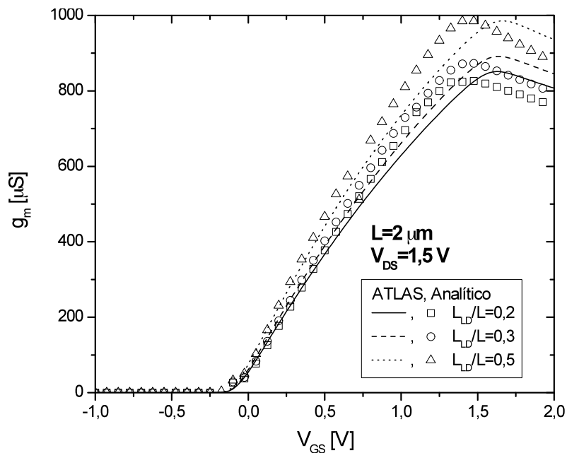
Figura 4.40 - Transcondutância g_m \times V_{GS} com V_{DS}=1,5 V, para L = 2 \mu\text{m} .
