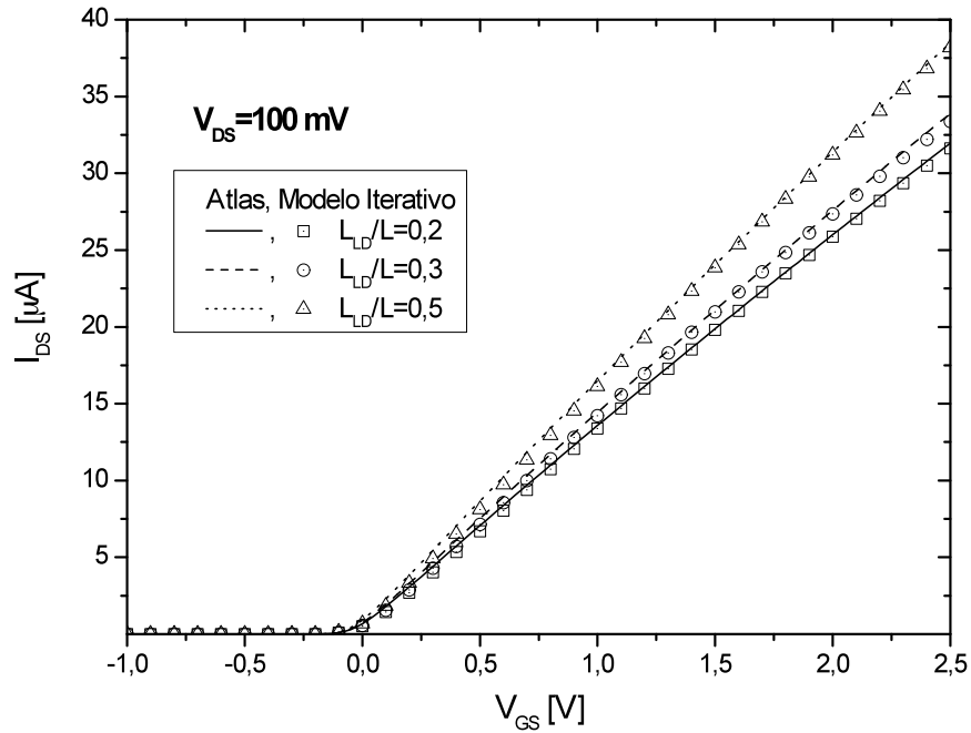
Figura 3.2 - Característica I_{DS} \times V_{GS} com V_{DS}=100 mV
