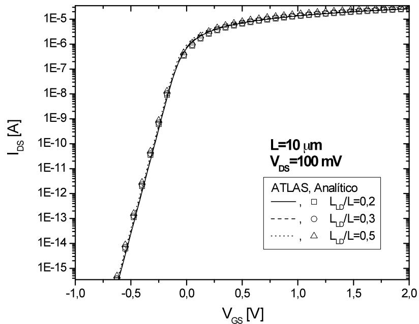
Figura 4.26 - Característica I_{DS} \times V_{GS} em sublimiar com V_{DS} = 100 \text{ mV} , para L = 10 \mu\text{m} .
