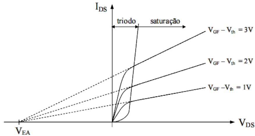
Figura 2.9 - Determinação da tensão Early através da extrapolação da curva I_{DS} \times V_{DS} .
