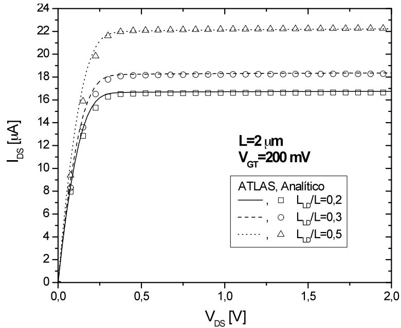
Figura 4.43 - Característica I_{DS} \times V_{DS} com sobretensão V_{GT}=200\ \text{mV} , para L = 2\ \mu\text{m} .
