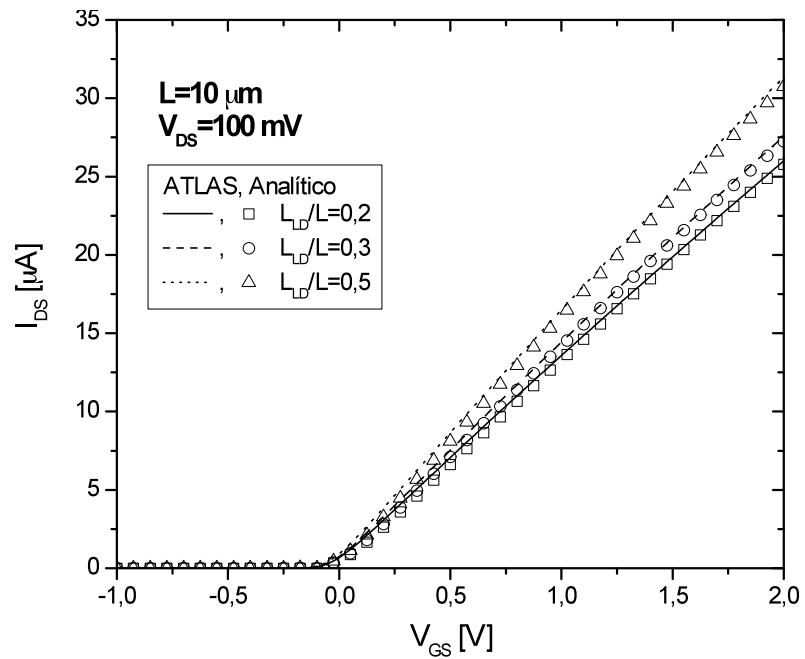
Figura 4.23 - Característica I_{DS} \times V_{GS} com V_{DS}=100 mV, para L = 10 \mu\text{m} .
