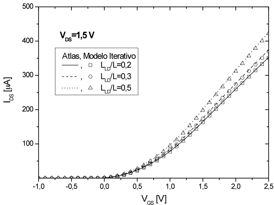
Figura 3.3 - Característica I_{DS} \times V_{GS} com V_{DS}=1,5 V
