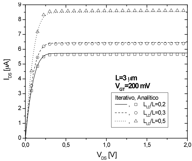
Figura 4.18 - Característica I_{DS} \times V_{DS} com sobretensão V_{GT}=200 \text{ mV} , para L = 3 \mu\text{m} .
