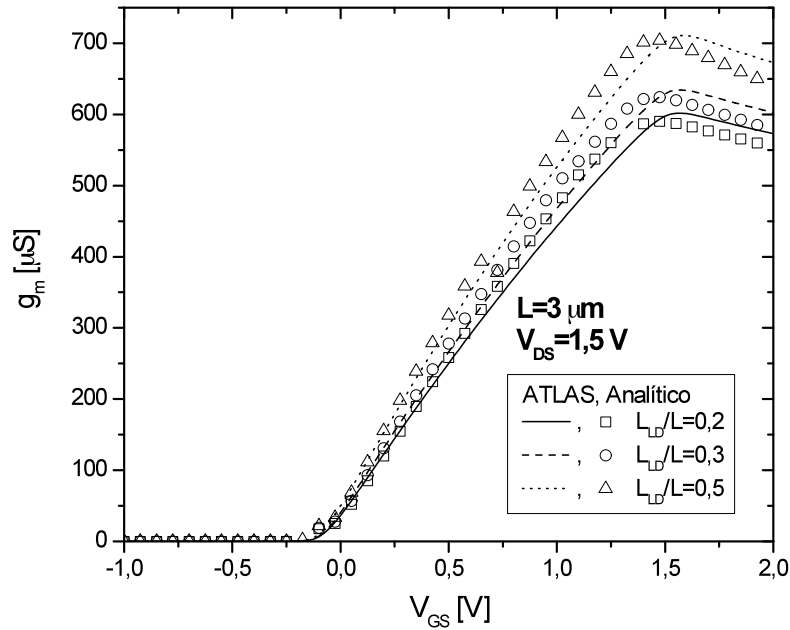
Figura 4.39 - Transcondutância g_m \times V_{GS} com V_{DS}=1,5 V, para L = 3 \mu\text{m} .
