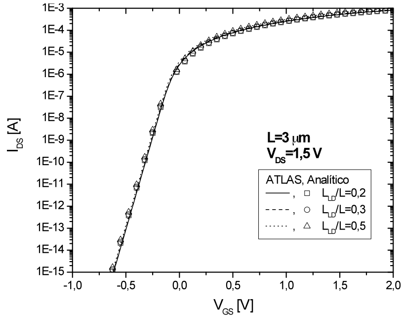
Figura 4.33 - Característica I_{DS} \times V_{GS} em sublimar com V_{DS}=1,5 V, para L = 3 \mu\text{m} .
