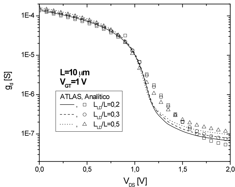
Figura 4.50 - Condutância g_d \times V_{DS} com V_{GT}=1 V, para L = 10 \mu\text{m} .
