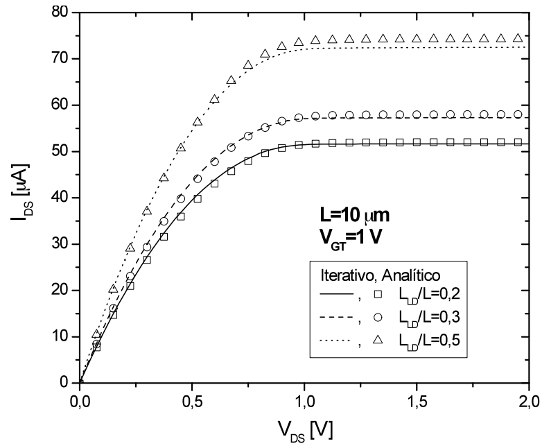
Figura 4.20 - Característica I_{DS} \times V_{DS} com sobretensão V_{GT}=1 V, para L = 10 \mu\text{m} .
