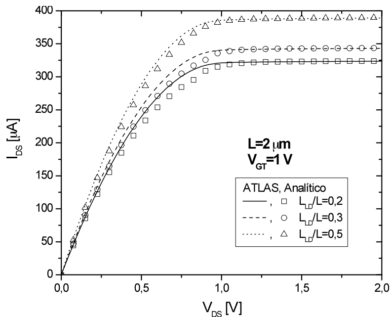
Figura 4.46 - Característica I_{DS} \times V_{DS} com sobre-tensão V_{GT}=1 V, para L = 2 \mu\text{m} .
