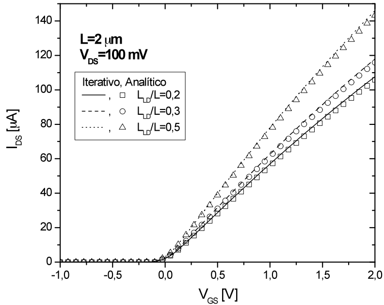
Figura 4.7 - Característica I_{DS} \times V_{GS} com V_{DS} = 100 \text{ mV} , para L = 2 \mu\text{m} .
