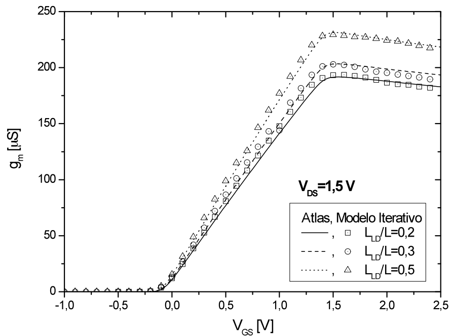
Figura 3.9 - Transcondutância g_m \times V_{GS} com V_{DS}=1,5 \text{ V}
