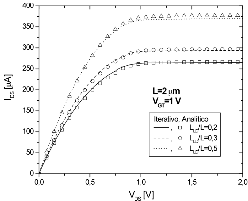
Figura 4.22 - Característica I_{DS} \times V_{DS} com sobretensão V_{GT}=1 V, para L = 2 \mu\text{m} .
