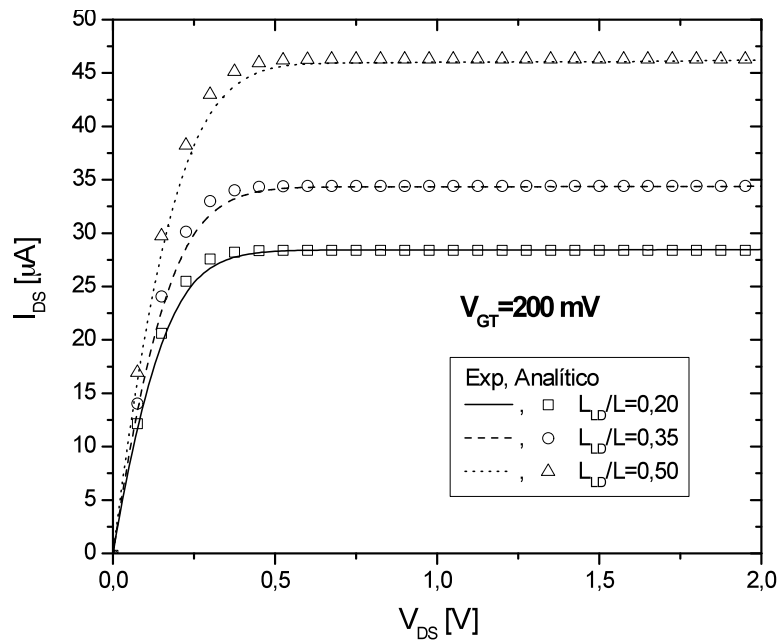
Figura 4.58 - Característica I_{DS} \times V_{DS} com sobretensão V_{GT}=200 mV.
