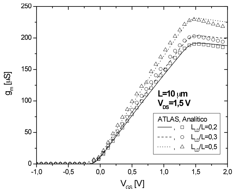
Figura 4.38 - Transcondutância g_m \times V_{GS} com V_{DS}=1,5 V, para L = 10 \mu\text{m} .
