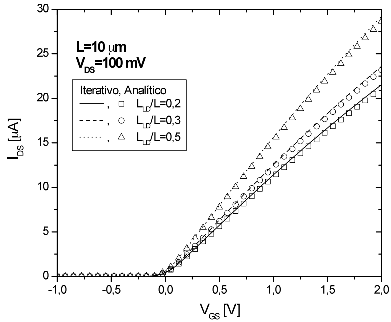
Figura 4.5 - Característica I DS xV GS com V DS =100 mV, para L = 10 \mu\text{m} .
