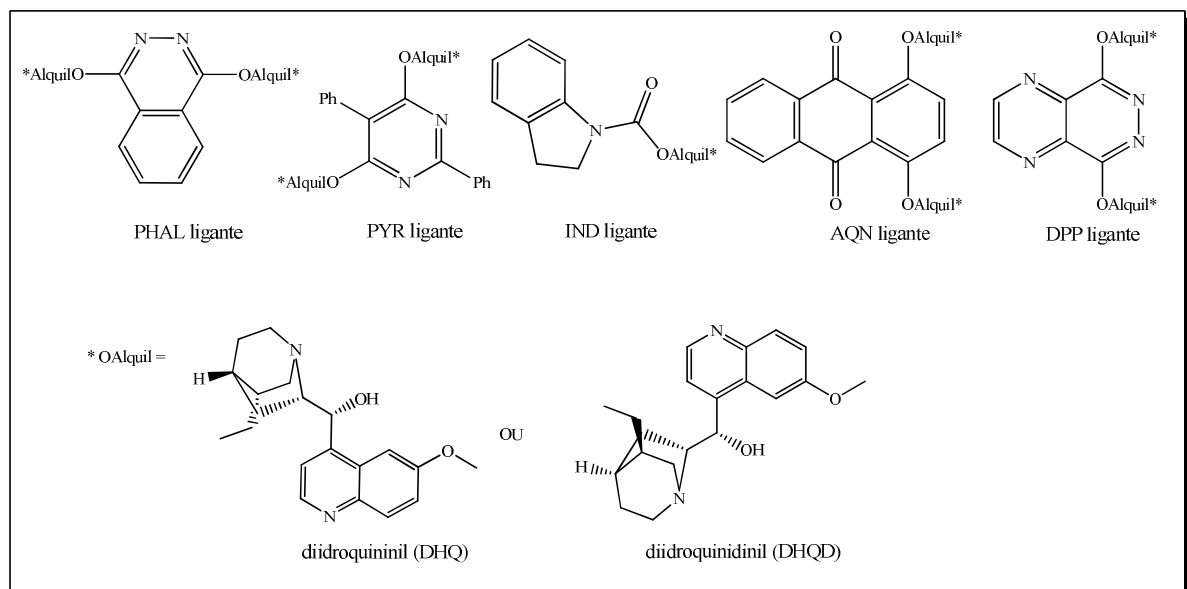
Figura 2.9. Ligantes derivados da Cinchona.
