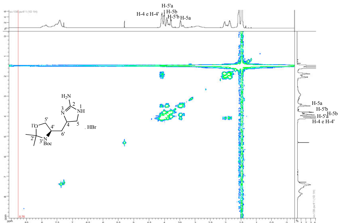
Figura 2.18. Mapa de contornos COSY de 141a em CDCl 3 (300MHz).
