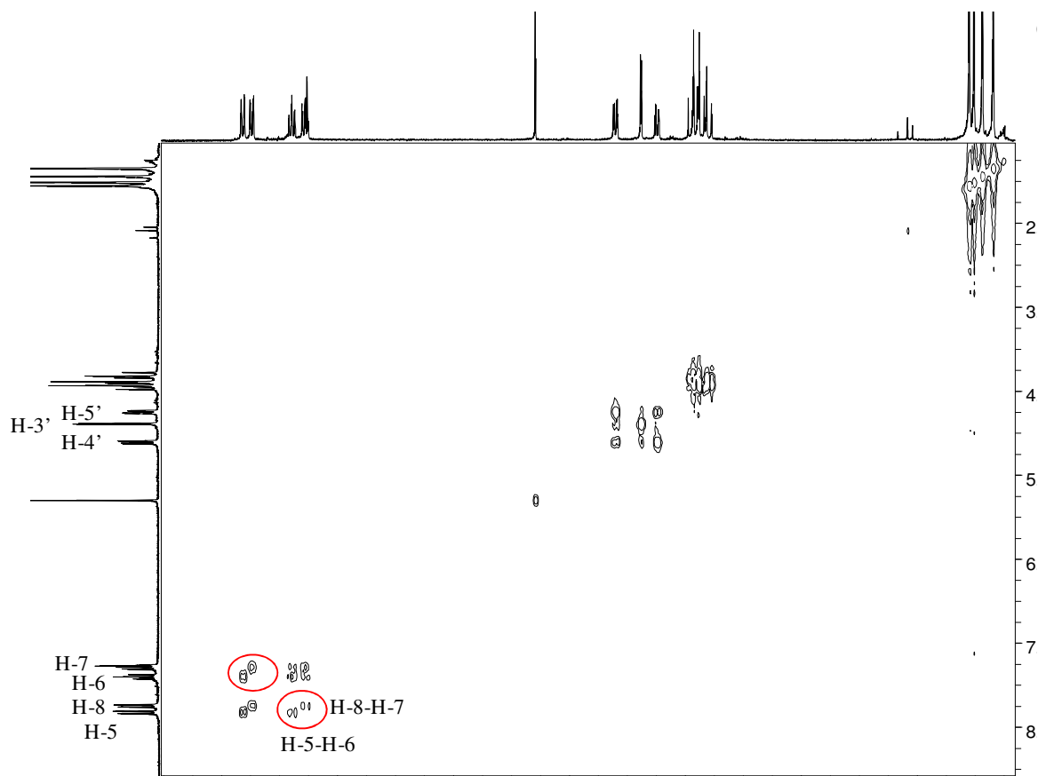
Figura 1.58. Mapa de contornos COSY de 17 em \text{CDCl}_3 (300MHz).
