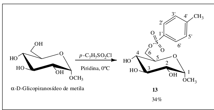
Esquema 1.17. Preparação do composto 13 .
