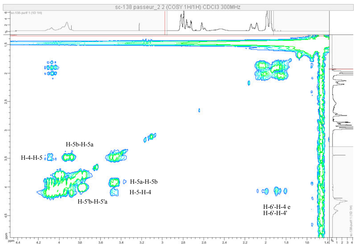
Figura 2.19. Expansão do COSY de 141a em CDCl 3 (300MHz).
