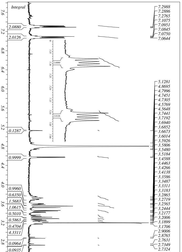
Figura 1.67. Espectro de RMN de 1 H de 20 em D 2 O (300MHz).
