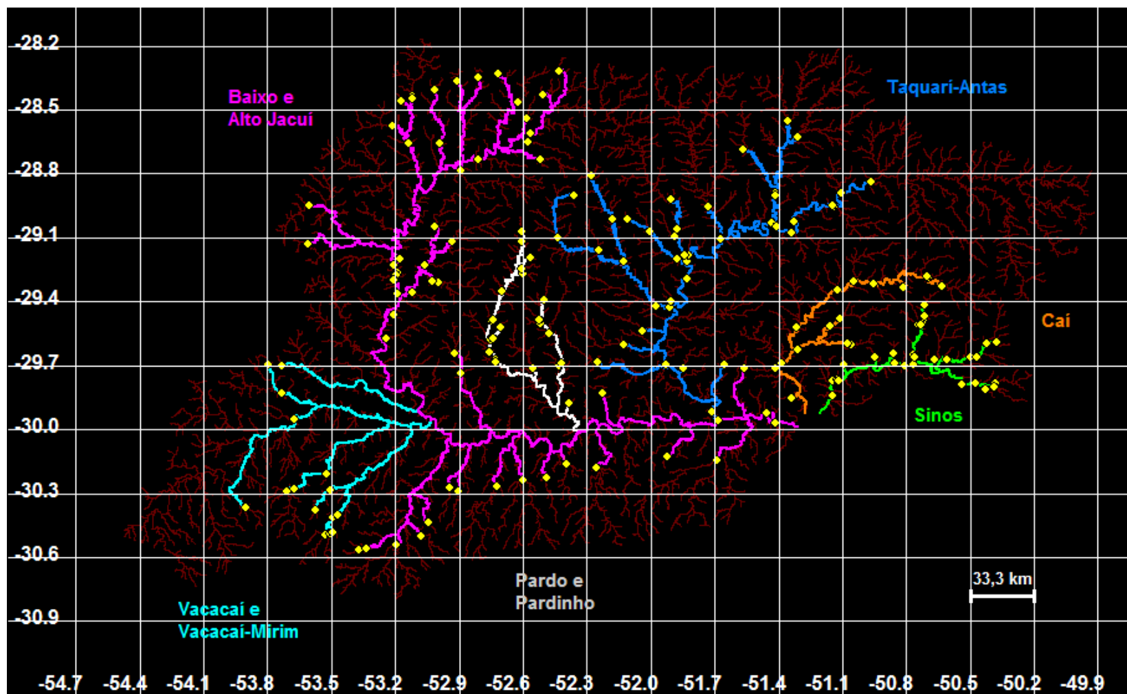
Figura 1. Hidrografia amostrada sobreposta à hidrografia total da bacia do Jacuí (em vermelho). Os 155 pontos em amarelo representam os locais de amostragem (mapa gerado a partir de modelo numérico de elevação em pixel de 92 por 92 m, segundo WEBER et al. , 2004).
