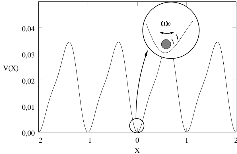
Fig. 3.9: Potencial adimensional V(X) descrito pela Eq. (3.17). A ampliação da região do mínimo, em X = 0 , ilustra a partícula oscilando em torno desse ponto com freqüência \omega_0 dada pela Eq. (3.14).
