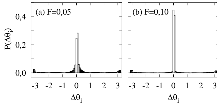
Fig. 6.12: Distribuição P(\Delta\theta_i) da diferença entre os ângulos dos subseqüentes passeios de Lévy para N = 60 , sendo (a) F = 0,05 e (b) F = 0,10 .
