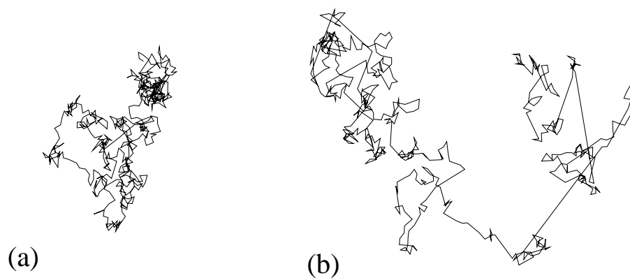
Fig. 2.2: Passeios aleatórios, após 500 passos, gerados artificialmente com a distribuição de probabilidade P(l) \sim l^{-\mu} , onde a direção de cada passo foi escolhida aleatoriamente [73]. O valor do expoente \mu foi escolhido apropriadamente: (a) \mu = 3,8 para difusão normal e (b) \mu = 2,2 para o caso super-difusivo (vôos de Lévy).
