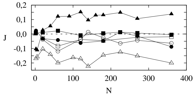
Fig. 6.2: Corrente J em função do número N de osciladores para diferentes valores da amplitude F da força externa: F = 0,05 (■, □), F = 0,1 (▲, △) e F = 0,5 (●, ○). Os símbolos cheios representam os resultados referentes à distribuição de freqüências de Debye baixa e os símbolos vazios à distribuição de freqüências de Debye alta .
