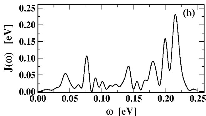
Fig. 3.3: Densidade espectral dos fônons que representam o banho térmico que interage com o sistema principal (que é constituído por 16 unidades moleculares de B850 BChls). Figura retirada da Ref. [82].
