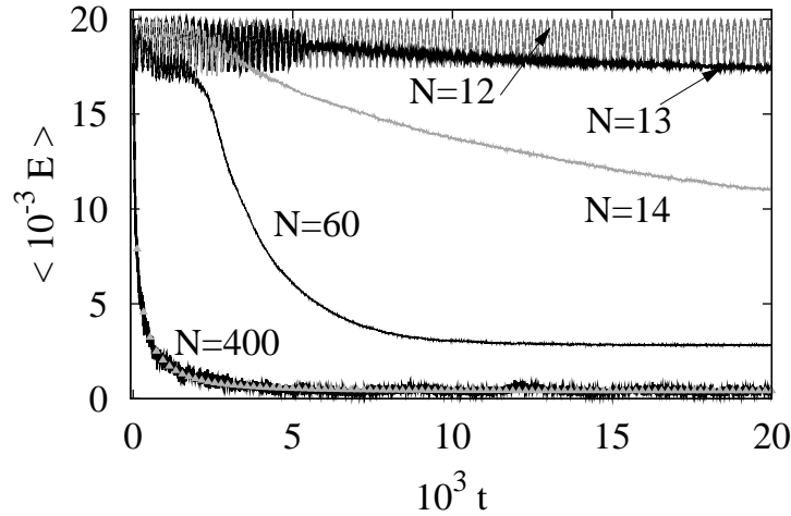
Fig. 5.1: Energia média da partícula em função do tempo, para N = 12, 13, 14, 60 e 400 . A média foi realizada sobre 800 condições iniciais dos osciladores do meio. Os símbolos ( \blacktriangle ), junto da curva N = 400 , representam o ajuste da curva que é dado pela expressão: A + B \exp(-\alpha t^\beta) ( stretched exponential ) com os valores A \sim 4 \times 10^{-4} , B \sim 0,027 , \alpha \sim 0,203 e \beta \sim 0,384 .
