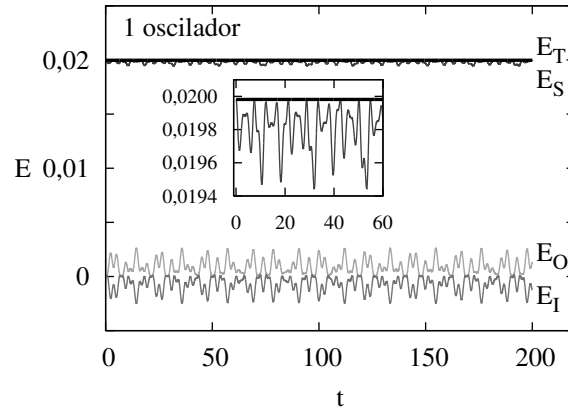
Fig. 4.1: Evolução temporal das energias individuais: E_T , E_S , E_O e E_I . A figura interna mostra os detalhes da evolução temporal para a energia da partícula no intervalo de tempo 0 \leq t \leq 60 .
