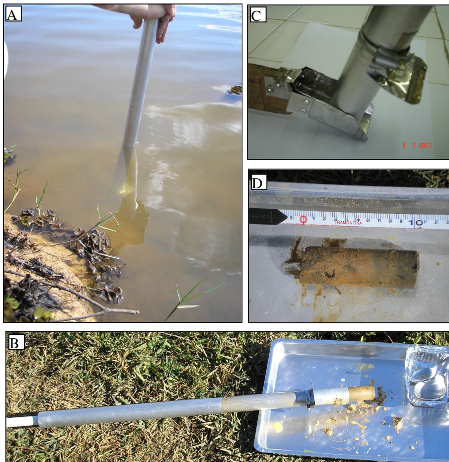
FIGURA 3.2: Detalhes do coletor desenvolvido e sua aplicação em campo. A - Inserção do tubo no sedimento; B - Extrusão do sedimento; C - posição de encaixe da pá sustentação; D - aspecto de uma amostra após a retirada do tubo.
