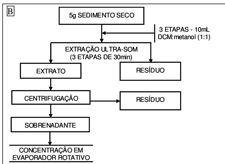
FIGURA 3.5: Fluxograma representando a otimização da extração das amostras. A – extração por ultra-som com uso do cadinho de Gooch e B – Extração por ultra-som seguido de centrifugação do extrato.
