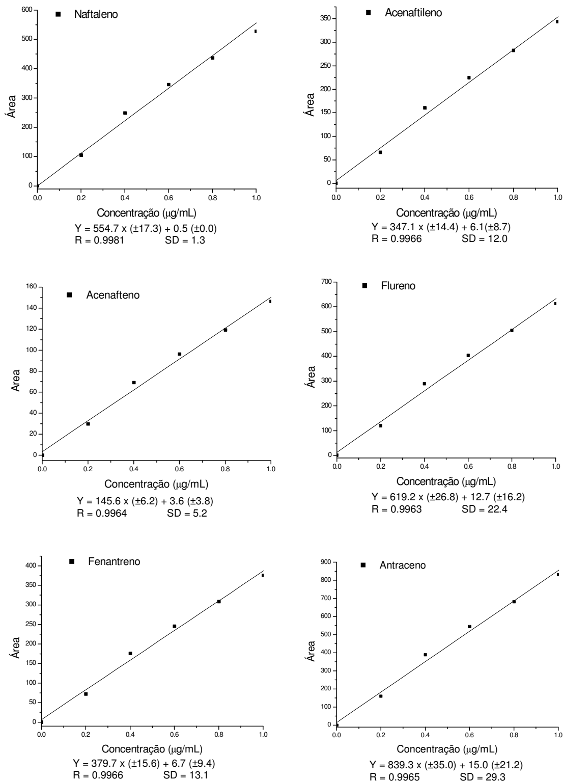
FIGURA 4.11-A: Curvas analíticas obtidas na condição otimizada para Naph, Acen, Ace, Flu, Phe e Ant. Todas as curvas foram preparadas em triplicata nas concentrações de 0,00 \mu\text{g}\cdot\text{mL}^{-1} ; 0,20 \mu\text{g}\cdot\text{mL}^{-1} ; 0,40 \mu\text{g}\cdot\text{mL}^{-1} ; 0,60 \mu\text{g}\cdot\text{mL}^{-1} ; 0,80 \mu\text{g}\cdot\text{mL}^{-1} e 1,00 \mu\text{g}\cdot\text{mL}^{-1} do Mix 16 HPA., sendo o primeiro ponto da curva o solvente empregado na diluição dos padrões.
