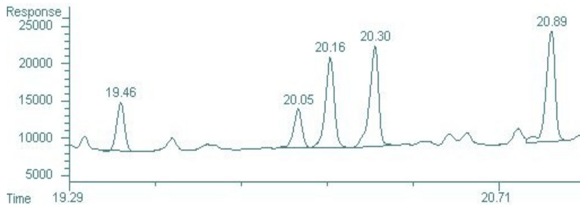
Figura 82: Detalhe do cromatograma do óleo de "andirola" no método estabelecido em coluna HP-5ht.
