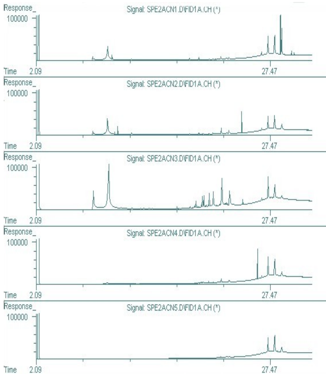
Figura 32: Cromatogramas das frações MeCN do experimento 2.
