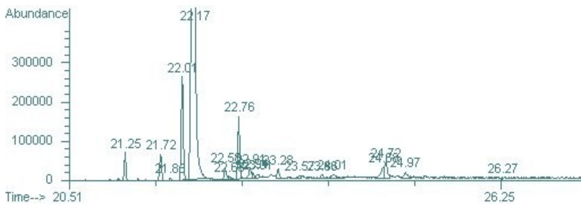
Figura 22: Cromatograma da etapa de obtenção de 7-oxo do experimento 8 com detalhe
