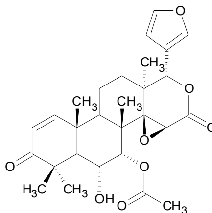
6 \alpha -hidroxigedunina
