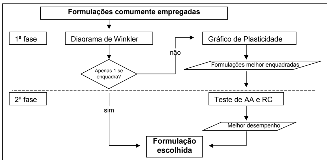
Figura 5.9 - Esquema para a escolha da formulação para fabricação dos tijolos com lodo.
