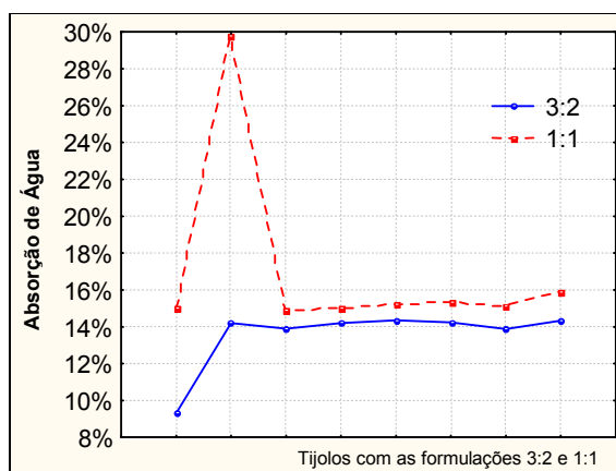
Gráfico 6.9 – Variação de Absorção de Água dos tijolos fabricados com as formulações de melhor desempenho.
