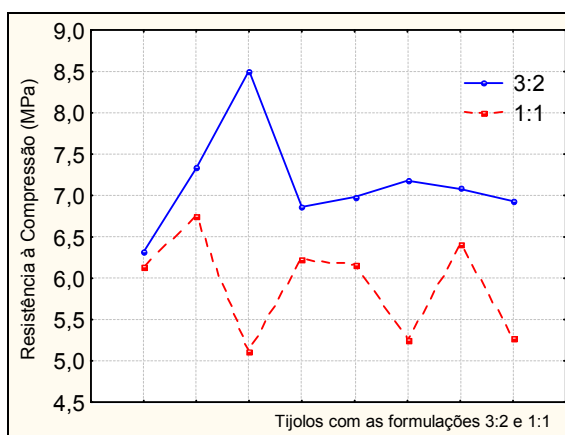
Gráfico 6.10 – Variação de Resistência à Compressão dos tijolos fabricados com as formulações de melhor desempenho.
