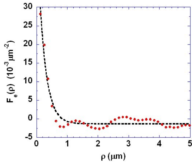
Figura 5.3: Comportamento típico da função de autocorrelação espacial F_e(\rho) . O comprimento de correlação \xi e a curvatura rms \kappa médios para as FAC são determinados ajustando-se a curva obtida pela Equação 5.2 . Para este gráfico, \xi = 0,23 \mu\text{m} , \kappa = 0,23 \mu\text{m}^{-1} e B_0 = -1 \times 10^{-3} \mu\text{m}^{-2} .
