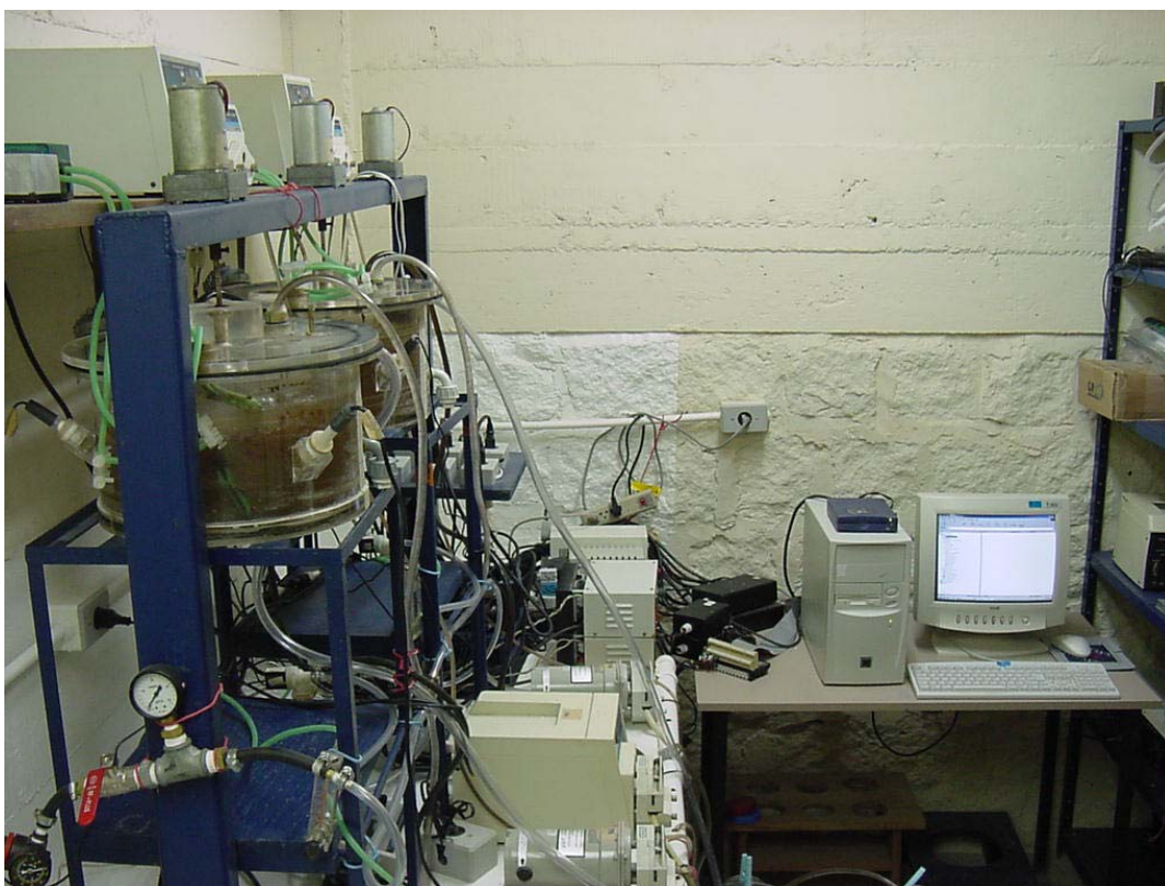
Figura 4.3 - Sistema de automação e reatores seqüenciais em batelada.
