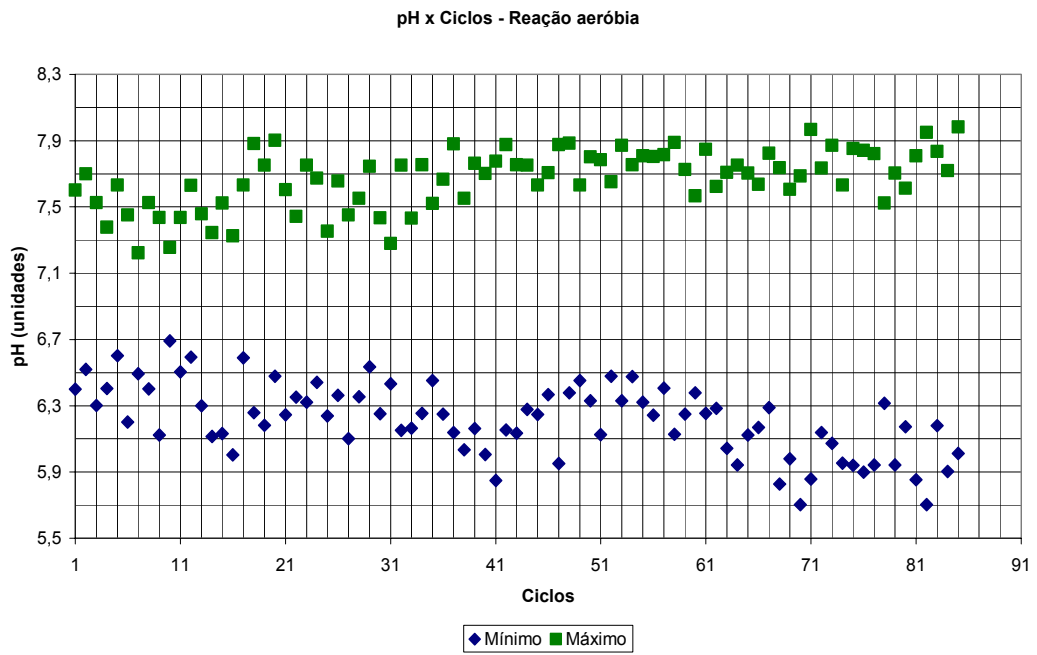
Figura 5.22 - Faixa do pH durante a reação aeróbia.
