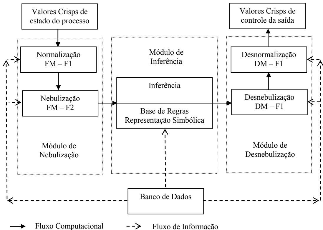
Figura 3.32 - Arquitetura do controle difuso.
