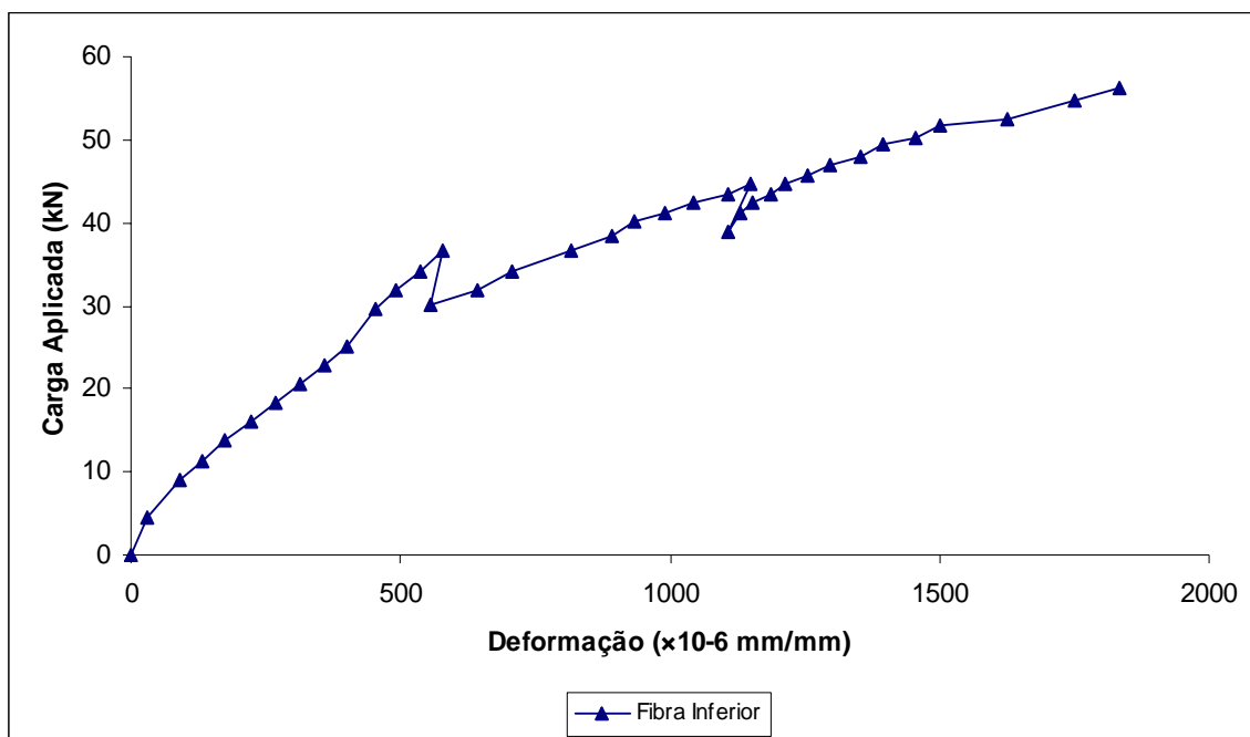
Figura B.41 - Relação carga \times deformação no “steel-deck” - Série E - Protótipo 10
