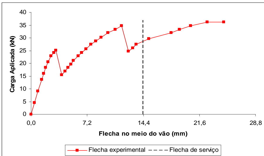
Figura B.15 - Relação carga × flecha no meio do vão - Série H - Protótipo 15
