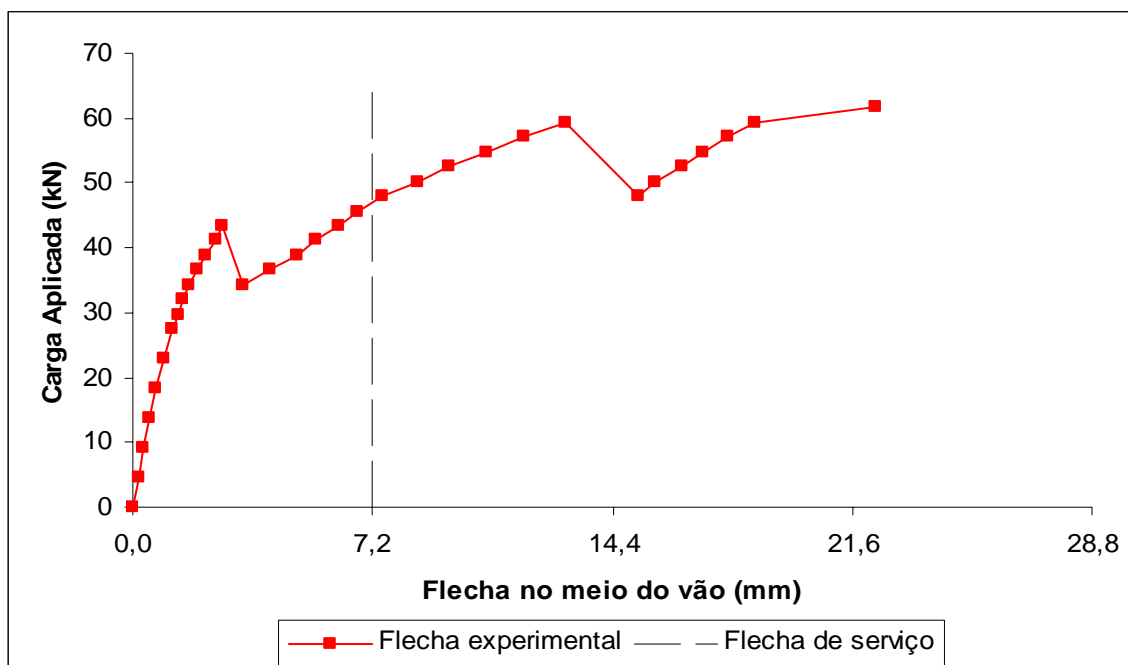
Figura 5.6 - Curva carga × flecha no meio do vão do protótipo da série G
