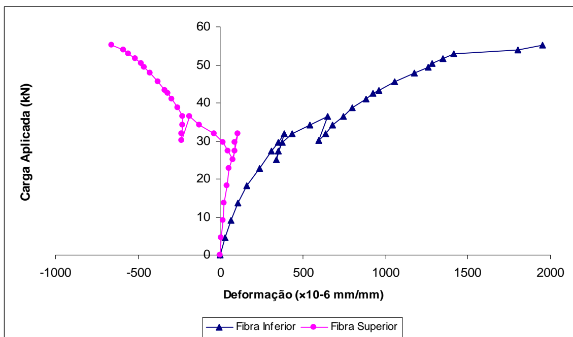
Figura B.42 - Relação carga \times deformação no “steel-deck” - Série E - Protótipo 11
