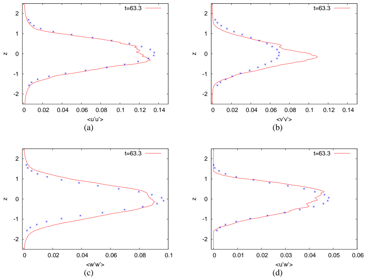
Figura 7.12: Comparação das tensões de Reynolds calculadas com as medidas experimentais (×, em azul) em regime de auto-similaridade de Bell & Mehta, 1990 [4]. Simulação FS F4VRi0 . (a) \langle u'u' \rangle ; (b) \langle v'v' \rangle ; (c) \langle w'w' \rangle ; (d) \langle u'w' \rangle ;
