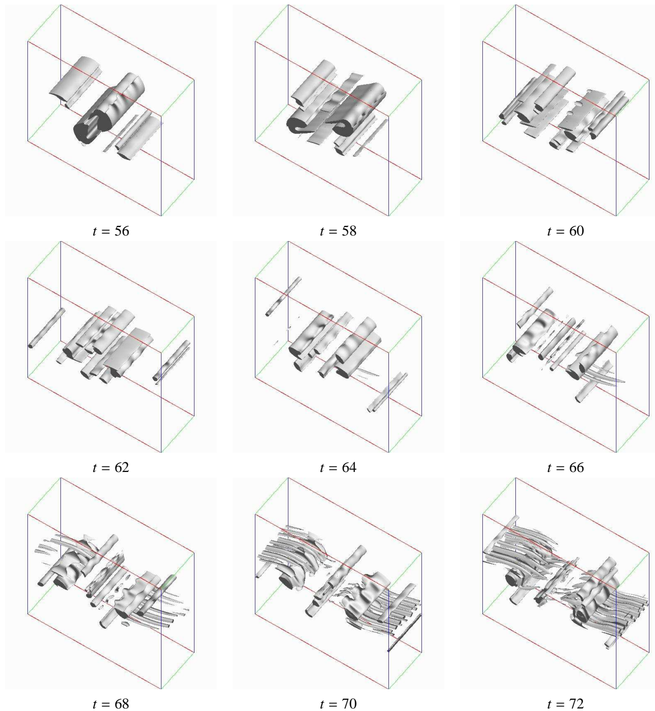
Figura 5.23: Isosuperfícies de Q = 0.2 . Simulação 3DF, Re = 500 , Ri = 0.167 .
