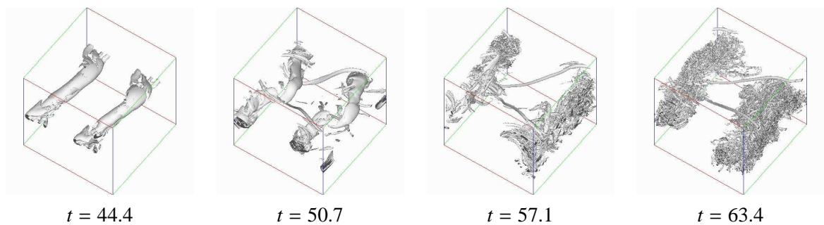
Figura 7.3: Isosuperfícies do critério Q. Simulação F S F 192 Ri 005 para Ri = 0.05 e Re = 2000 .
