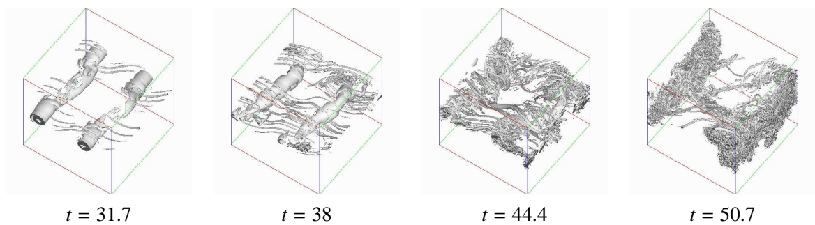
Figura 7.2: Isosuperfícies do critério Q. Simulação F S F 192 Ri 0 , para Ri = 0 e Re = 2000 .
