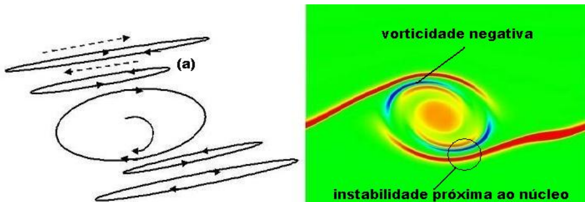
Figura 5.1: Representação esquemática da instabilidade próxima ao núcleo.
