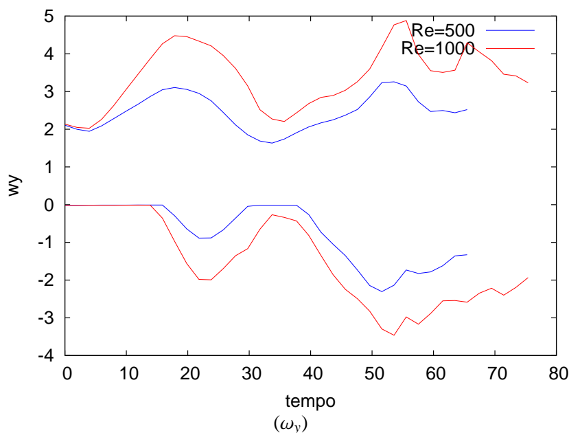
Figura 5.15: Evolução no tempo da vorticidade máxima e mínima ( \omega_y ). Simulação 2DFV_{II} , Re = 500 e simulação 2DFV , Re = 1000 , Ri = 0.167 .
