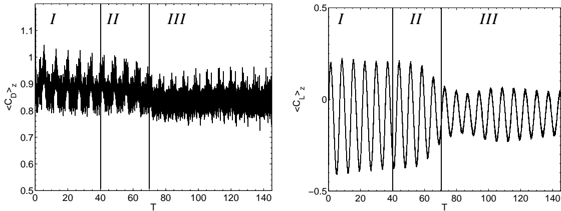
Figura 7.13: Serie temporal dos coeficientes de (a) arrasto e (b) sustentação, para Re_D = 300 e G = 0, 8 .
