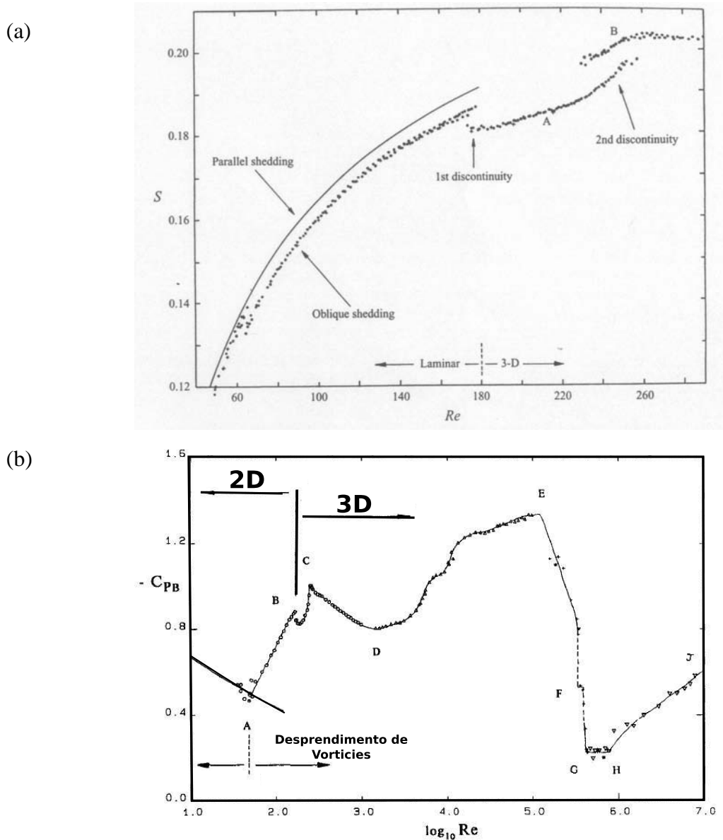
Figura 2.1: Variação: a) do número de Strouhal e b) do coeficiente de pressão de base em função do número de Reynolds ( Re_D ) (WILLIAMSON, 1996b).
