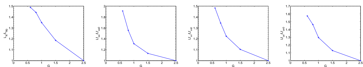
Figura 5.15: Comportamento do comprimento de formação ou recirculação em função do cisalhamento e/ou razão de afastamento.
