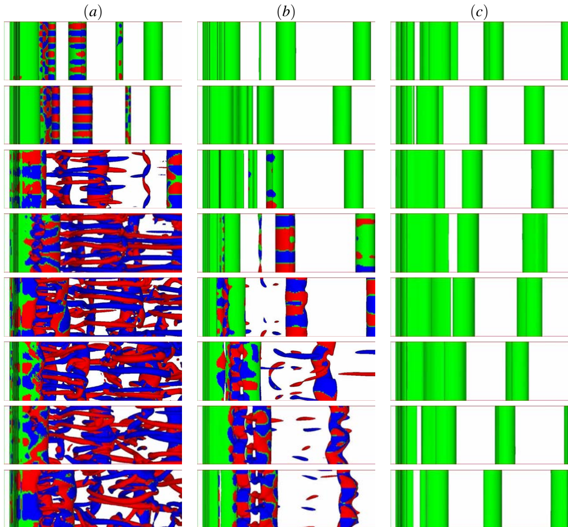
Figura 7.8: Visualização do campo instantâneo do critério Q em diferentes instantes para (a) G = 2,5 , (b) 0,8 e (c) 0,5 . (Vista superior da isosuperfície de Q = 0,1 , variação temporal de cima para baixo - T = 10, 15, 30, 45, 60, 90, 120 e 142 ).
